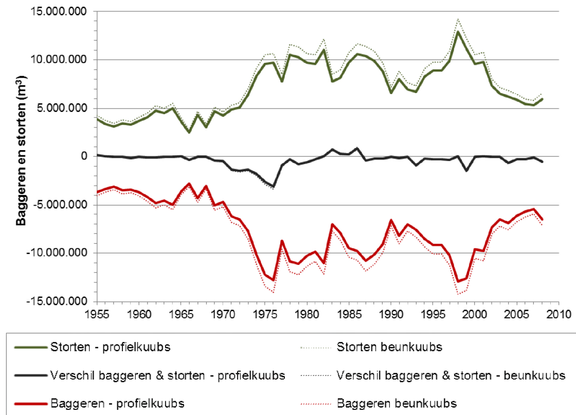
Figuur 6.6: Bagger en stortvolumes en het verschil voor de gehele Westerschelde in de periode 1955-2008
