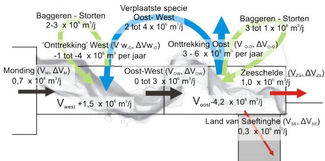
Figuur 10.3: Schematische weergave van de sedimentstromen in en rond de Westerschelde in drie perioden.
