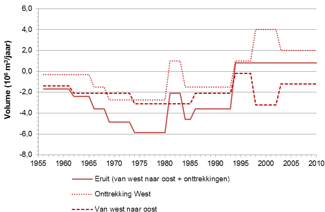
Figuur 8.6: Grafiek van de jaar op jaar sedimentvolumes uit de westelijke helft (eruit) en de twee bijdragende factoren daarin: de sedimentonttrekkingen en het berekende transport vanuit het westen naar het oosten.
