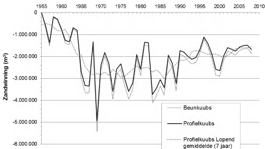
Figuur 6.8: Zandwinvolumes voor de gehele Westerschelde in de periode 1955-2008.
