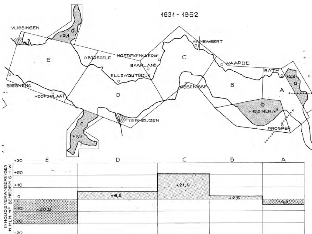
Figuur 2.2: Volumeveranderingen 1931-1952 volgens Bakker en De Looft (1977)
