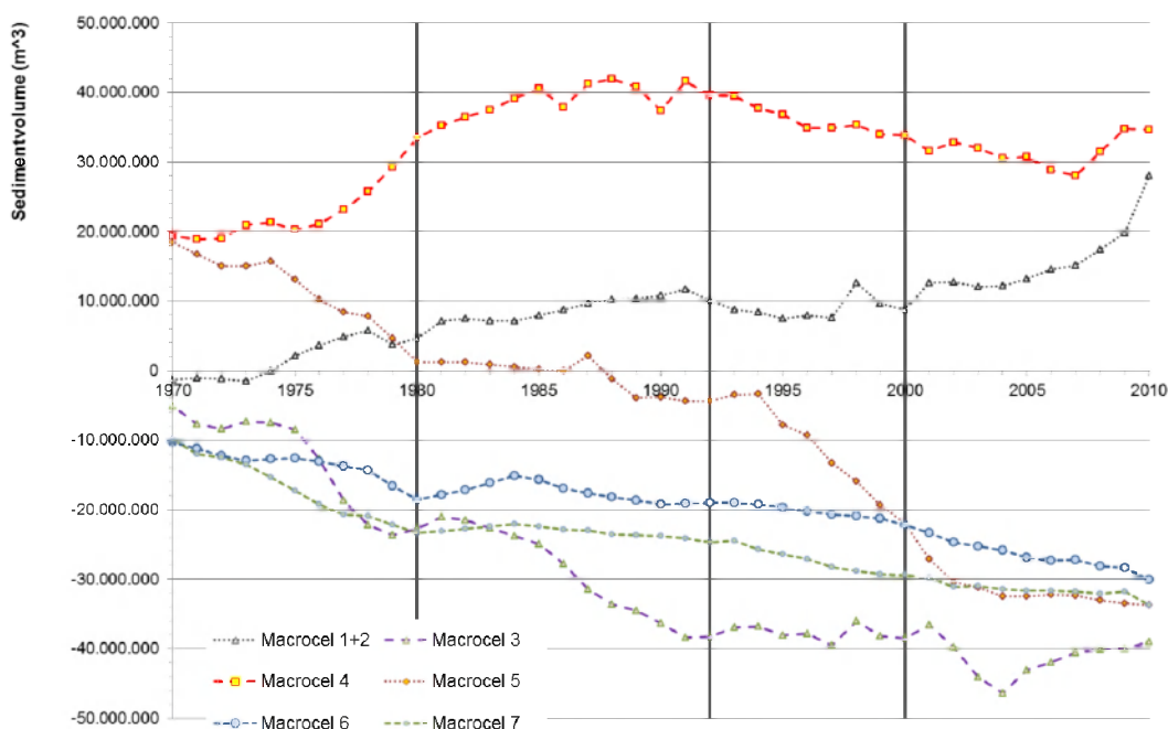
Figuur 4.1 Grafiek met de ontwikkeling van het sedimentvolume per macrocel voor de periode 1970-2010 (bron Rijkswaterstaat Zandbalans).
