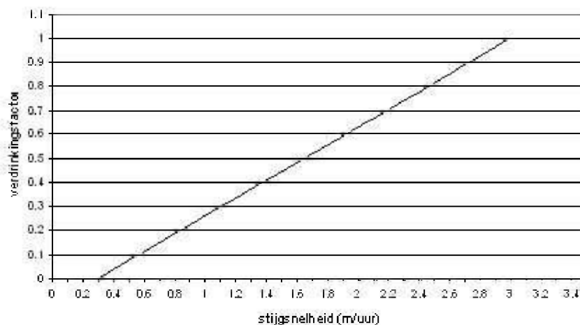
Figuur 5.7 Verdrinkingsfactor als functie van de stijgsnelheid.
