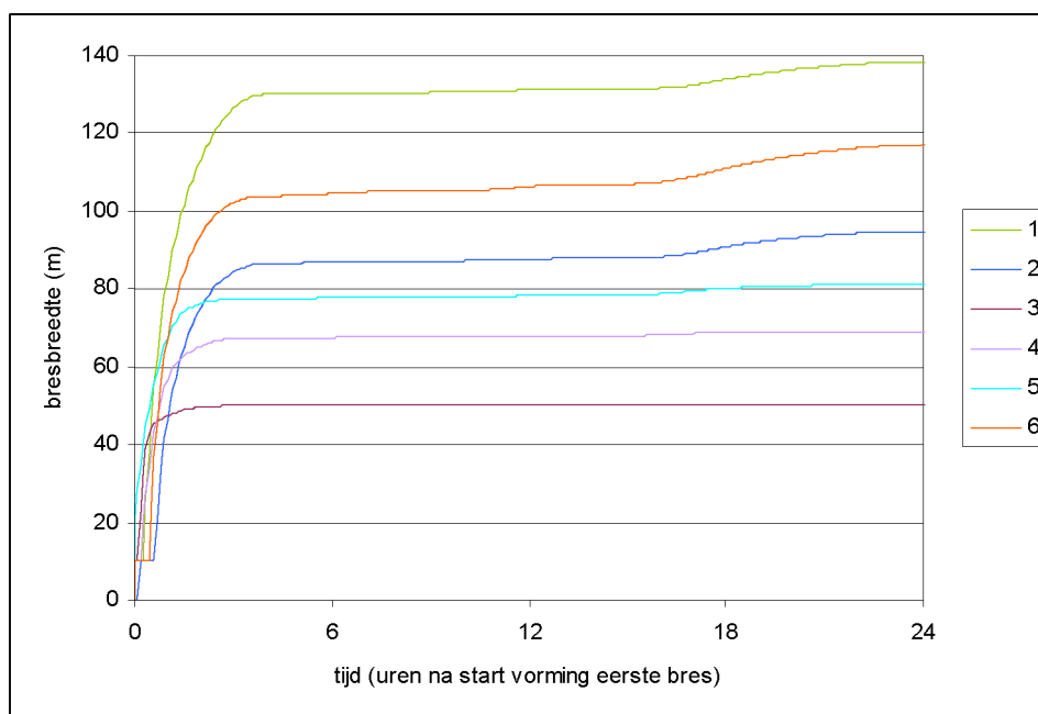
Figuur 4.14 Bresgroei gesimuleerd met SOBEK voor een stormvloed met een kans van voorkomen van 1:10.000 per jaar uitgaande van een zanddijk
