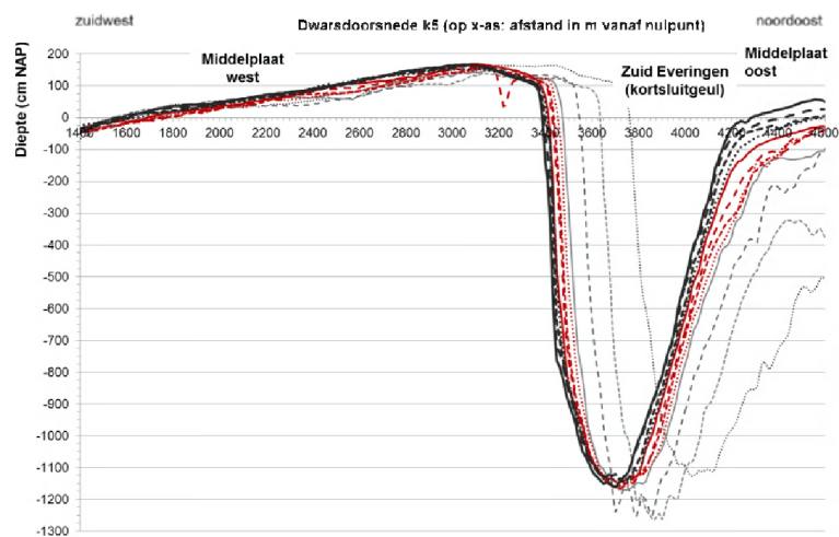
Figuur 11.3 Dwarsdoorsnede K5 (locatie in figuur 11.4).
