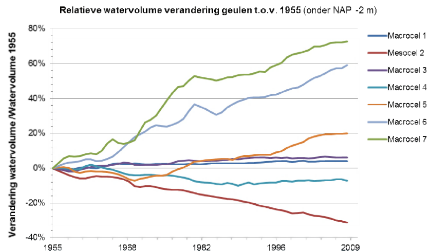
Figuur 7.10 Relatieve verandering van het watervolume van de geulen (onder NAP -2 m, op basis van de Zandbalans Rijkswaterstaat).
