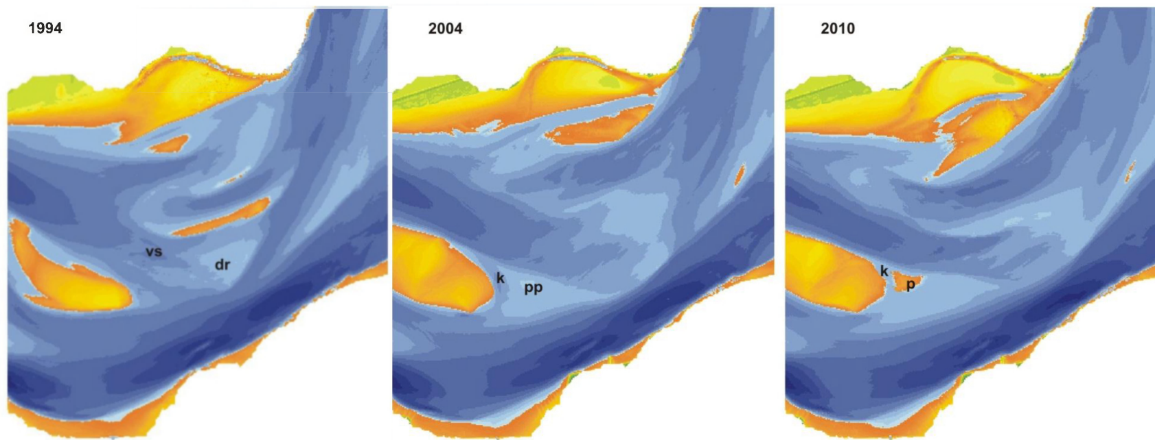
Figuur 12.3 Voorbeeld van de ontwikkeling van een plaat (p) en tijdelijke kortsluitgeul (k), uit een vloedschaar (vs) en drempel (dr), met een "protoplaat" (pp) bij de oostzijde van de Middelpaas.
