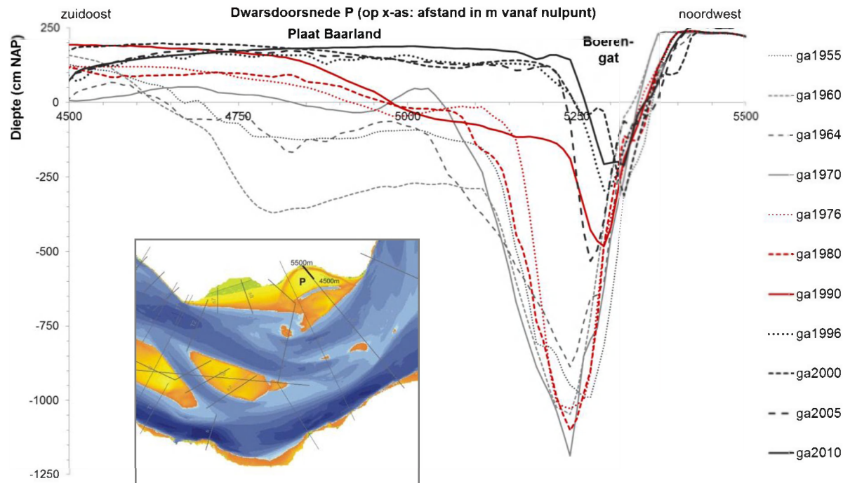
Figuur 13.2 Dwarsdoorsnede P door de Plaat van Baarland en het Boerengat (locatie in inzet).
