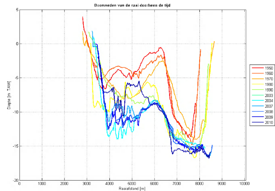
Figuur 7.3 Variatie in bodemligging over raai 1 in de Zeeschelde ( van linker- naar rechtoever, locatie van de raai in figuur 7.4) (uit: LTV V&T-rapport K-19).
