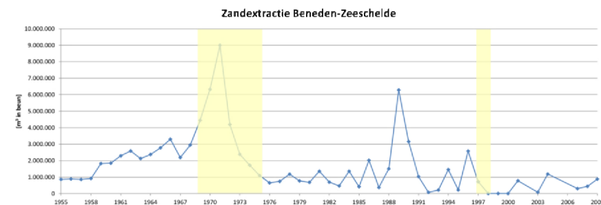
Figuur 7.11 Volume zand dat uit het systeem van de Beneden-Zeeschelde gehaald werd [ \text{m}^3 in beun]. De verdiepingsperiodes in geel (LTV V&T-rapport K-19).
