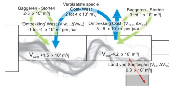
Figuur 7.13 Schematische weergave van de ingrepen in de Westerschelde in drie periode (naar LTV V&T-rapport G-2).
