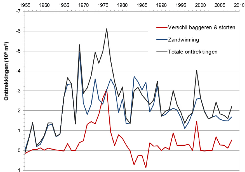
Figuur 7.12 Totaal Volume sediment dat uit de Westerschelde is onttrokken [ \text{m}^3 in beun].
