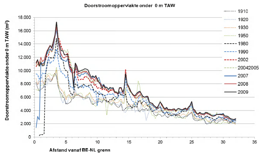
Figuur 7.6 Doorstroomoppervlakte onder 0 m TAW in de Beneden-Zeeschelde (Consortium T2009, concept 2013).
