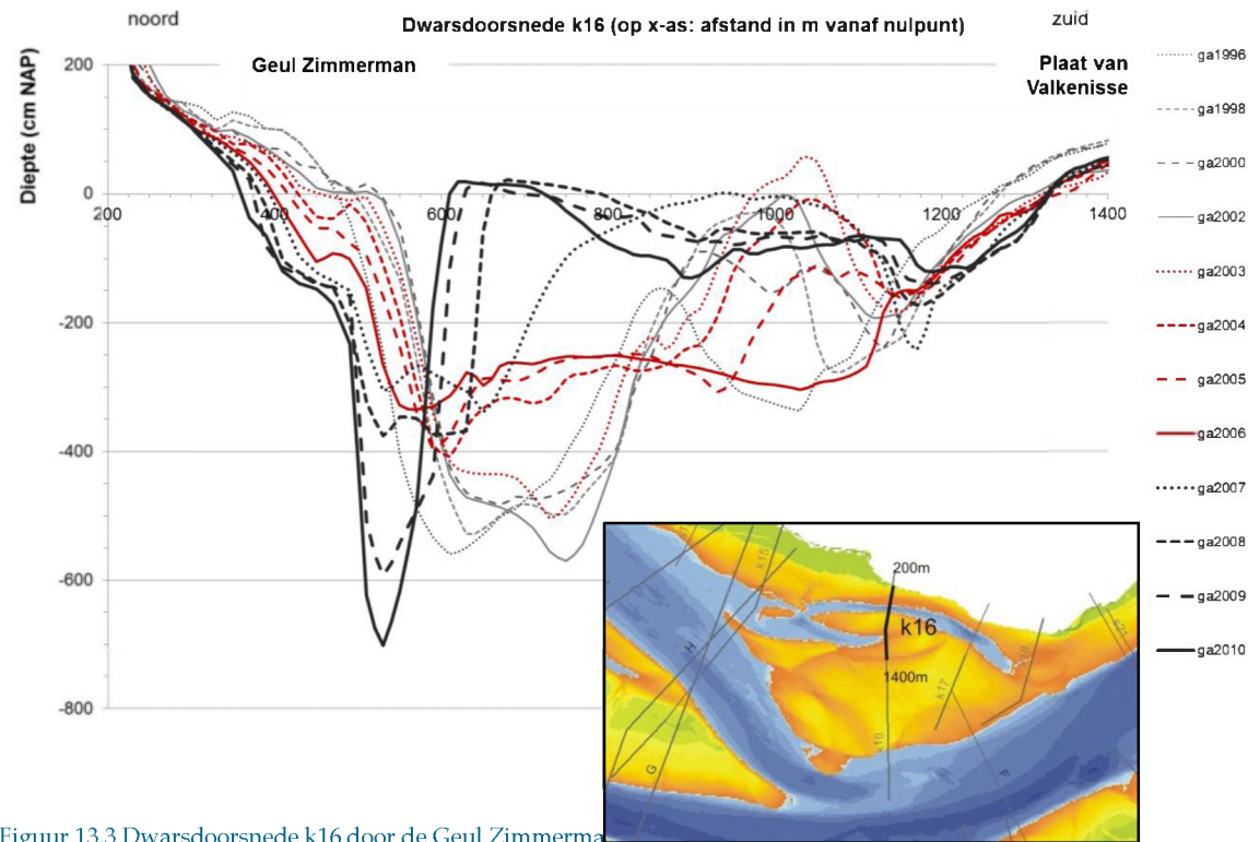
Figuur 13.3 Dwarsdoorsnede k16 door de Geul Zimmerman
