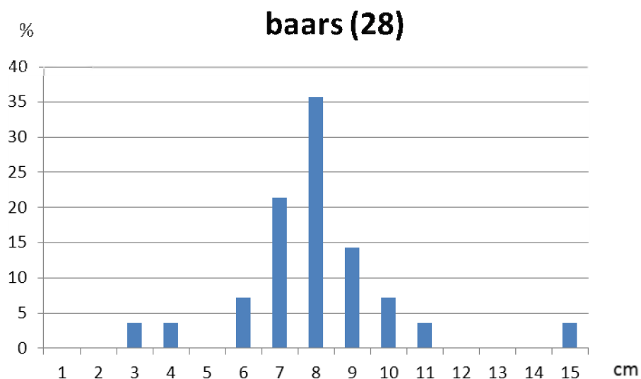
Figuur 7. Lengte frequentie (%) van totale vangst baars in de Durme (2013). Het aantal gemeten exemplaren staat tussen haakjes.
