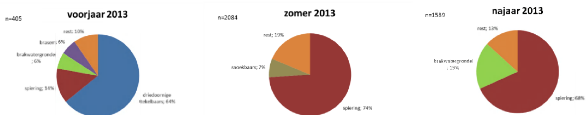
Figuur 4. Het relatief aantal gevangen individuen in de Durme tijdens de 2013 campagne.
