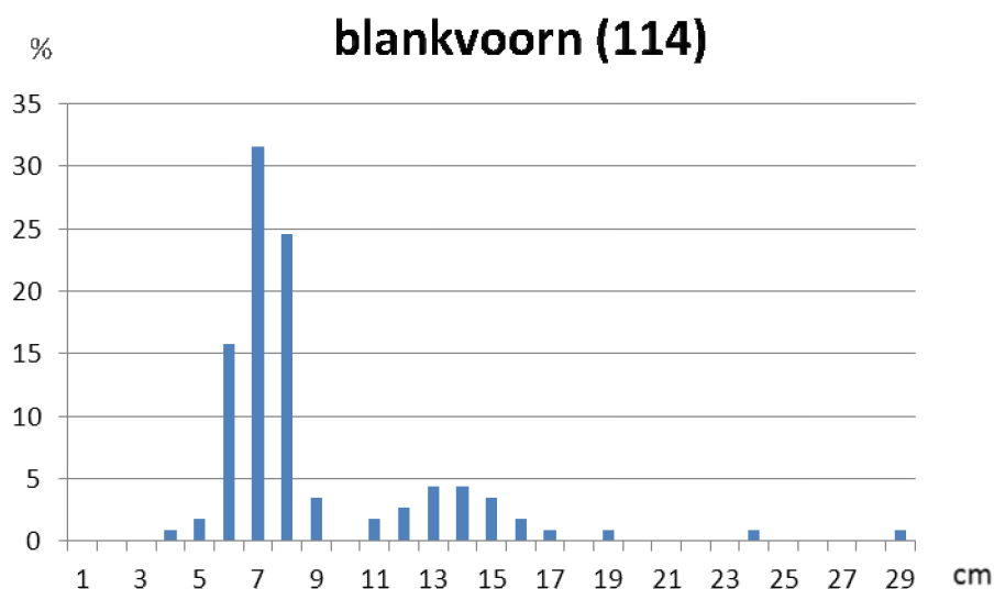
Figuur 8. Lengte frequentie (%) van totale vangst blankvoorn in Durme (2013). Het aantal gemeten exemplaren staat tussen haakjes.
