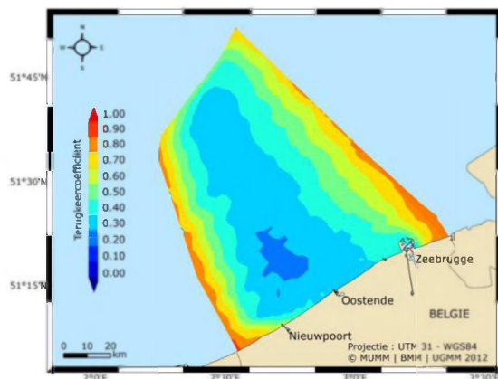
Figuren 6, 7 en 8: Verblijftijd (linksboven), expositietijd (rechtsboven) en terugkeercoëfficiënt (onder) in het BNZ [Bron: BMM 2012; Belgische Staat, 2012. Initiële Beoordeling voor de Belgische mariene wateren. Kaderrichtlijn Mariene Strategie – Art 8 lid 1a & 1b. BMM, Federale Overheidsdienst Volksgezondheid, Veiligheid van de Voedselketen en Leefmilieu, Brussel, België, 81 pp, blz 15].
