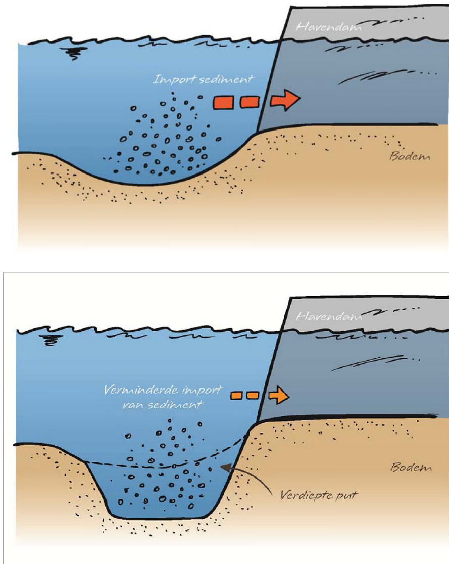
Figuur 28. Effect van de lokale verdieping voor de haven op het sedimenttransport
