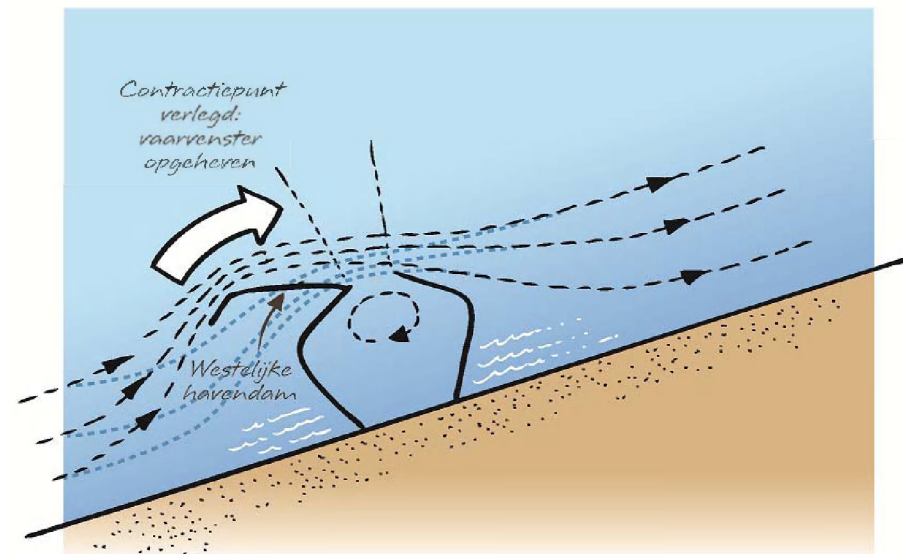
Figuur 30. Contractie van de stroming ter hoogte van de haven van Zeebrugge met (zwart) en zonder (blauw) uitbreiding van de westelijke havendam
