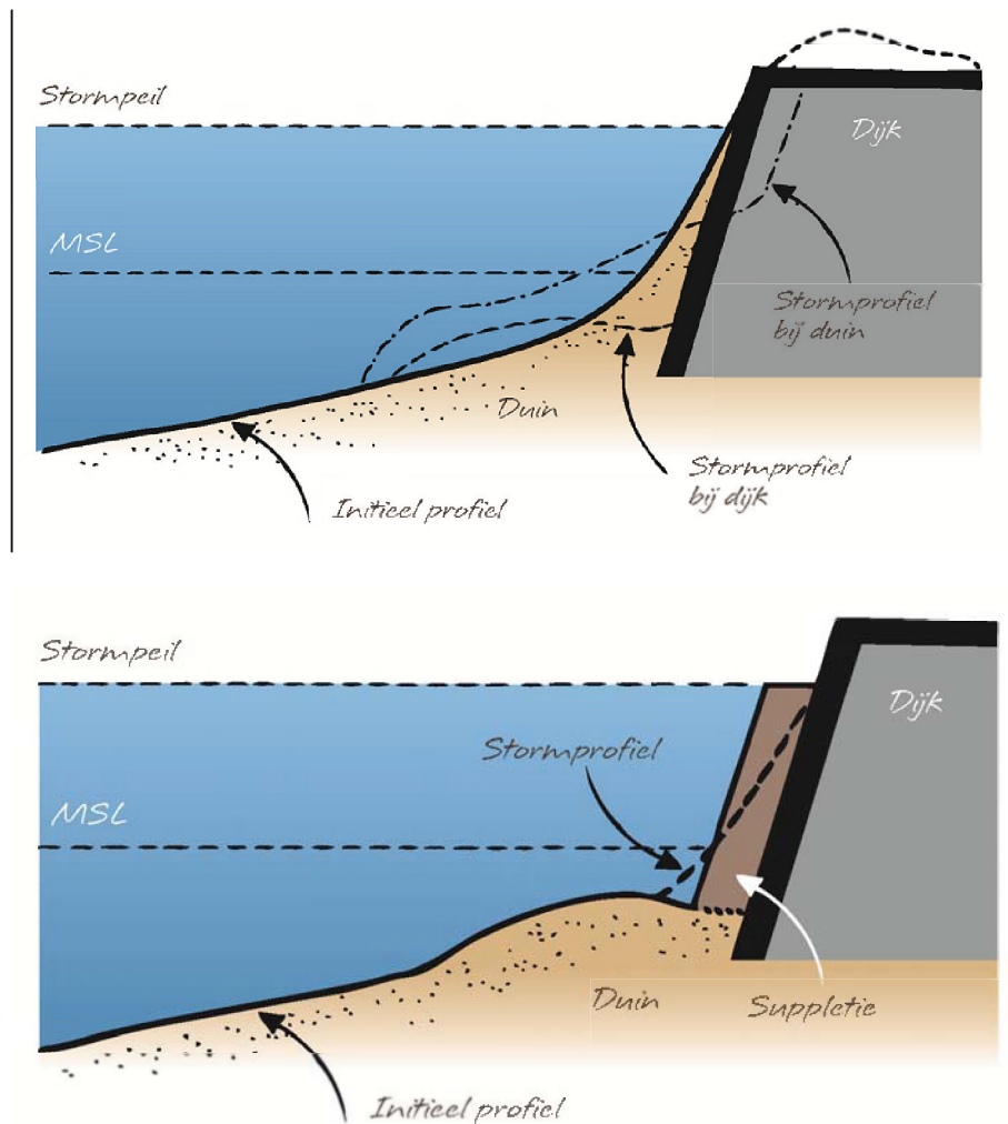
Figuur 13. Effect van een dijk op het natuurlijke strandprofiel – aanleiding tot suppleties
