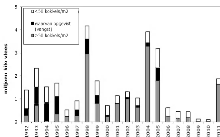
Figuur 5. De septemberschatting van de kokkelbiomassa in de Westerschelde in de periode 1992-2011, berekend uit de voorjaarsinventarisaties van IMARES. Er is onderscheid gemaakt in bestand in bevisbare dichtheden : meer dan 50 kokkels per m 2 , behaalde vangsten : deel van het bestand dat is opgevisst (zwart) en bestand in niet bevisbare dichtheden : 50 kokkels per m 2 en minder.
