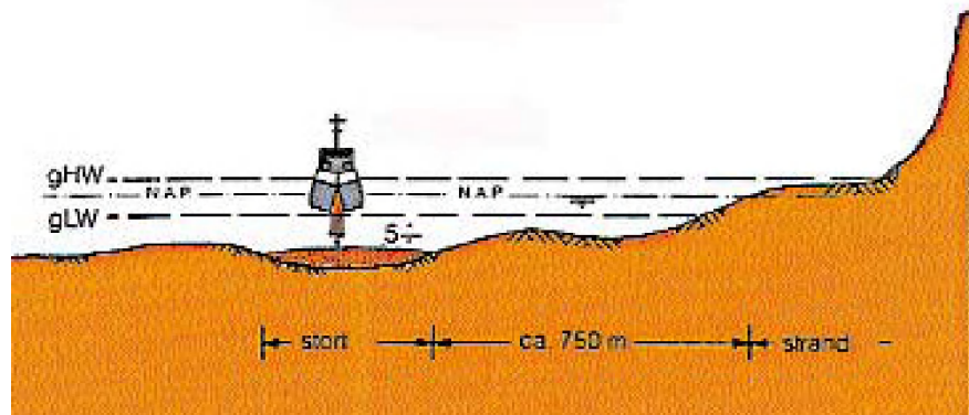
Figuur 8.1. Schematisch profiel van de vooroever met brekerbanken en de positie van de vooroeversuppletie.
