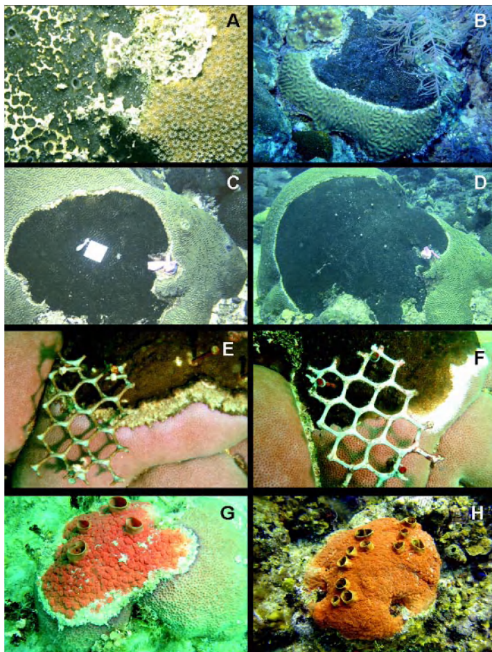
Figura 4-8 (Página siguiente). Esponjas excavadoras incrustantes del Caribe colombiano. (A) Chiona aprica en coral Solenastrea bournoni , San Andrés (campo horizontal aprox. 7.2 cm). (B) Chiona caribbaea en coral Diploria strigosa , Providencia (campo horizontal aprox. 1.5 m). (C) y (D) Chiona tenuis en coral Diploria strigosa , Islas del Rosario; vista inicial (C) y a los 13 meses (D), intervalo en el que la esponja avanzó lateralmente sobre el coral unos 15-20 cm (marca blanca en el centro de C tiene 5 cm de lado). (E) y (F) Chiona tenuis en coral Siderastrea siderea , Islas del Rosario, con una malla plástica para evitar el acceso de peces a la frontera entre el coral y la esponja; (E) vista inicial con una banda coral mordido por peces coralívoros unos días antes; (F) después de 6 meses; nótese que bajo la malla la esponja ha avanzado muy poco y que fuera de la malla continúa el avance, precedido de mordiscos de peces coralívoros (area blanca) (diámetro del ojo de la malla 3 cm). (G) Chiona delitrix en coral Siderastrea siderea , San Andrés, mostrando la banda de muerte que rodea la esponja y el oscurecimiento del coral afectado (diámetro aprox. de la esponja 30 cm). (H) Chiona delitrix , San Andrés, cubriendo completamente una colonia de coral (diámetro aprox. de la esponja 40 cm).
