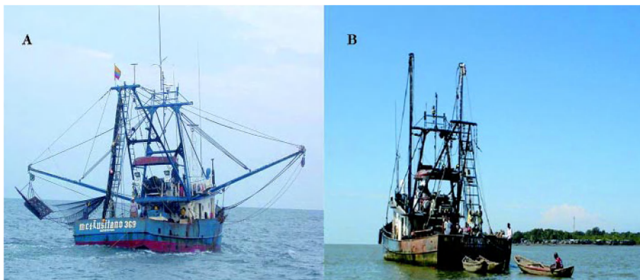
Figura 10-30. Embarcaciones pesqueras de la flota industrial del Pacífico colombiano usadas en los cruceros de pesca experimental. A = Alexander, B = Lusitano.
