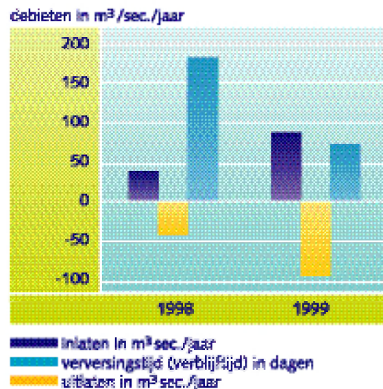
Figuur 2.2: Debieten van in- en uitlaten Brouwerssluis, verdamping en neerslag plus polder waterlozingen over de periode 1998 t/m 1999
