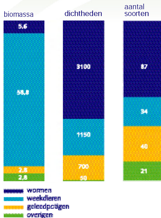
Figuur 5.1: Verdeling van gemiddelde biomassa (gram asvrijdroogge wicht/m²), gemiddelde dichtheid (aantal per m²) en aantal aangetroffen soorten per diergroep.
