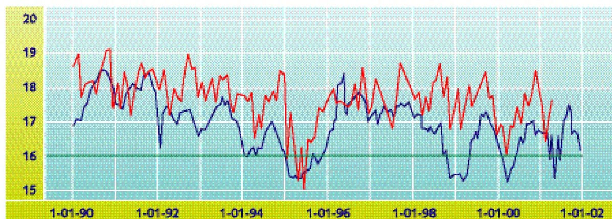
Figuur 2.3: Verloop in de tijd van het zoutgehalte in het Grevelingenmeer (meetpunt Dreischor, binnendijks) en het inlaatswater bij de Brouwerssluis (BG8, buitendijks)
