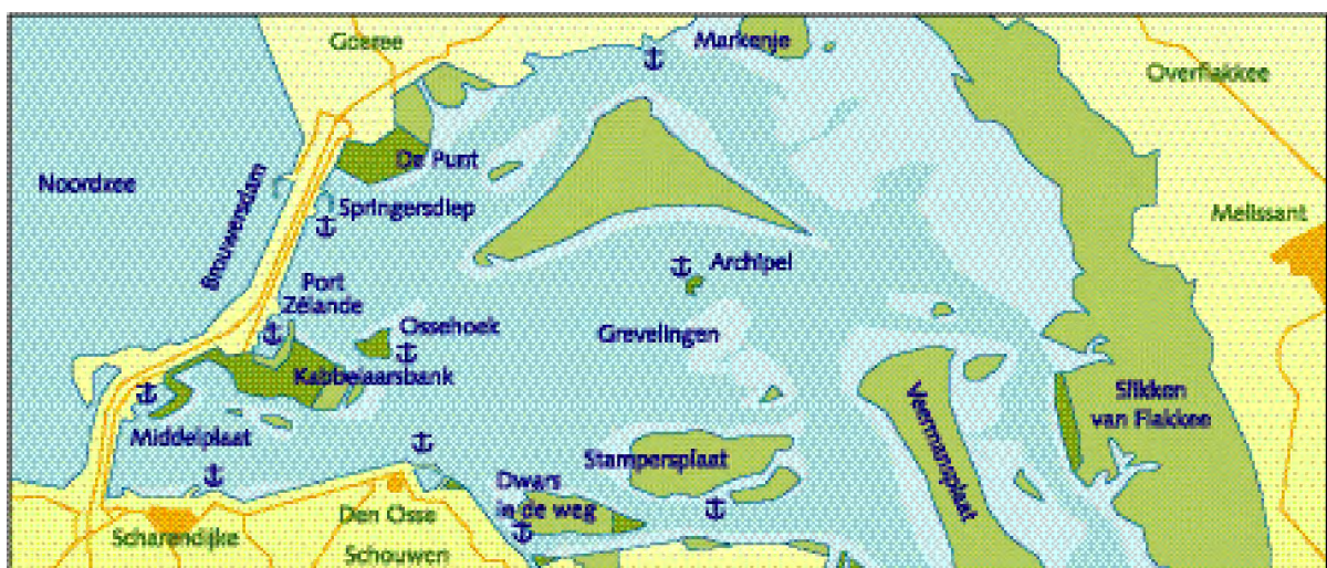
Figuur 1.1: De historische ontwikkeling van het Grevelingenmeer (uit: Visser J. 1995, zie bronnen)
