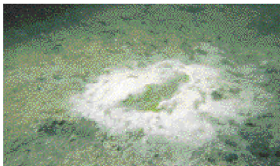
Schimmelplek op de bodem als gevolg van zuurstofloosheid, karakteristiek voor de diepere delen van het meer
