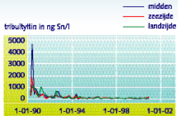
Figuur 2.8: Verloop van de TBT concentraties in de haven van Scharendijke in de periode 1990 t/m 2000
