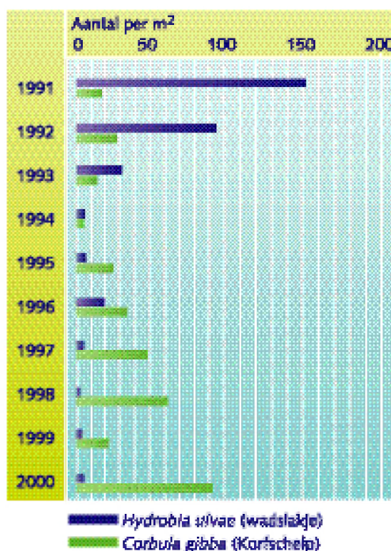
Figuur 5.2: Veranderingen in gemiddelde dichtheden van het wadslakje ( Hydrobia ulvae ) en de kortschelp ( Corbula gibba ) in het Grevelingenmeer over de periode 1991 – 2000
