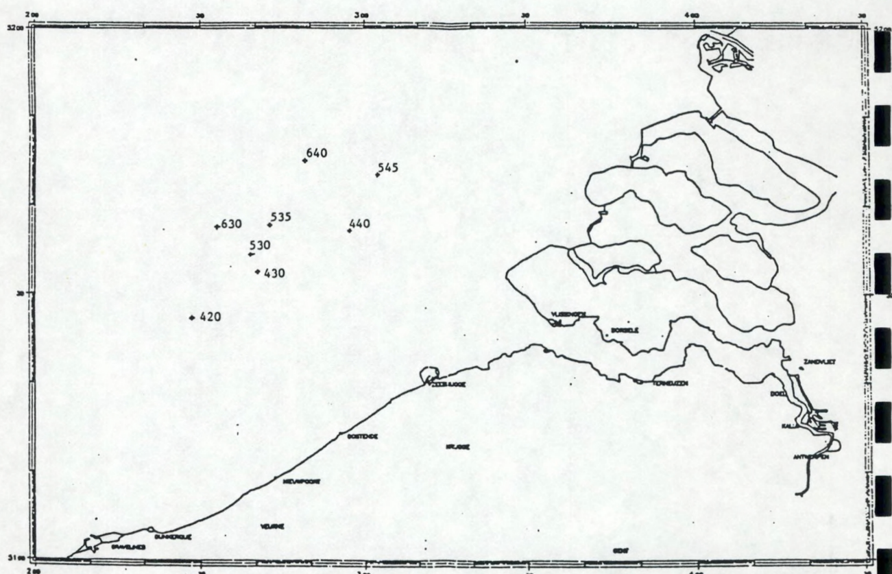
Ligging van de acht stations in de Zuidelijke Bocht van de Noordzee.
