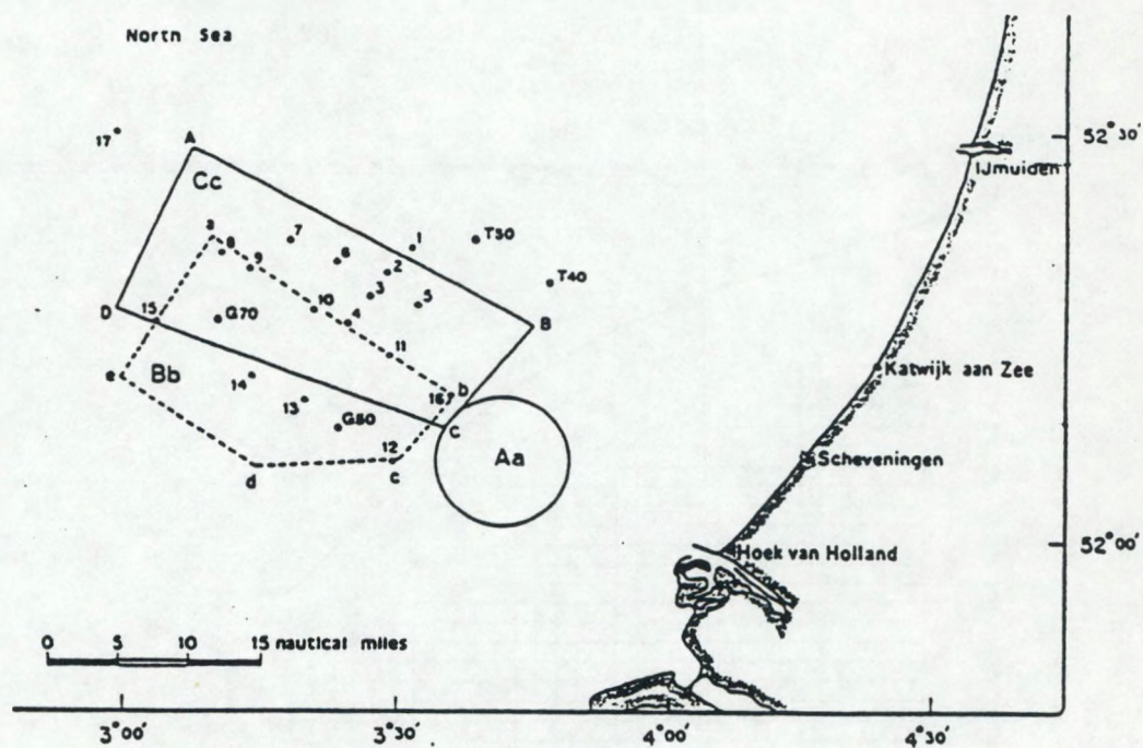
fig. 2a : \text{TiO}_2 -dumpingsgebied op het Nederlands Continentaal Plat
