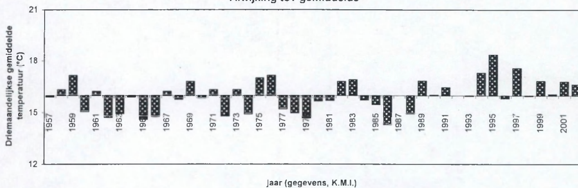
Fig. 4.5 Koksijde, jul-aug-sep gemiddelde temperatuur (°C) 1957-2002 Afwijking tov gemiddelde
