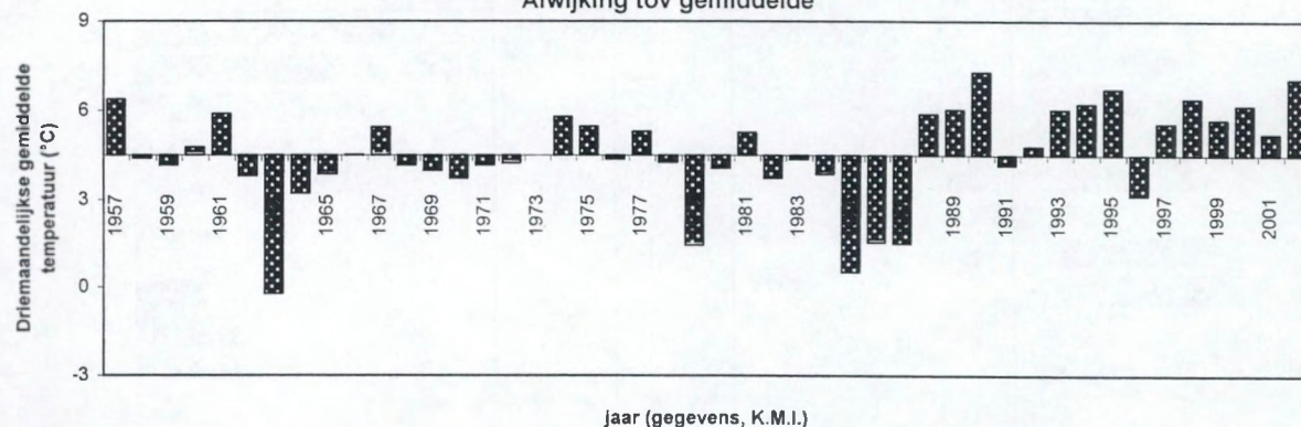
Fig. 4.3 Koksijde, jan-feb-mrt gemiddelde temperatuur (°C) 1957-2002 Afwijking tov gemiddelde
