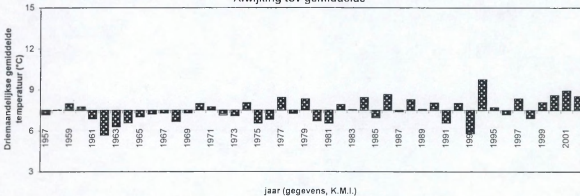
Fig. 4.6 Koksijde, okt-nov-dec gemiddelde temperatuur (°C) 1957-2002 Afwijking tov gemiddelde
