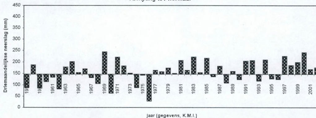
Fig. 4.9 Koksijde, jul-aug-sep neerslag (mm) 1957-2002 Afwijking tov normaal
