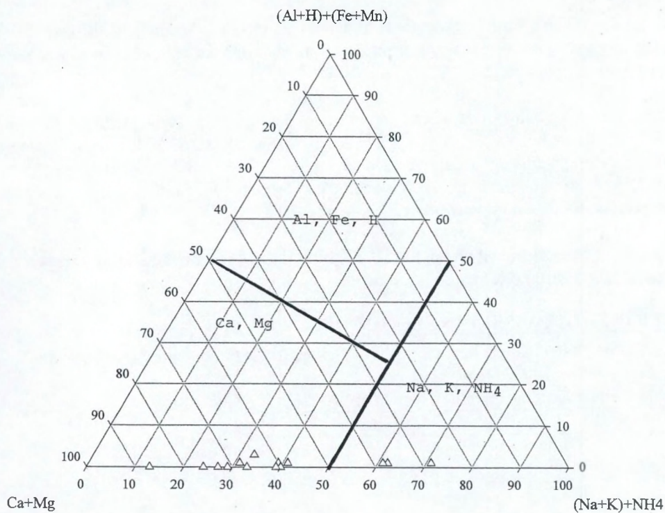
Fig. 6.3. : Bepaling van het type, kationen - 5/9/2002
