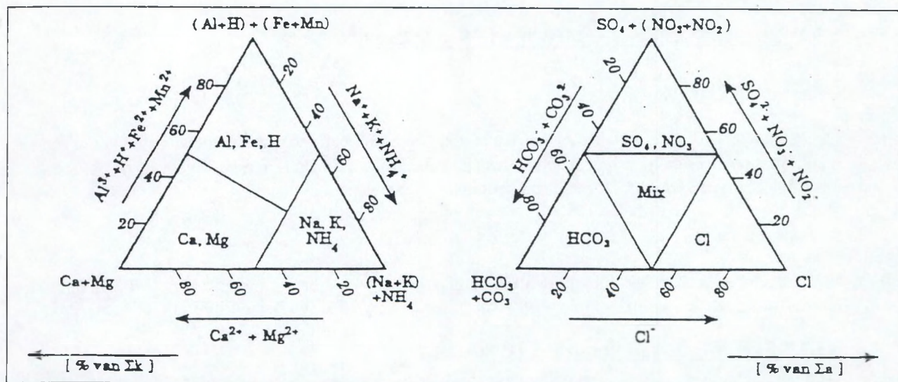
Fig. 3.1 : Bepaling van het watertype (Stuyfzand, 1986)
