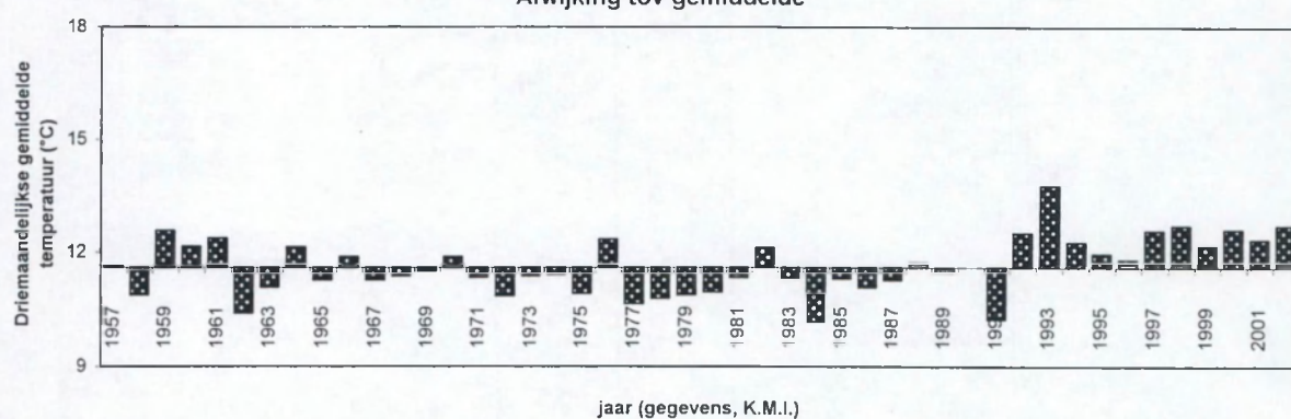
Fig. 4.4 Koksijde, apr-mei-jun gemiddelde temperatuur (°C) 1957-2002 Afwijking tov gemiddelde
