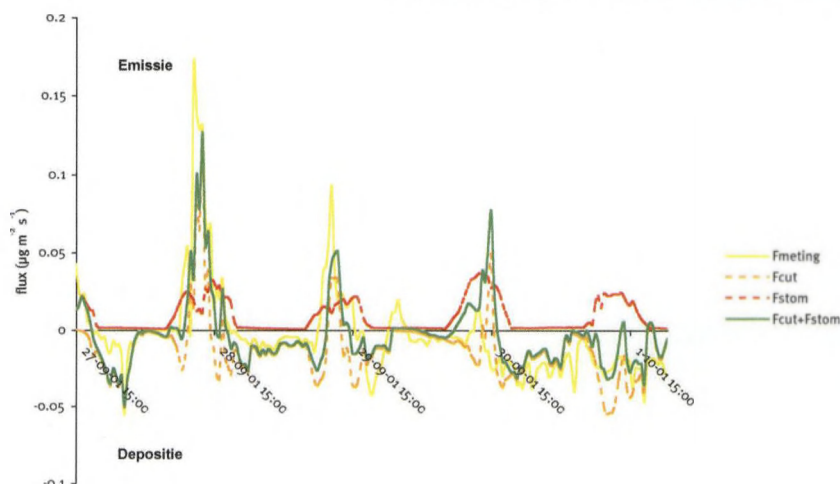
Verloop van gemeten en gemodelleerde ammoniakfluks (deze laatste opgesplitst in stomataire en cuticulaire fluks)
