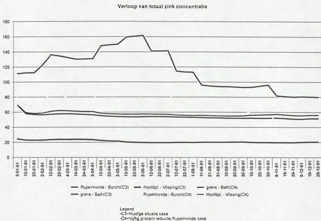
Figuur 9.4 Verloop van concentraties van totaal zink voor de case van de huidige situatie resp. de case met een halvering van de stofvracht bij RupeImonde
