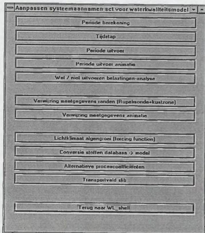
Figuur 8.2 Overzicht van systeemaannamen met toegang tot invoerbestanden van DELWAQ
