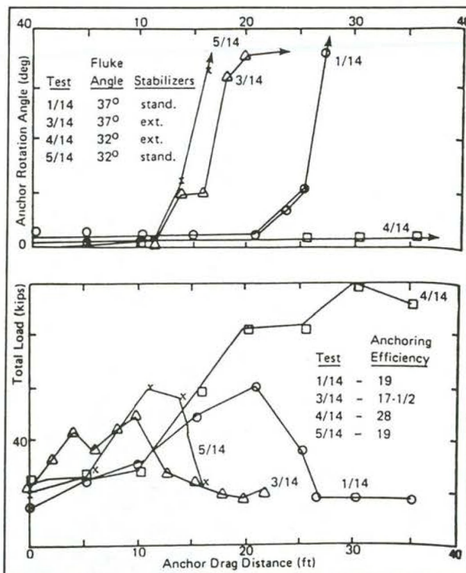
Figuur 4.7 Invloed stabilisator en vloeihoeck op stabiliteit en houdkracht [Taylor, 1981]
