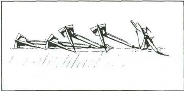
Figuur 4.4 Kantelen anker door combinatie harde bodem met grote vloeihoeek [Vryhof, 1990]
