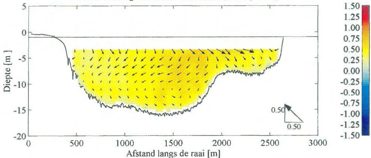
Globale verdeling van de stroomsnelheid (u-component)
