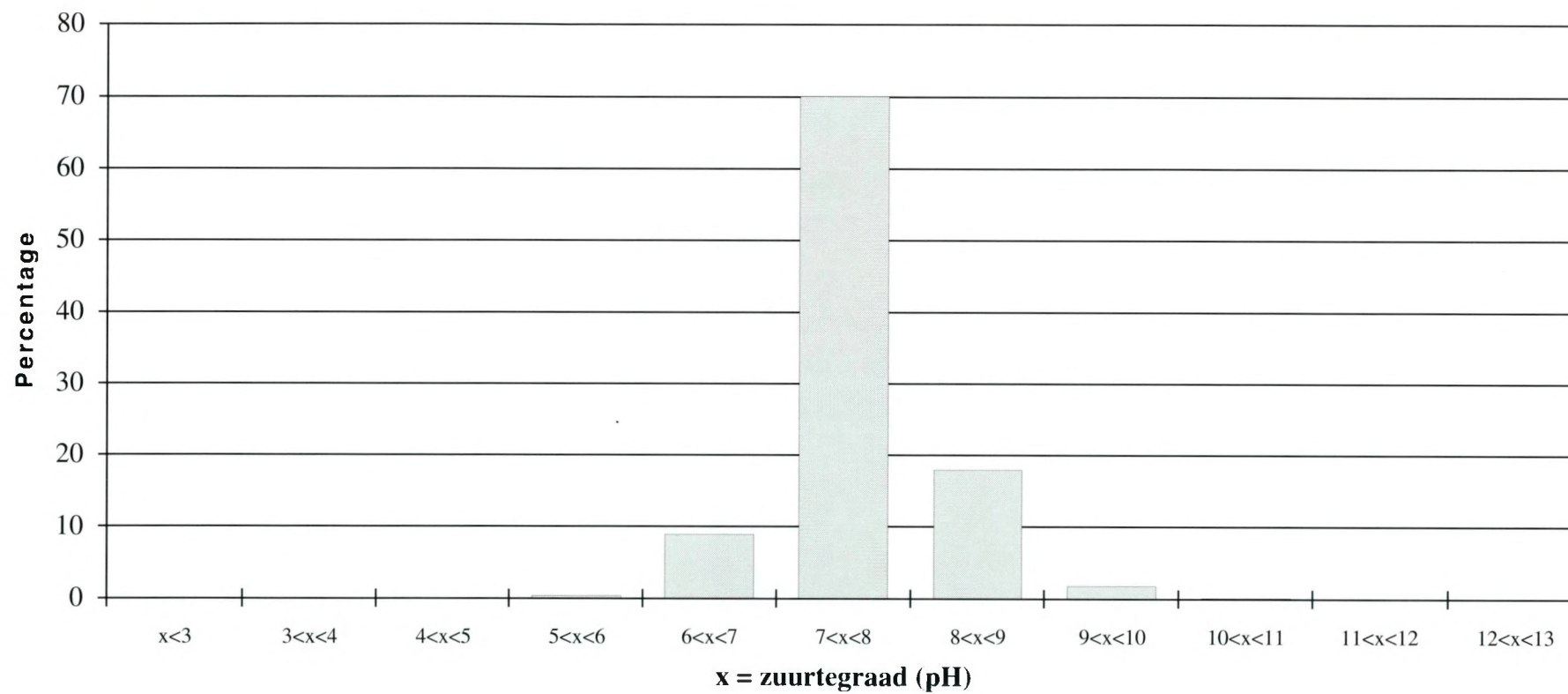
Fig. 14 : Frequentiedistributie pH-waarnemingen VMM-meetnet 1990 (8725 waarnemingen)
