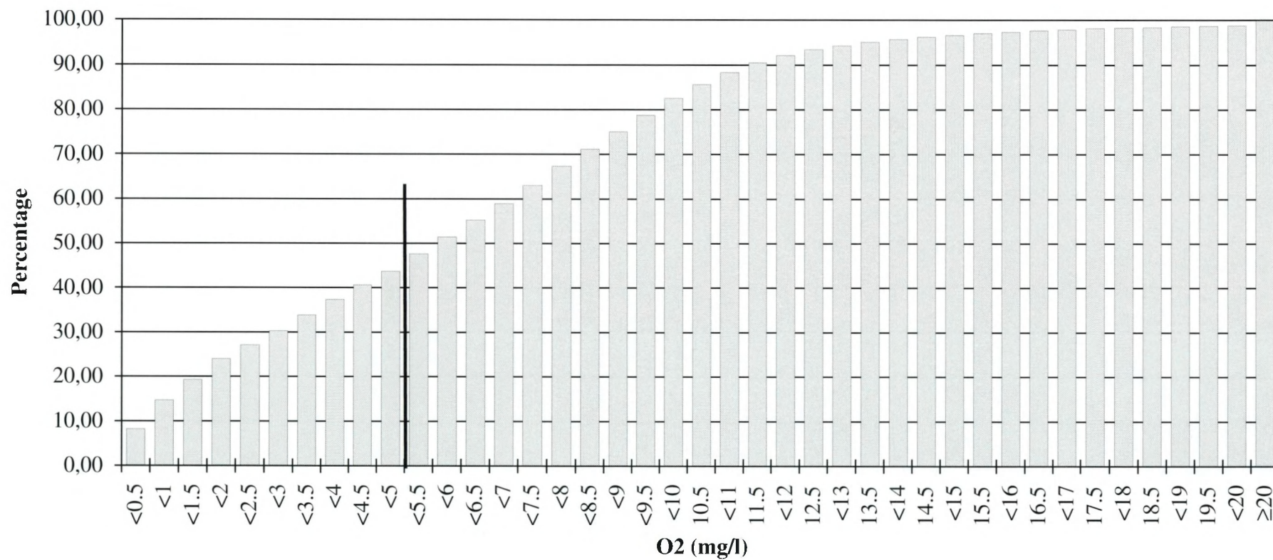
Fig. 3 : Cumulatieve frequentiedistributie zuurstofconcentratie VMM-meetnet 1990
