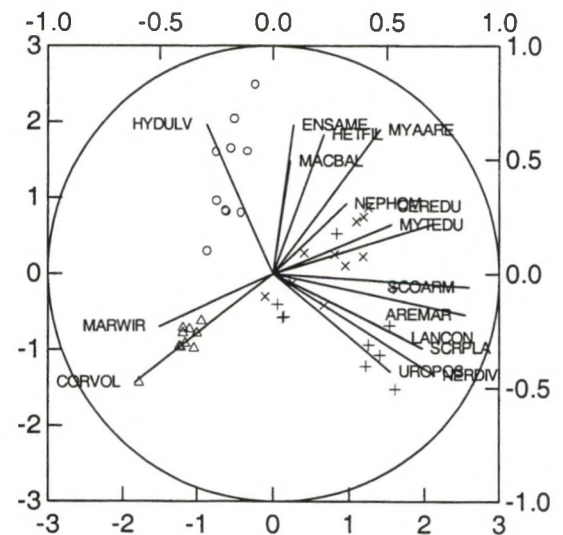
Figuur 4. Principale componenten analyse van het macrozoöbenthos (biomassa in de winter) in de vier deelgebieden Balgzand (x), sublitorale westelijke Waddenzee (O), Piet Scheveplaat (+) en Heringsplaat (Δ). Soortenafkortingen zie p. 10.
