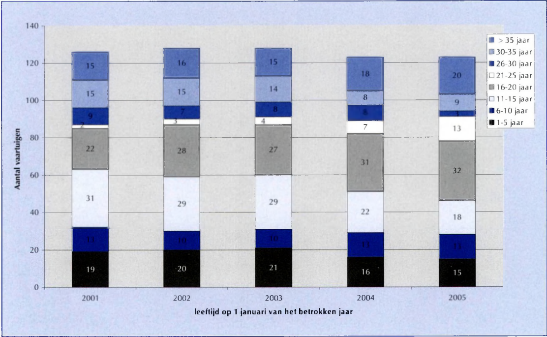
Grafiek 10.6 : Evolutie leeftijdsopbouw vaartuigen/casco
