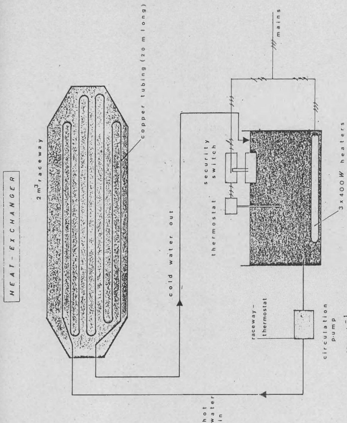
Figuur 9: Schematische voorstelling van de warmtewisselaar in een 2 \text{ m}^3 raceway
