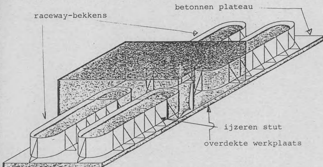
Figuur 11: Overzichtsschets pilootinstallatie te Sas Slijkens ( Bredene)
