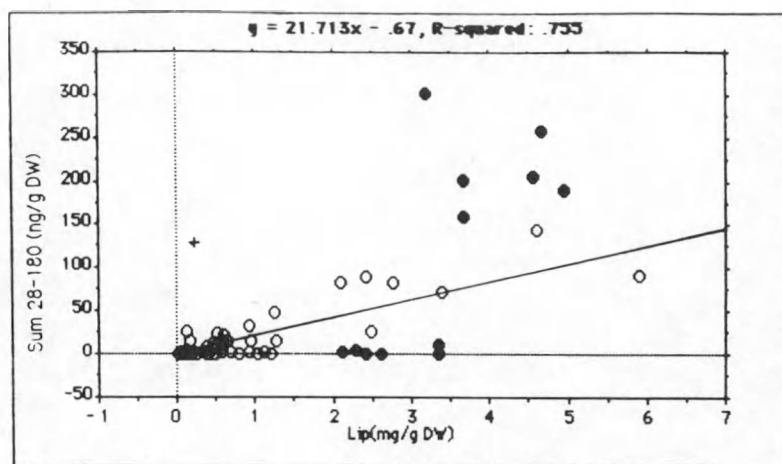
Figuur 3.3.10: Relatie tussen de PCB besmetting en de lipidegehalten van oppervlakte sedimenten uit het Schelde estuarium en het Belgisch Kontinentaal Plat in de periode oktober 1987 - maart 1988. Regressie en korrelatie: zie ook figuur 3.3.12.
