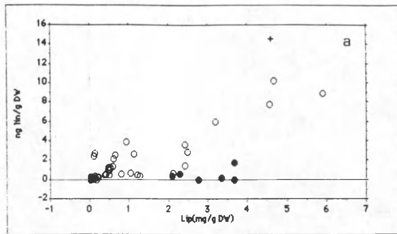
Figuur 3.4.5: Relatie tussen de lindaanbesmetting en de lipidegehaltes van oppervlakte sedimenten uit het Schelde estuarium en het Belgisch Kontinentaal Plat in de periode oktober 1987 - maart 1988. Regressie en correlatie zie figuur 3.4.6.
