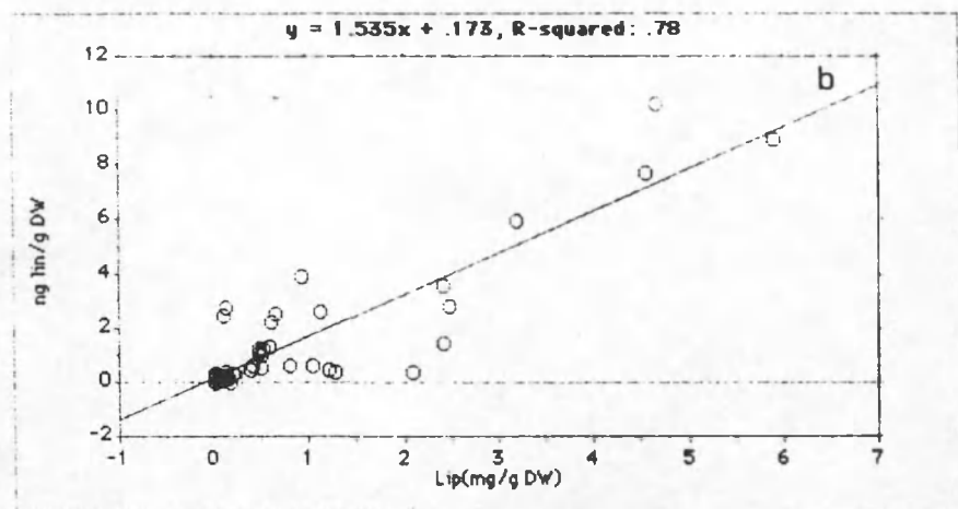
Figuur 3.4.5: Relatie tussen de lindaanbesmetting en de lipidegehaltes van oppervlakte sedimenten uit het Schelde estuarium en het Belgisch Kontinentaal Plat in de periode oktober 1987 - maart 1988. Regressie en correlatie zie figuur 3.4.6.
