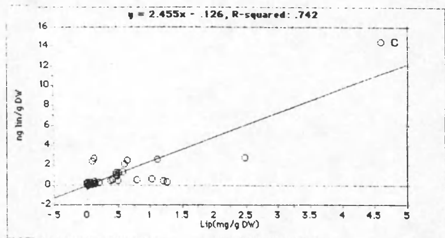
Figuur 3.4.7: Relatie tussen de lindaanbesmetting en de lipidegehaltes van oppervlakte sedimenten buiten de zone Kalo - Doel.
