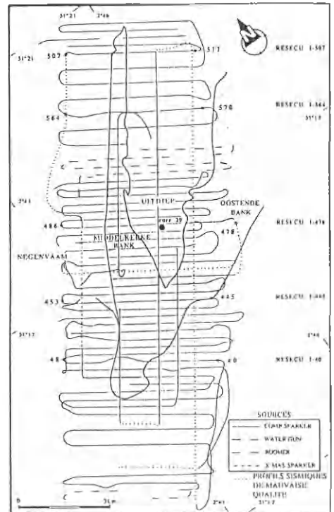
Fig. 8 : Profils sismiques à haute résolution enregistrés sur le Middelkerke Bank en décembre 1990
