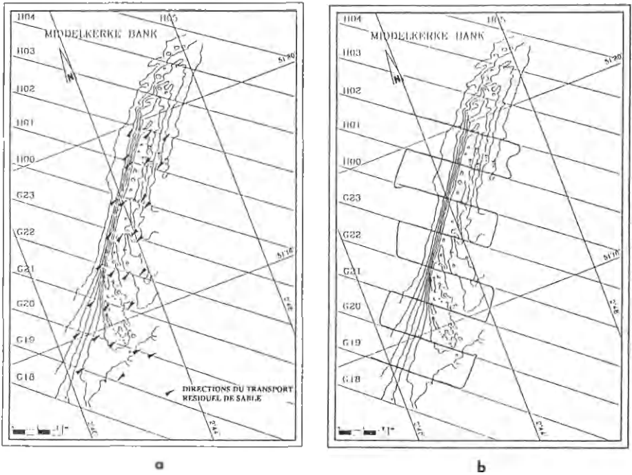
Fig. 3 : a) Les directions du transport résiduel de sable b) Profils enregistrés en octobre 1990.
