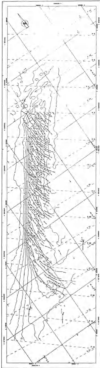
Fig. 5 : Les vagues de sable du Middelkerke Bank (cartographie basée sur des enregistrements réalisés en mai 1990).
