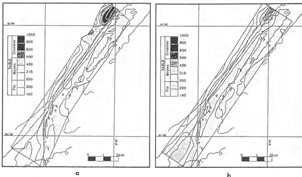
Fig. 7 : a) Grain moyen calculé sur le sédiment brut. b) Grain moyen calculé sur le sédiment décalcifié.
