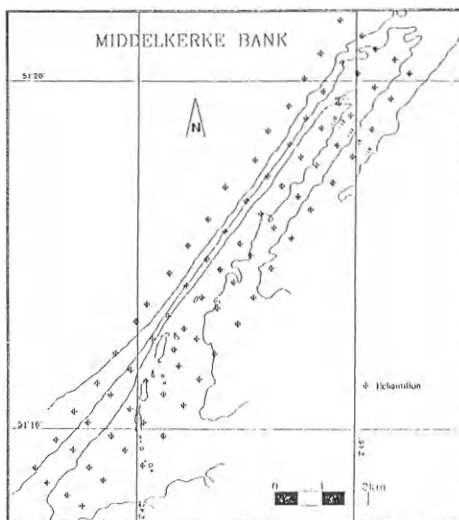
Fig. 6 : Les échantillons pris sur le Middelkerke Bank
