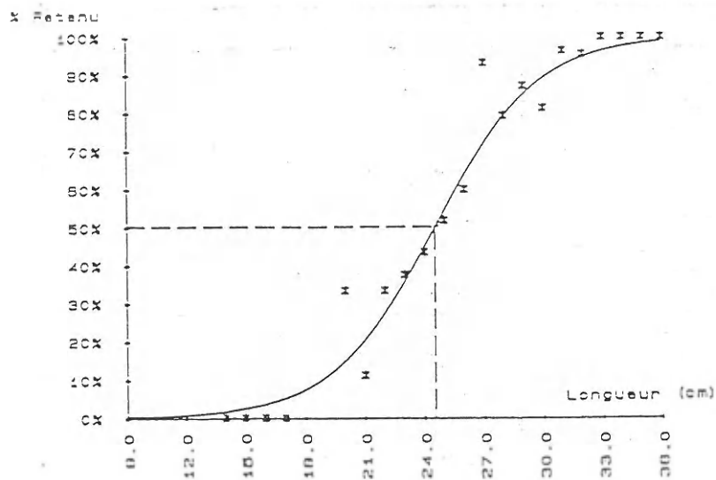
Figure 20 - Courbe de sélectivité tracée à partir des données de la deuxième sortie (poche en polyester à bâbord)
