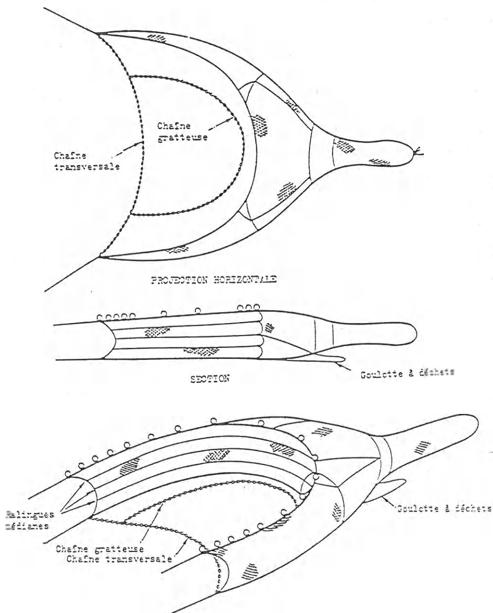
Figure A 1 - Configuration opérationnelle d'un chalut à crevette avec une nappe de séparation verticale utilisé aux Etats-Unis (d'après ELLIS, 1973).
