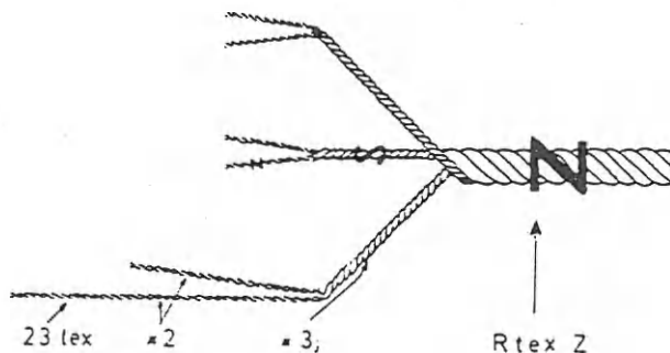
Figure 18 - Exemple d'une désignation complète d'un fil câblé.
