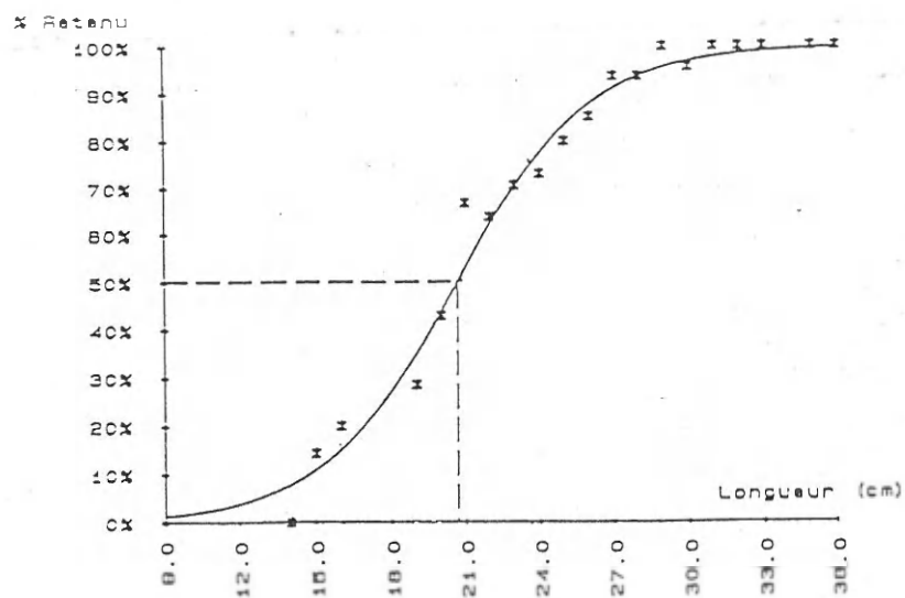
Figure 10 - Courbe de sélectivité tracée à partir des données de la deuxième sortie (poche courte à mailles losanges à bâbord)
