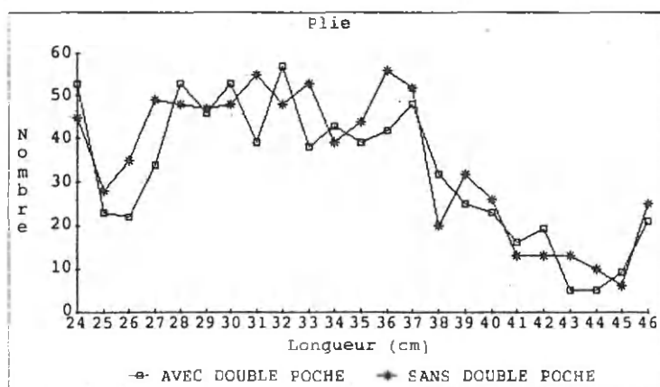
Figure 55 - Comparaison des captures de la poche avec double poche à celles de la poche sans double poche (effet de masque).
