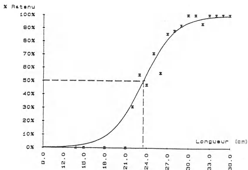
Figure 45 - Courbe de sélectivité de la poche en polyéthylène tracée à partir des données combinées des deux sorties.
