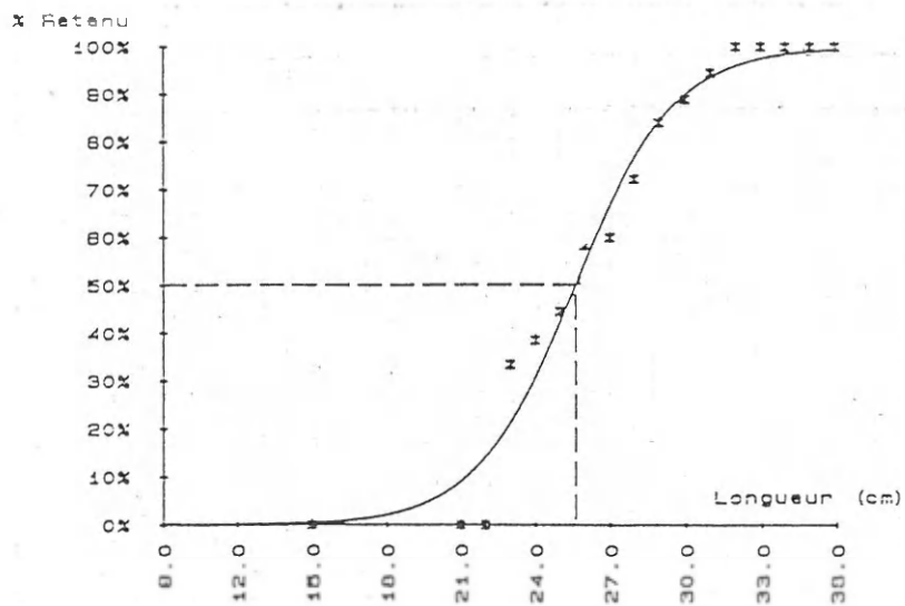
Figure 27 - Courbe de sélectivité tracée à partir des données de la deuxième sortie (poche de 85 mm de maillage à bâbord)
