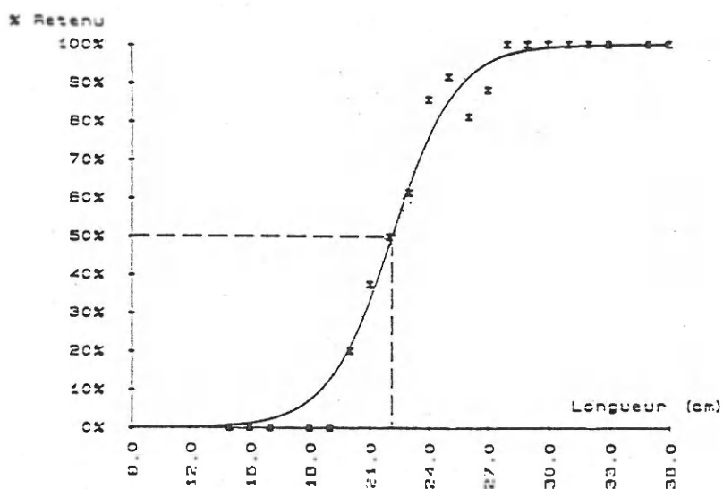
Figure 13 - Courbe de sélectivité tracée à partir des données de la première sortie (poche longue à mailles losanges à tribord)
