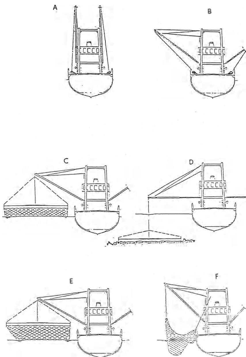
Figure 17 - Manoeuvres de filage et de virage en gréement double avec un chalutier à tangons utilisant des chaluts à perche (d'après DE BOER, 1969).
