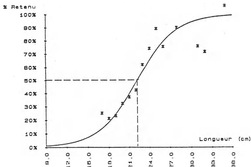
Figure 30 - Courbe de sélectivité de la poche à mailles carrées tracée à partir des données combinées des deux sorties (méthode de chalutage en gréement double).
