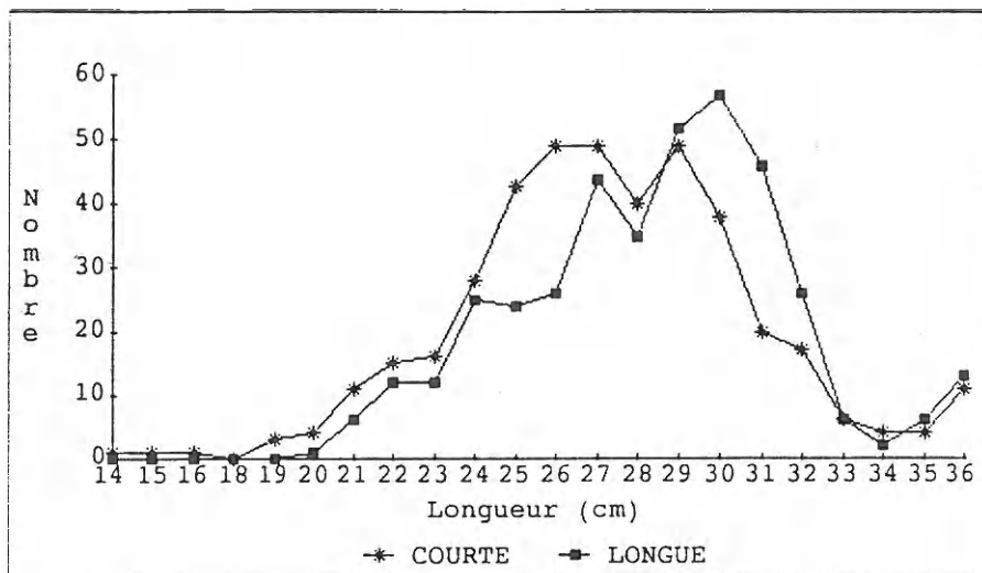
Figure 39 - Comparaison des captures de la poche courte à celle de la poche longue.
