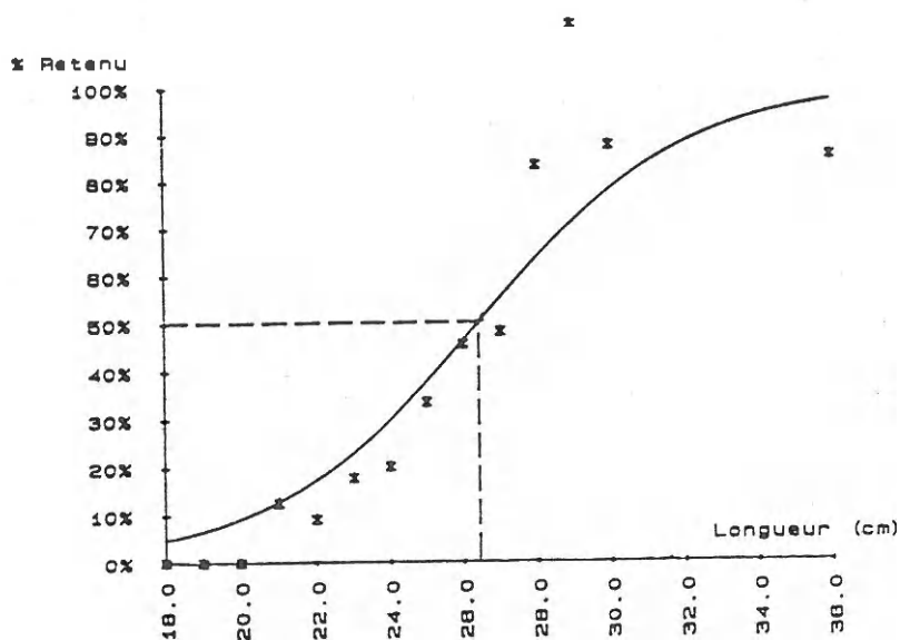
Figure 56 - Courbe de sélectivité du chalut utilisé au large déterminée par la méthode de deux chaluts jumeaux.
