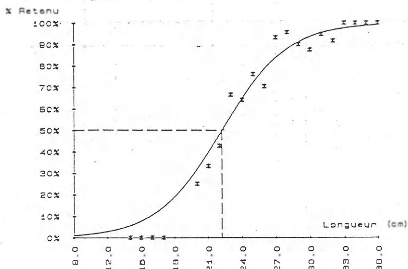
Figure 16 - Courbe de sélectivité tracée à partir des données de la première sortie (poche longue à mailles carrées à bâbord)
