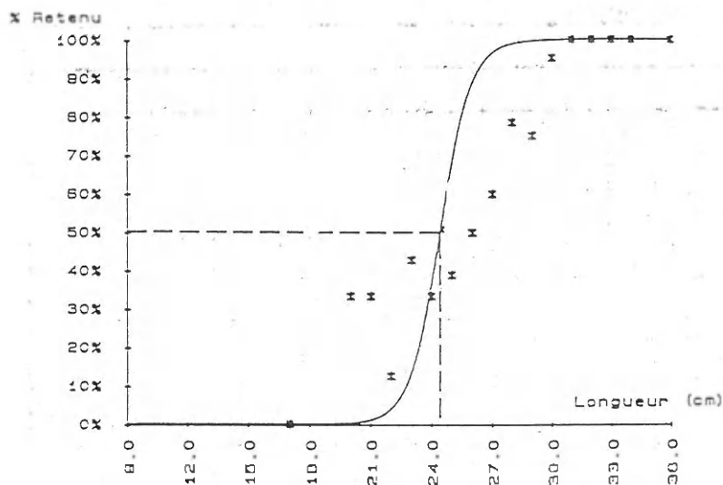
Figure 19 - Courbe de sélectivité tracée à partir des données de la première sortie (poche en polyester à tribord)
