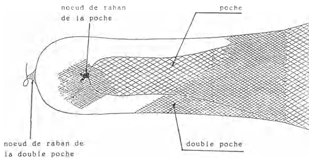
Figure 3 - Double poche complète.
