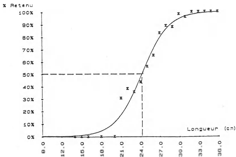
Figure 43 - Courbe de sélectivité de la poche en polyamide tracée à partir des données combinées des deux sorties.
