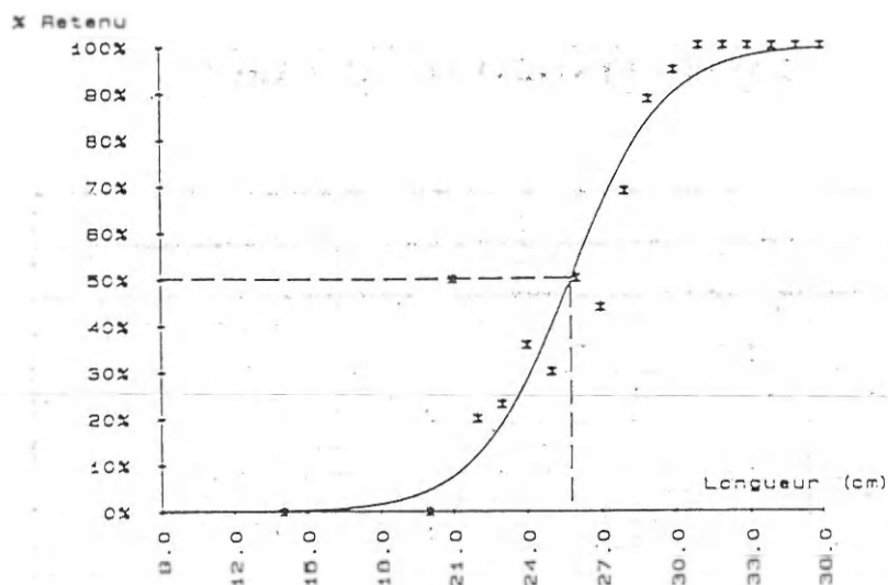
Figure 26 - Courbe de sélectivité tracée à partir des données de la première sortie (poche de 85 mm de maillage à tribord)
