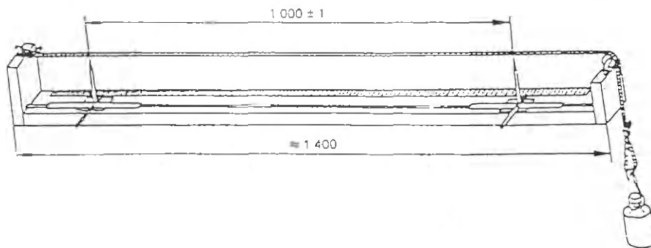
Figure 21 - Appareil pour la détermination de la variation de longueur.
