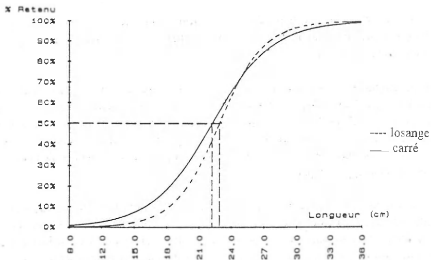
Figure 33 - Courbes de sélectivité de la poche à mailles losanges et de celle à mailles carrées (méthode de chalutage en gréement double).
