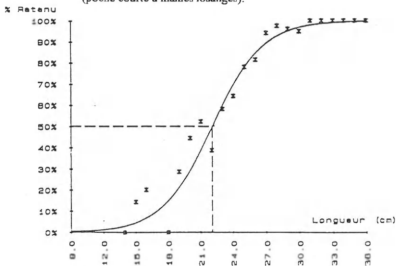
Figure 37 - Courbe de sélectivité de la poche courte à mailles losanges (tracée à partir des données combinées des deux sorties).
