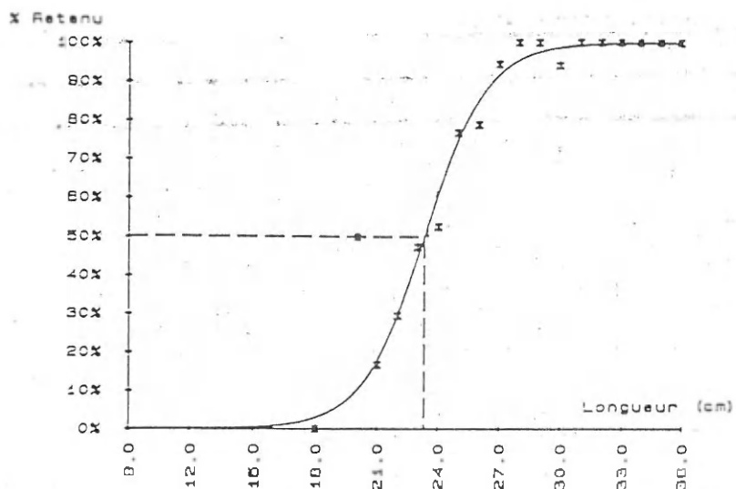
Figure 9 - Courbe de sélectivité tracée à partir des données de la première sortie (poche courte à mailles losanges à tribord)
