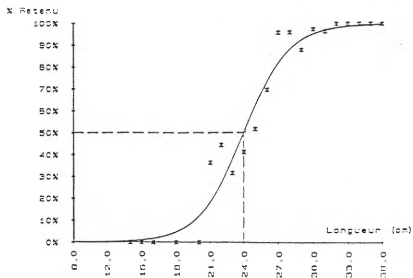
Figure 18 - Courbe de sélectivité tracée à partir des données de la deuxième sortie (poche en polyamide à bâbord)
