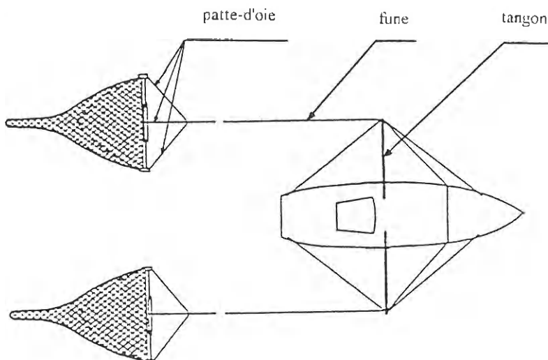
Figure 13 - Chalutage à perche en gréement double.
