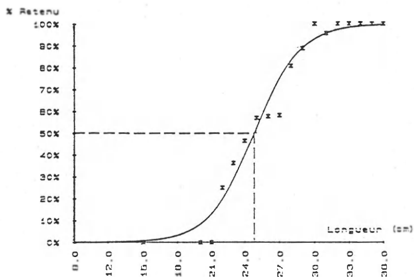
Figure 17 - Courbe de sélectivité tracée à partir des données de la première sortie (poche en polyamide à tribord)
