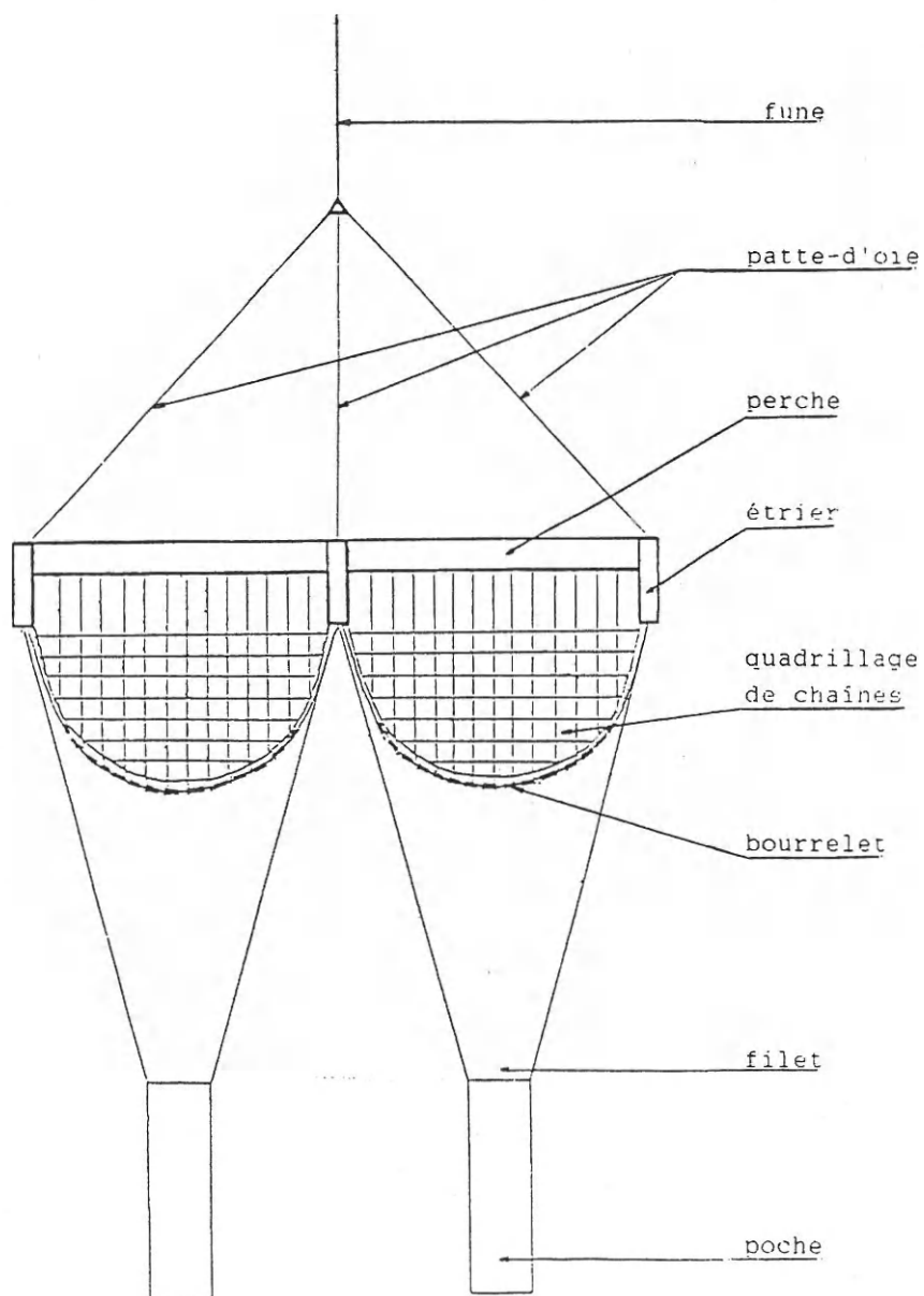
Figure 51 - Gréement des deux chaluts jumeaux.
