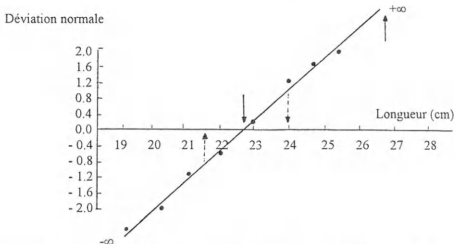
Figure 4 - Courbe de sélectivité pour le cabillaud tracée après transformation de pourcentages retenus en déviations normales (POPE et al., 1975).
