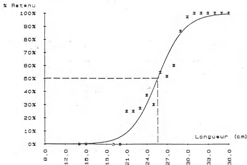
Figure. 46 - Courbe de sélectivité de la poche de 85 mm de maillage tracée à partir des données combinées des deux sorties.
