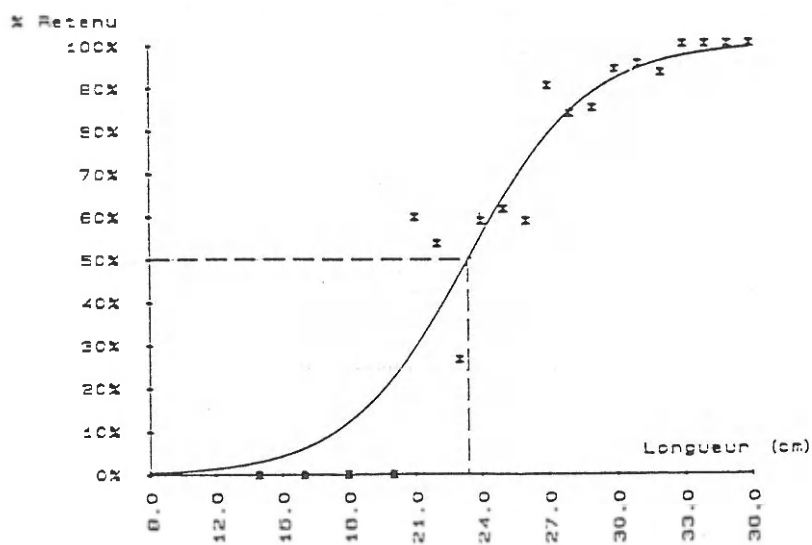
Figure 14 - Courbe de sélectivité tracée à partir des données de la deuxième sortie (poche longue à mailles losanges à bâbord)
