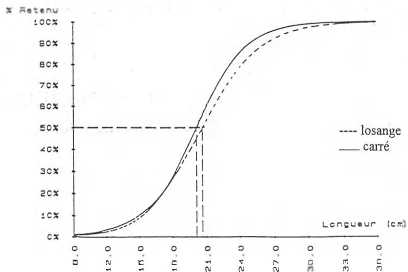
Figure 34 - Courbes de sélectivité de la poche à mailles losanges et de celle à mailles carrées (méthode de la double poche).
