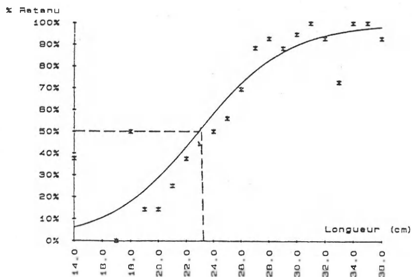
Figure 58 - Courbe de sélectivité du chalut à perche utilisé au large déterminée par la méthode de la double poche.
