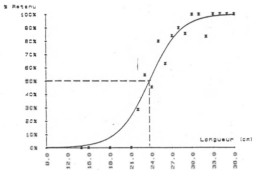
Figure 23 - Courbe de sélectivité tracée à partir des données de la première sortie (poche en polyéthylène à bâbord)
