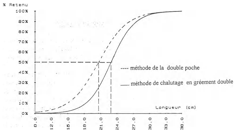
Figure 35 - Courbes de sélectivité obtenues par les deux méthodes expérimentales d'étude de la sélectivité (poche à mailles losanges).
