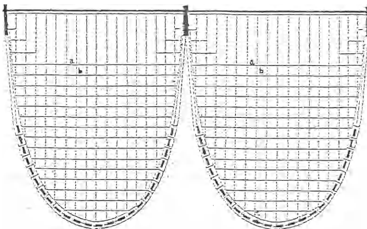
Figure 53 - Quadrillage de chaînes du chalut à perche utilisé au large.
