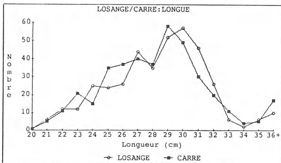
Figure 42 - Comparaison de la capture de la poche longue à mailles losanges à celle de la poche longue à mailles carrées.
