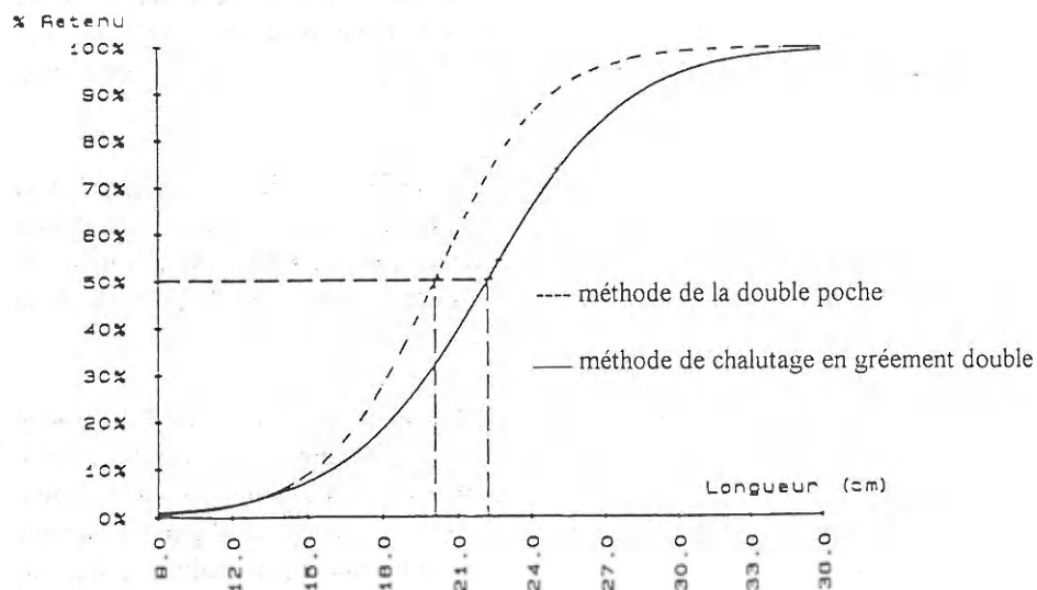
Figure 36 - Courbes de sélectivité obtenues par les deux méthodes expérimentales d'étude de la sélectivité (poche à mailles carrées).
