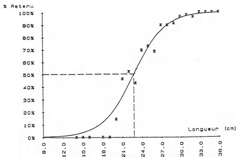
Figure 38 - Courbe de sélectivité de la poche longue à mailles losanges (tracée à partir des données combinées des deux sorties).
