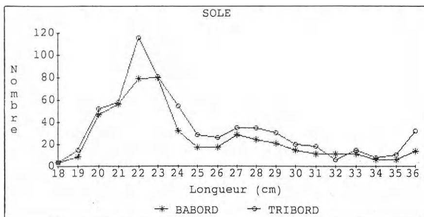
Figure 27 - Comparaison de l'efficacité de capture du chalut à bâbord à celle du chalut à tribord
