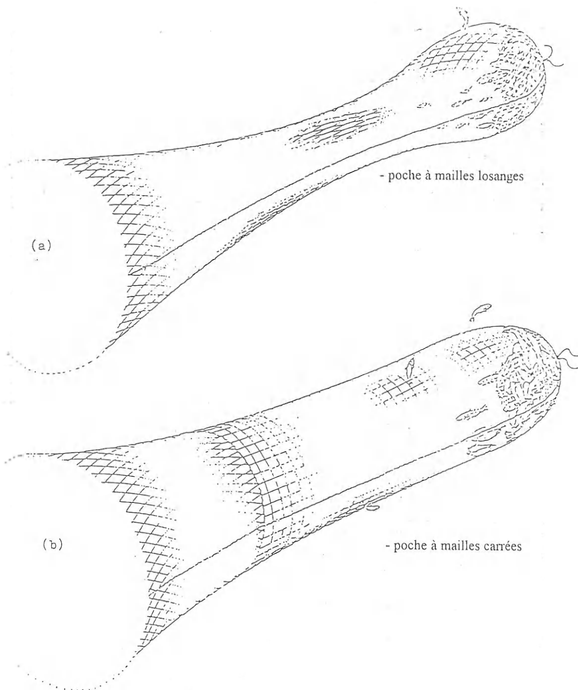
Figure 5 - Comparaison de la forme de la poche à mailles losanges à celle de la poche à mailles carrées au cours du chalutage (d'après ROBERTSON, 1982).
