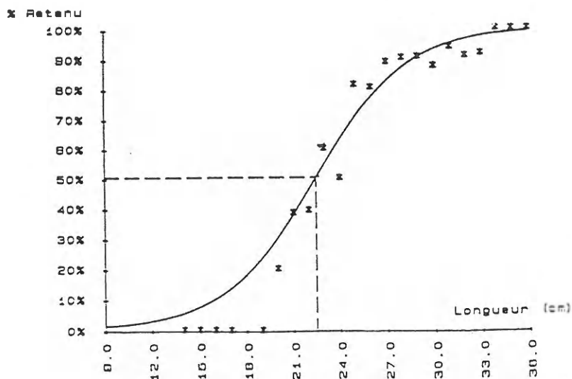
Figure 41 - Courbe de sélectivité de la poche longue à mailles carrées tracée à partir des données combinées des deux sorties.
