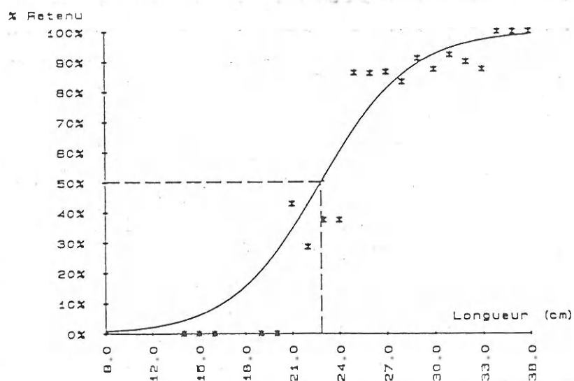
Figure 17 - Courbe de sélectivité tracée à partir des données de la deuxième sortie (poche longue à mailles carrées à tribord)
