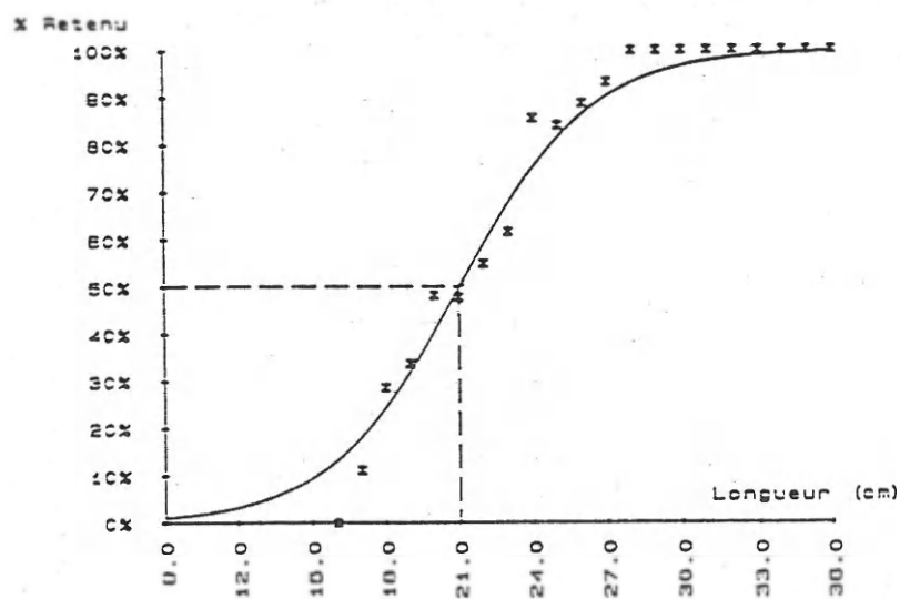
Figure 3 - Courbe de sélectivité tracée à partir des données de la première sortie (poche à mailles losanges à bâbord)
