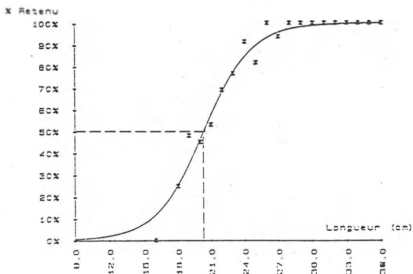
Figure 7 - Courbe de sélectivité tracée à partir des données de la première sortie (poche à mailles carrées à tribord)
