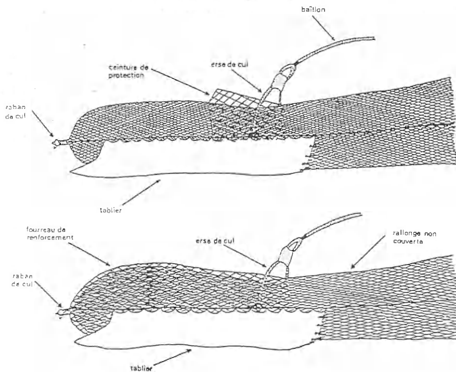
Figure 6 - Dispositifs de renfort ou de protection fixés à la poche (d'après BRABANT et NEDELEC, 1988)
