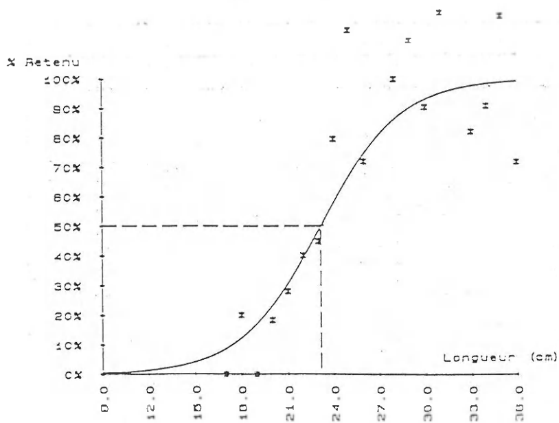
Figure 2 - Courbe de sélectivité tracée à partir des données de la deuxième sortie (poche à mailles losanges à bâbord)
