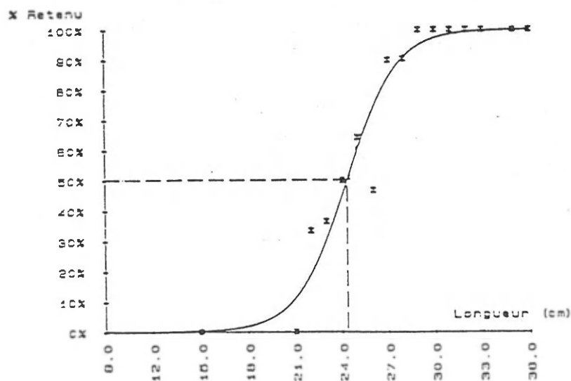
Figure 24 - Courbe de sélectivité tracée à partir des données de la deuxième sortie (poche en polyéthylène à tribord)
