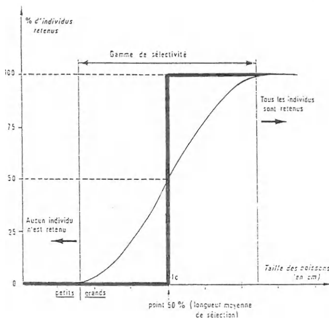
Figure. 1 - Exemple de courbe de sélectivité d'un chalut
