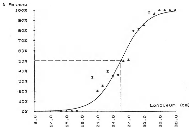
Figure 44 - Courbe de sélectivité de la poche en polyester tracée à partir des données combinées des deux sorties.
