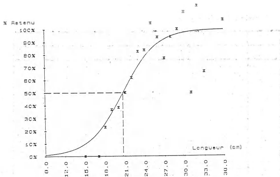
Figure 1 - Courbe de sélectivité tracée à partir des données de la première sortie (poche à mailles losanges à tribord)
