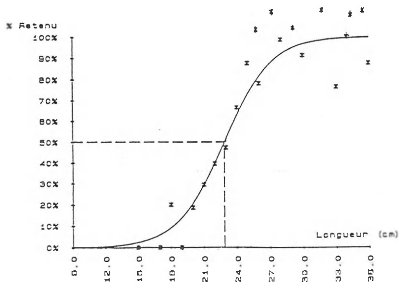
Figure 28 - Courbe de sélectivité de la poche à mailles losanges tracée à partir des données combinées des deux sorties (méthode de chalutage en gréement double).
