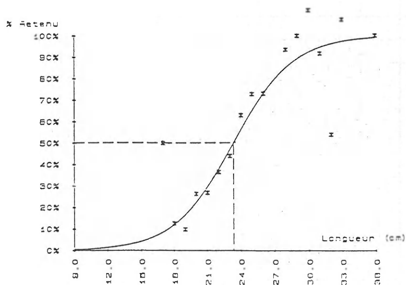
Figure 6 - Courbe de sélectivité tracée à partir des données de la deuxième sortie (poche à mailles carrées à bâbord)
