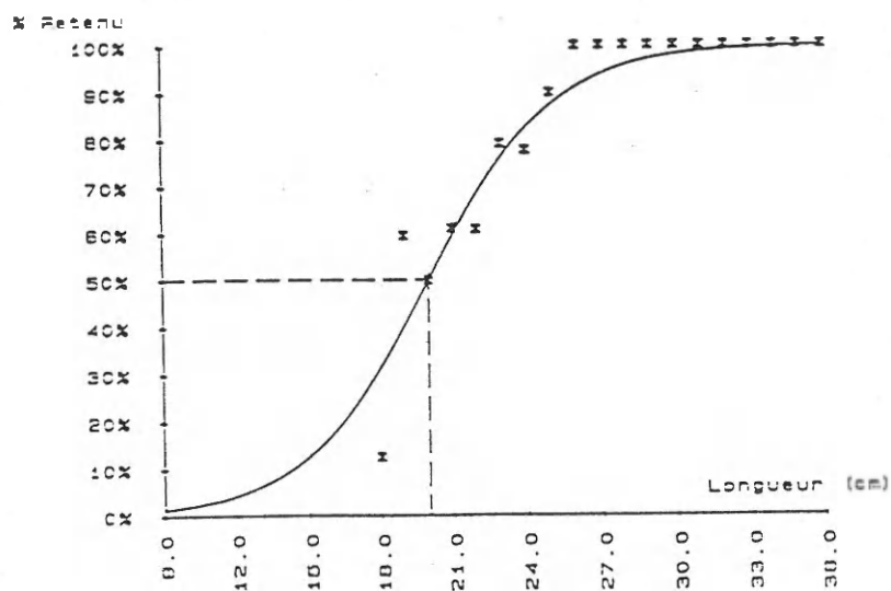
Figure 4 - Courbe de sélectivité tracée à partir des données de la deuxième sortie (poche à mailles losanges à tribord)
