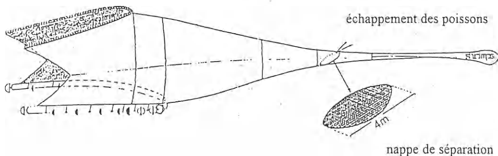
Figure A 2 - Chalut sélectif à crevette avec une nappe de séparation verticale montée au niveau de l'amorce du chalut (d'après LARSEN, 1986).
