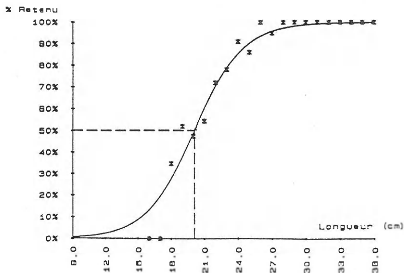
Figure 31 - Courbe de sélectivité de la poche à mailles carrées tracée à partir des données combinées des deux sorties (méthode de la double poche).
