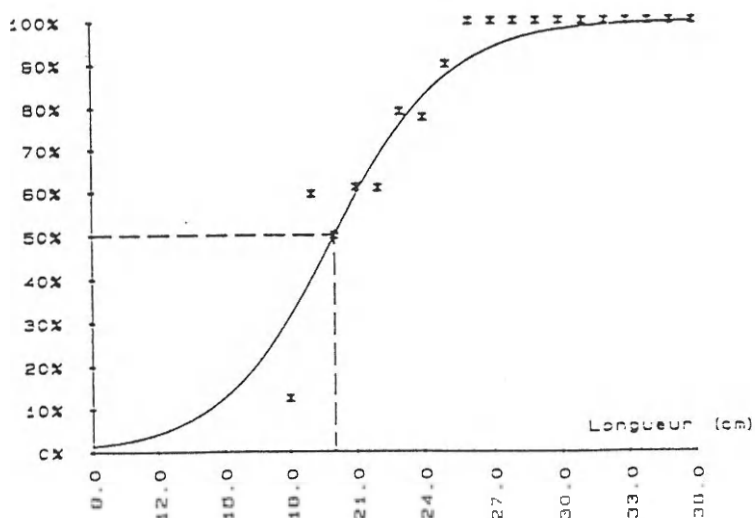
Figure 29 - Courbe de sélectivité de la poche à mailles losanges tracée à partir des données combinées des deux sorties (méthode de la double poche).
