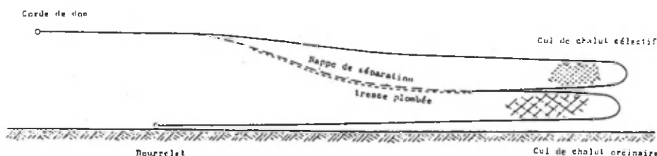
Figure. A 4 - Schéma de la section longitudinale d'un chalut sélectif à crevette avec une nappe de séparation horizontale (d'après VAN DEN BROUCKE et VAN MIDDELEM, 1973).
