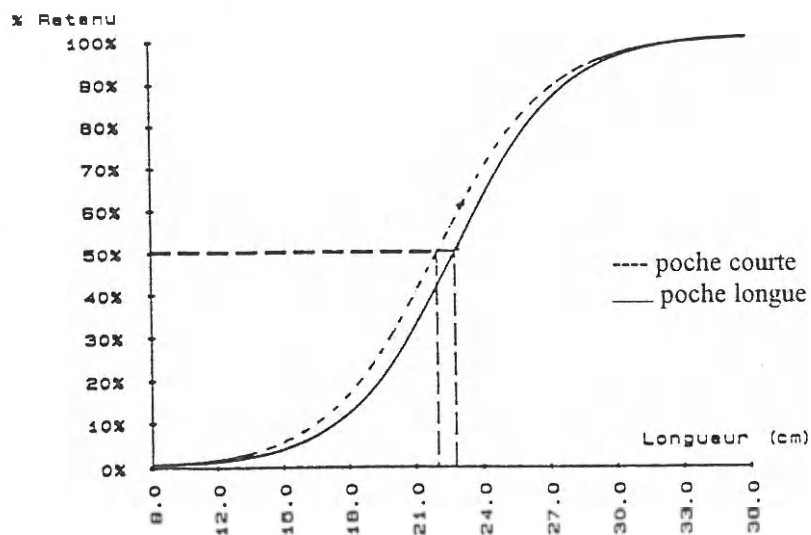
Figure 40 - Comparaison de la courbe de sélectivité de la poche courte à mailles losanges à celle de la poche longue à mailles losanges.
