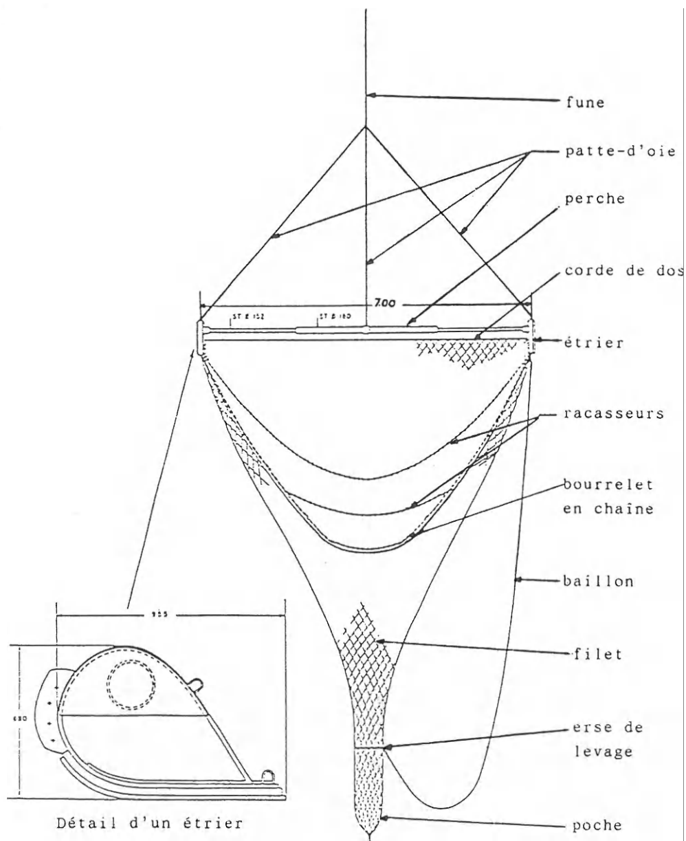
Figure 15 - Chalut à perche utilisé pour la pêche de la sole dans les eaux côtières
