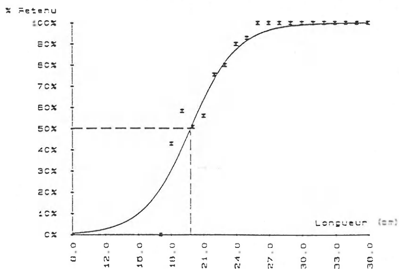
Figure 8 - Courbe de sélectivité tracée à partir des données de la deuxième sortie (poche à mailles carrées à bâbord)
