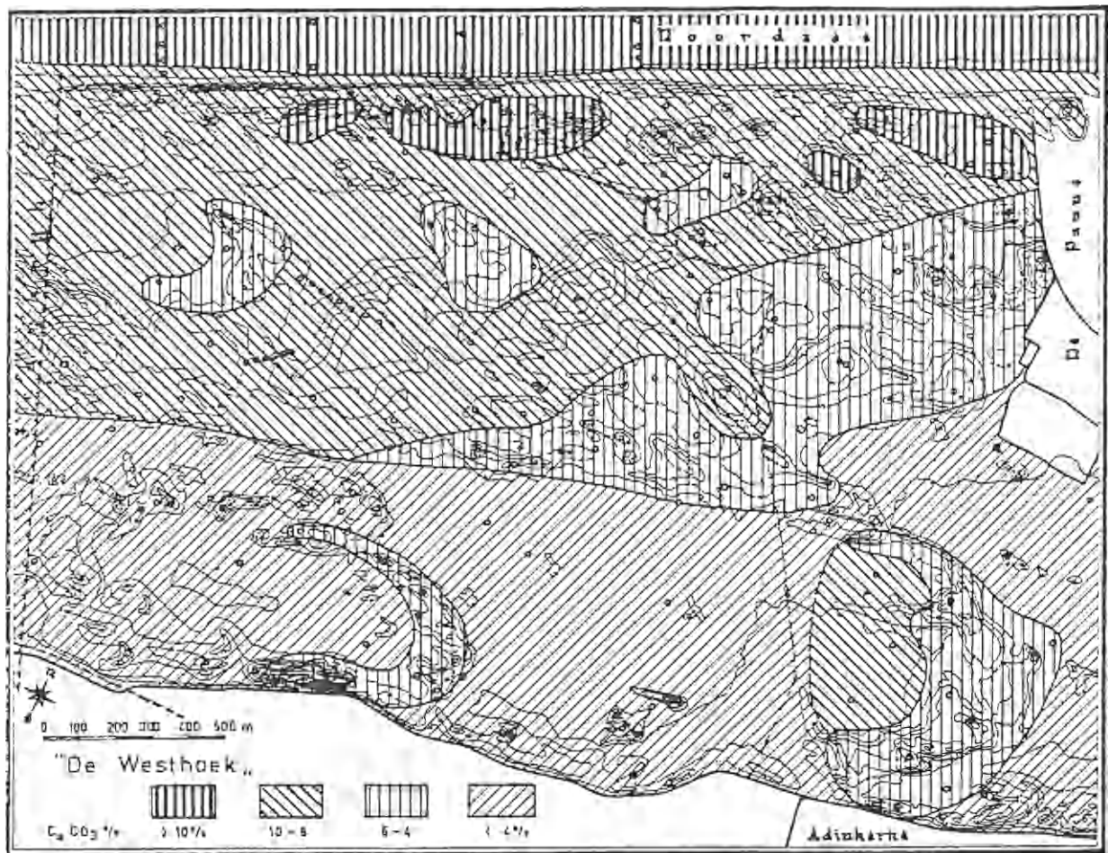
Fig. 8: Kalkgehaltebepaling van de Westhoeksedimenten, die zich voordoen aan het huidig evoluerend oppervlak. (DEPUYDT, 1966).
