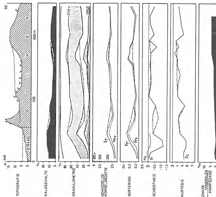
Figuur 2. Detailprofiel doorheen de recente noordgordel van de Westhoek-duinen. Elke parameterwaarde is het gemiddelde voor alle monsters, gebonden aan de respectieve morfologische eenheden. (DEPUYDT, 1972).
