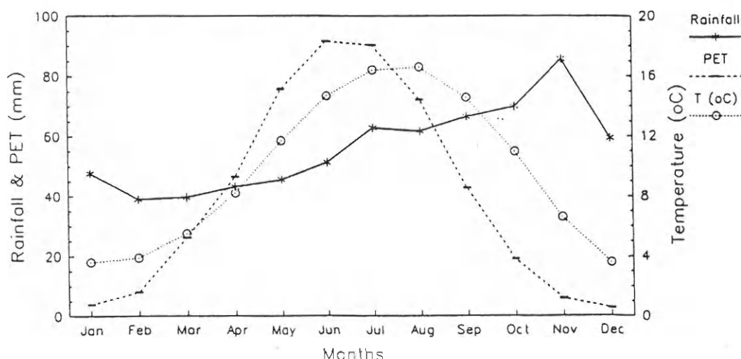
Figuur 3.39: Neerslag en temperatuur en het potentiale evapotranspiratie patroon voor de periode 1957-1976 voor Koksijde. PET werd berekend aan de hand van de Penman methode (KHEDR, 1993 aan de hand van gegevens van LEBBE, 1978)
