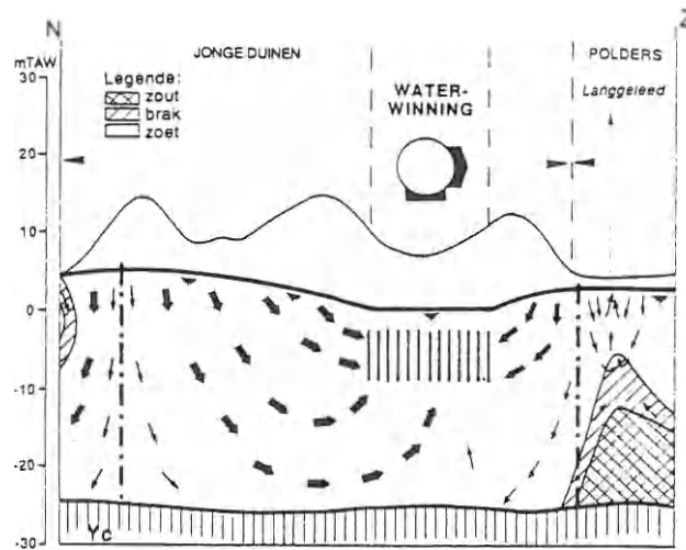
Figuur 3.9: De Jonge Duinen met een waterwinning (LEBBE et al., 1993)
