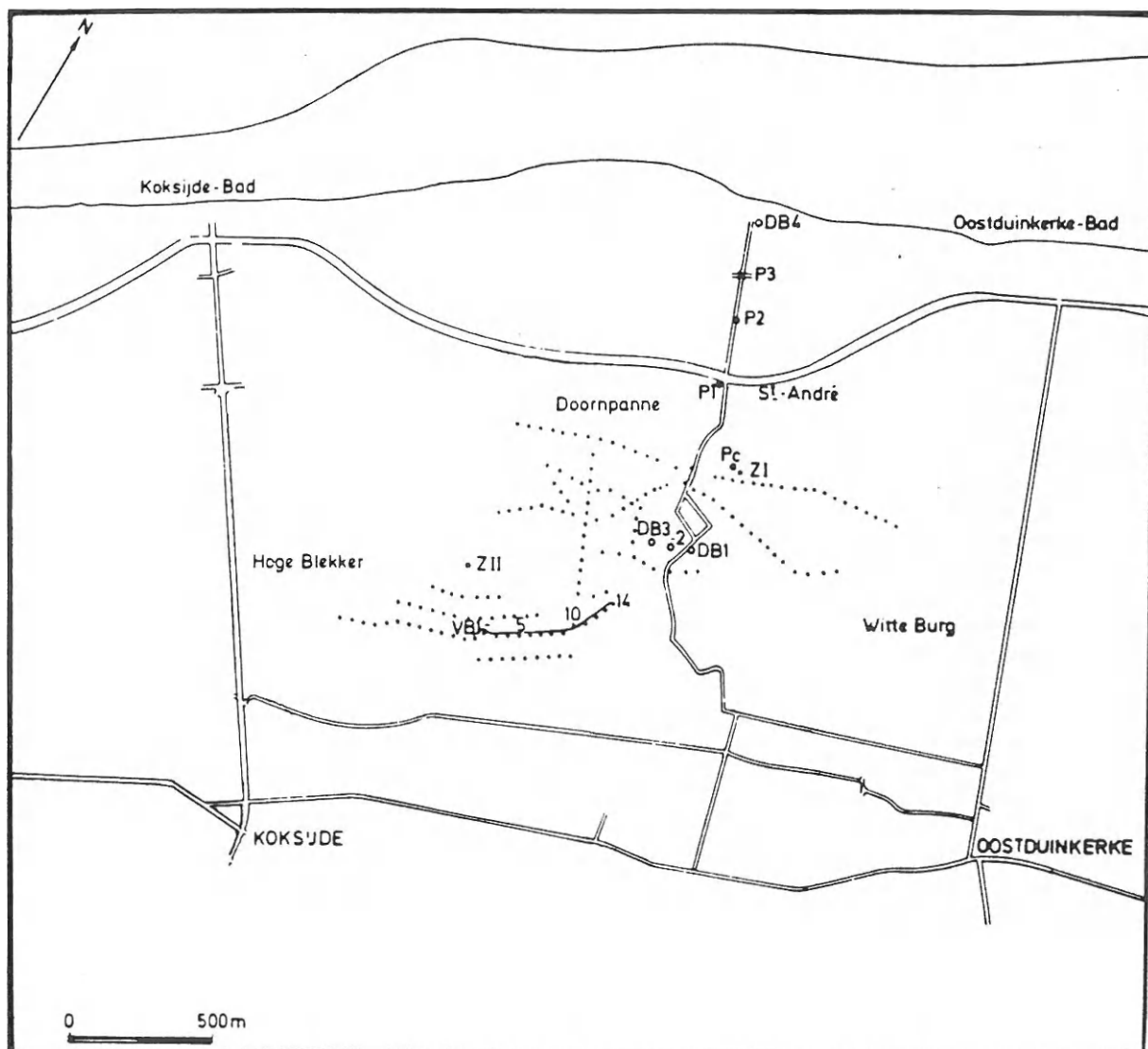
Figuur 2.6: Ligging van de boringen en profielen in het duingebied tussen Koksijde en Oostduinkerke (LEBBE & DE BREUCK, 1980)
