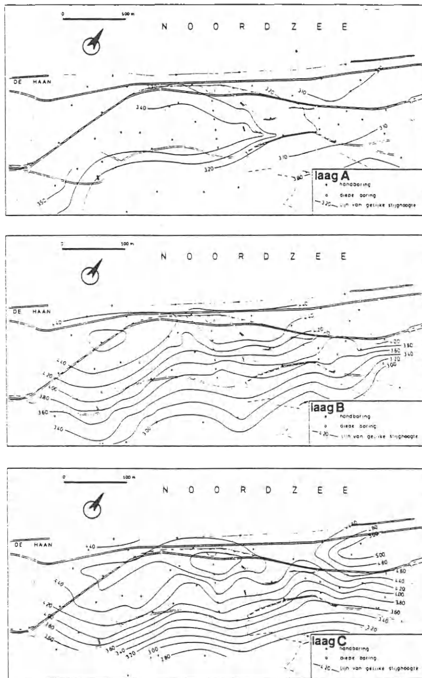
Figuur 3.24: Waargenomen gemiddelde stijghoogteconfiguratie (1980 - 1983) in de doorlatende lagen A, B en C in duingebied ten oosten van De Haan (DEVOS, 1984)
