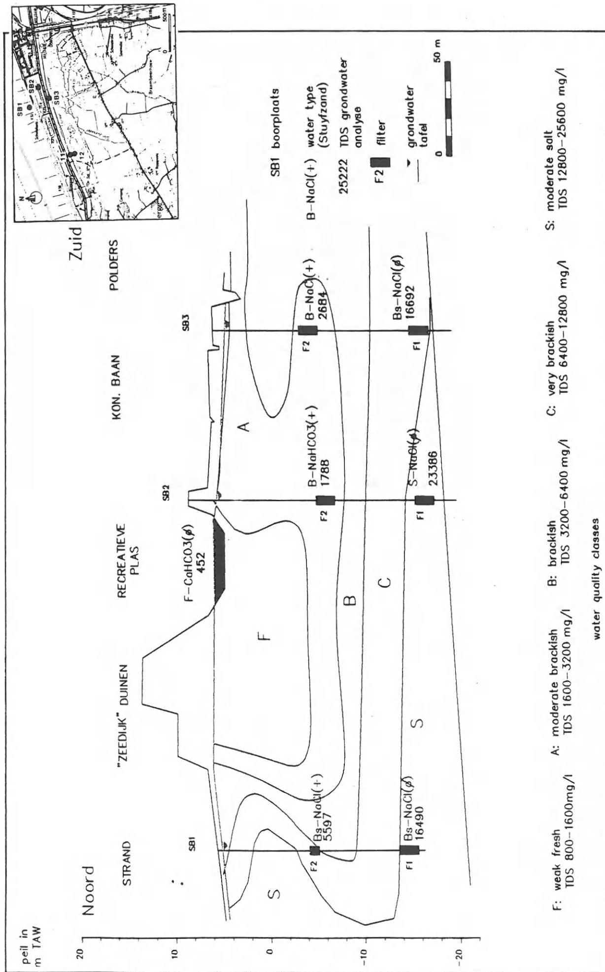
Figuur 3.36: Resultaten grond- en oppervlakteanalyse voor het natuurgebied "de Fonteyntjes" in Blankenberge (VERMOORTELT & DE BREUCK, 1994)
