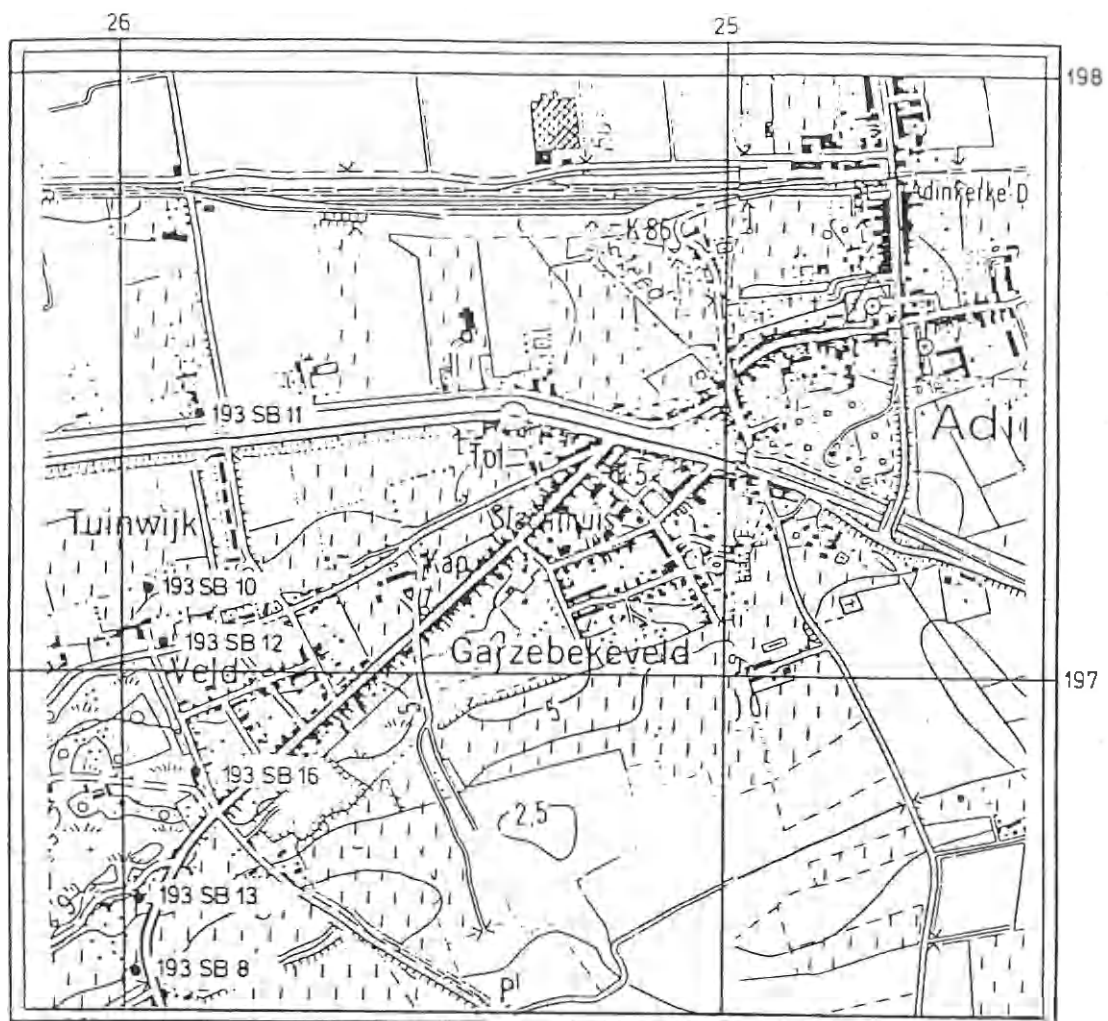
Figuur 3.14: Ligging van de verschillende peilbuizen in Adinkerke (BOLLE, 1983)
