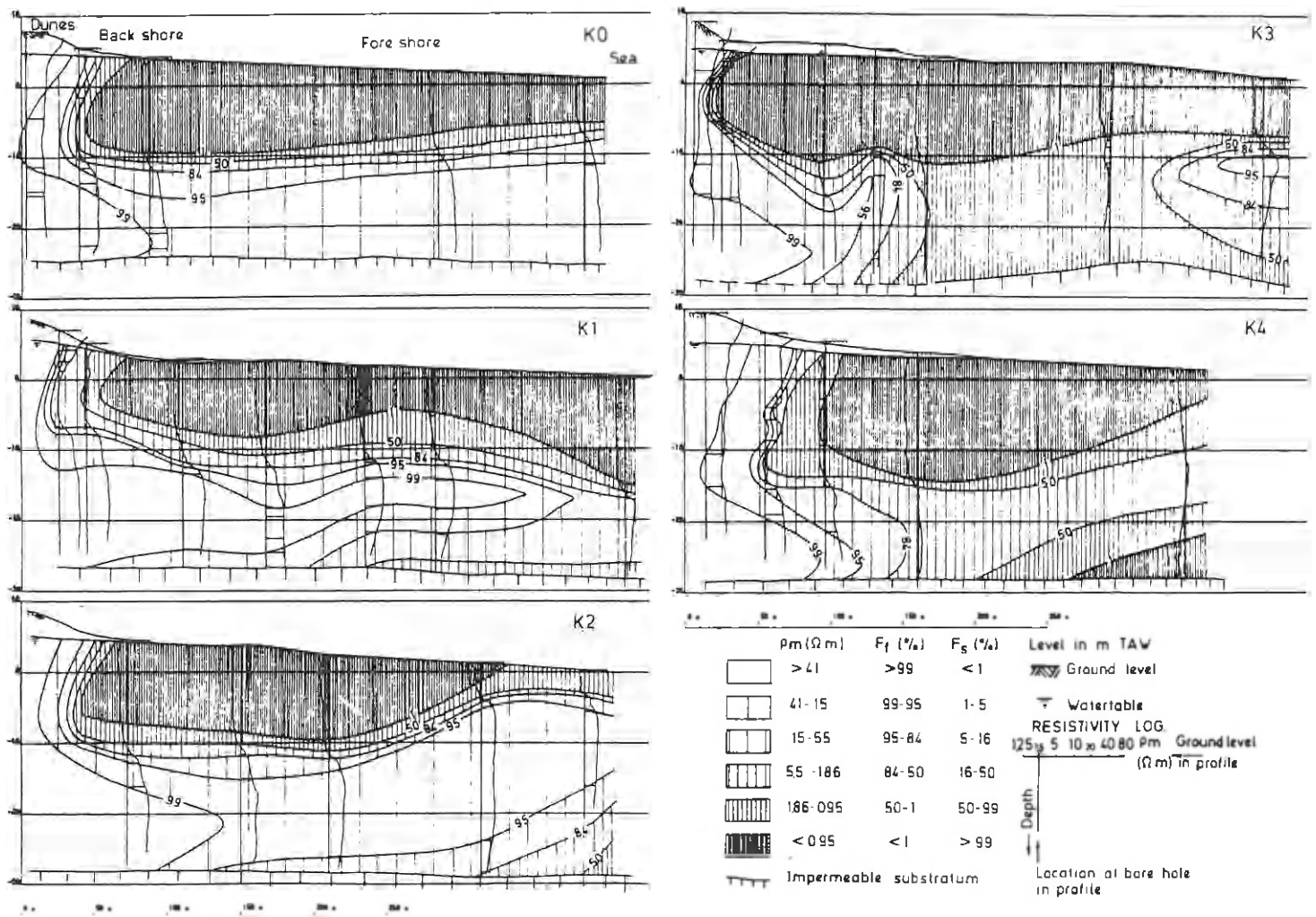
Figuur 3.29a: Profielen van zoetwaterpercentage in De Panne (LEBBE, 1984)
