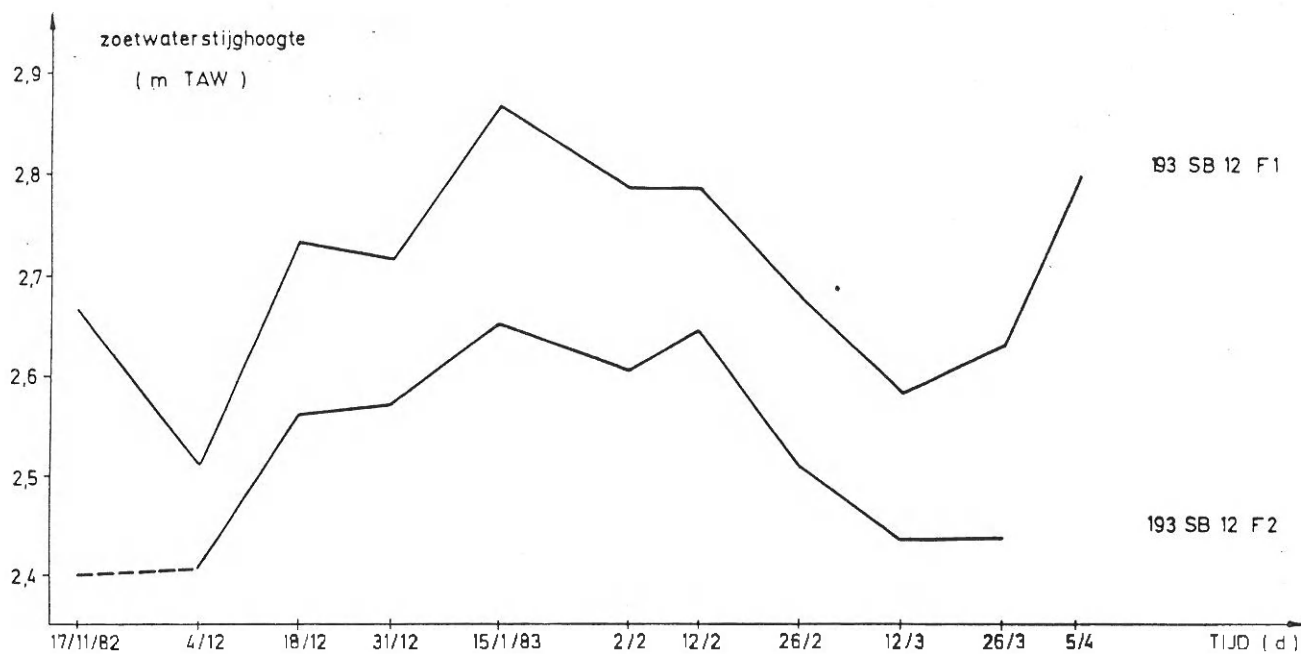
Figuur 3.18: Zoetwaterstijghoogte bij 193SB12F1, F2 (BOLLE, 1983)
