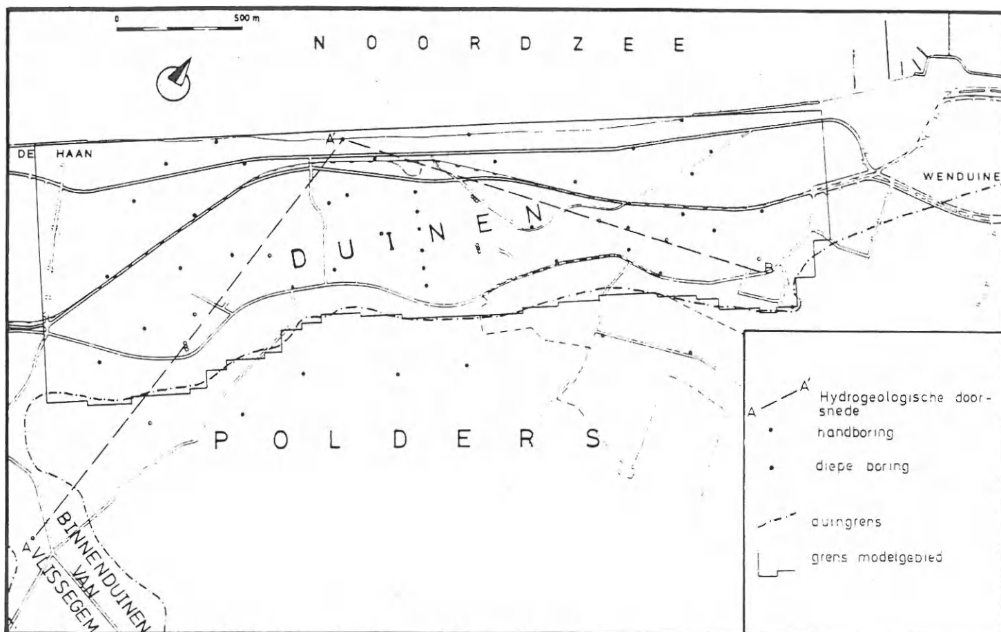
Figuur 2.18: Ligging van de twee profielen in het duingebied ten oosten van De Haan (DEVOS, 1984)
