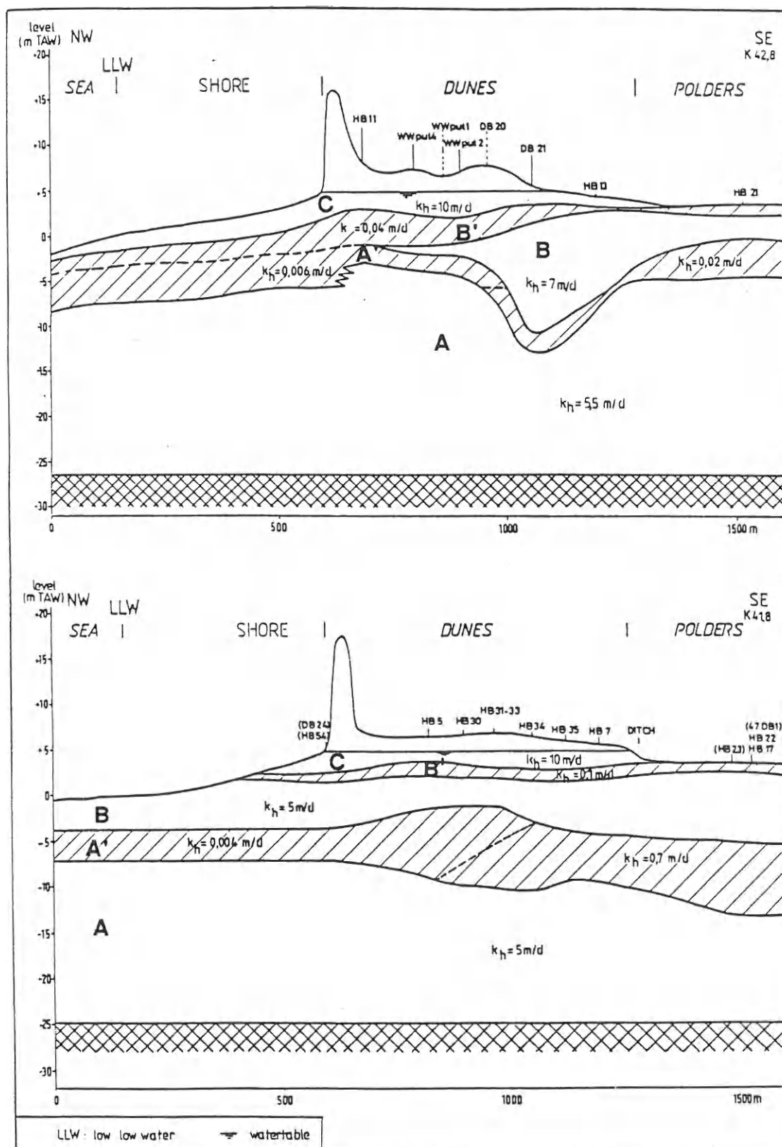
Figuur 3.3: Verdeling van de doorlatende en slecht doorlatende lagen in K41,8 en K42,8 in het duingebied ten oosten van De Haan (WALRAEVENS et al., 1990)
