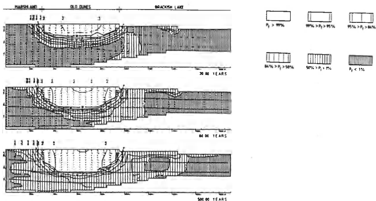
Figuur 3.30: De Oude Duinen onder natuurlijke omstandigheden (LEBBE & PEDE, 1986)
