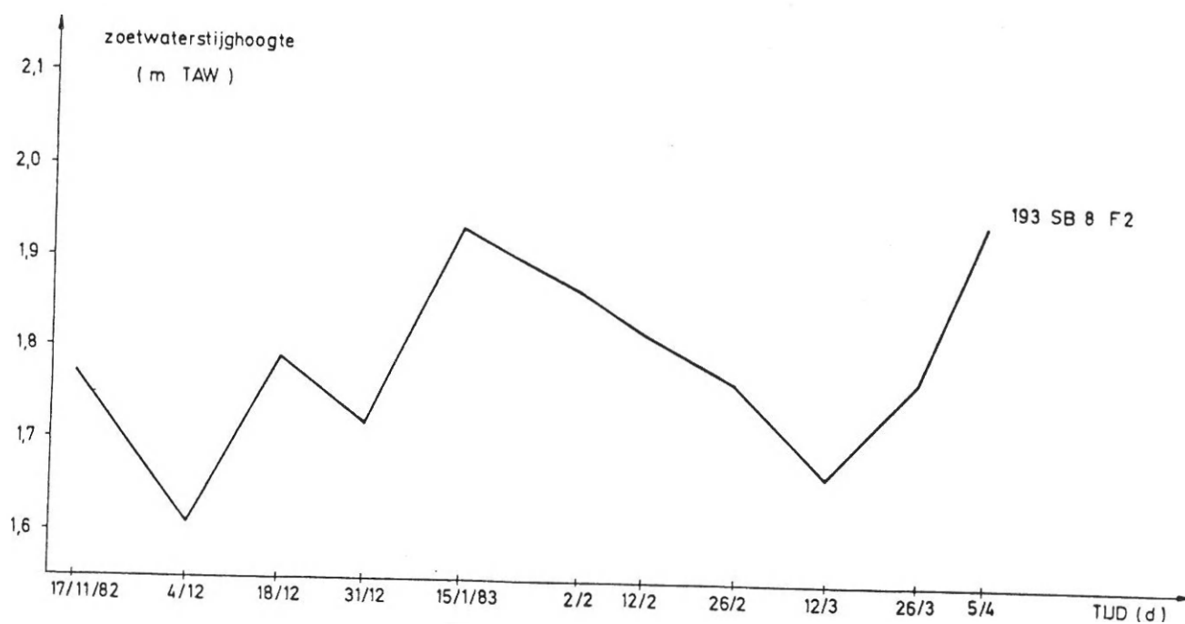
Figuur 3.15: Zoetwaterstijghoogte bij 193SB8F2 (BOLLE, 1983)
