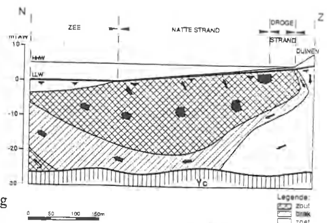
Figuur 3.5: Het strand met verminderde grondwaterstroming (LEBBE et al., 1993)
