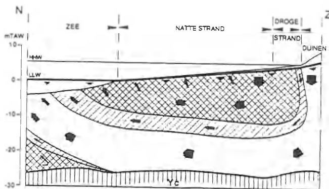
Figuur 3.4: Het strand met natuurlijke grondwaterstroming (LEBBE et al., 1993)
