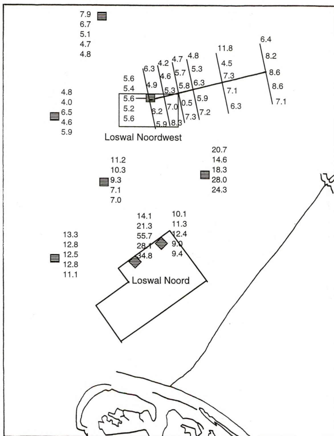
Fig. 3: Slibgehalten (totale fraktie <16 µm, %) van het sediment op en rond Loswal Noord en Loswal Noordwest.
