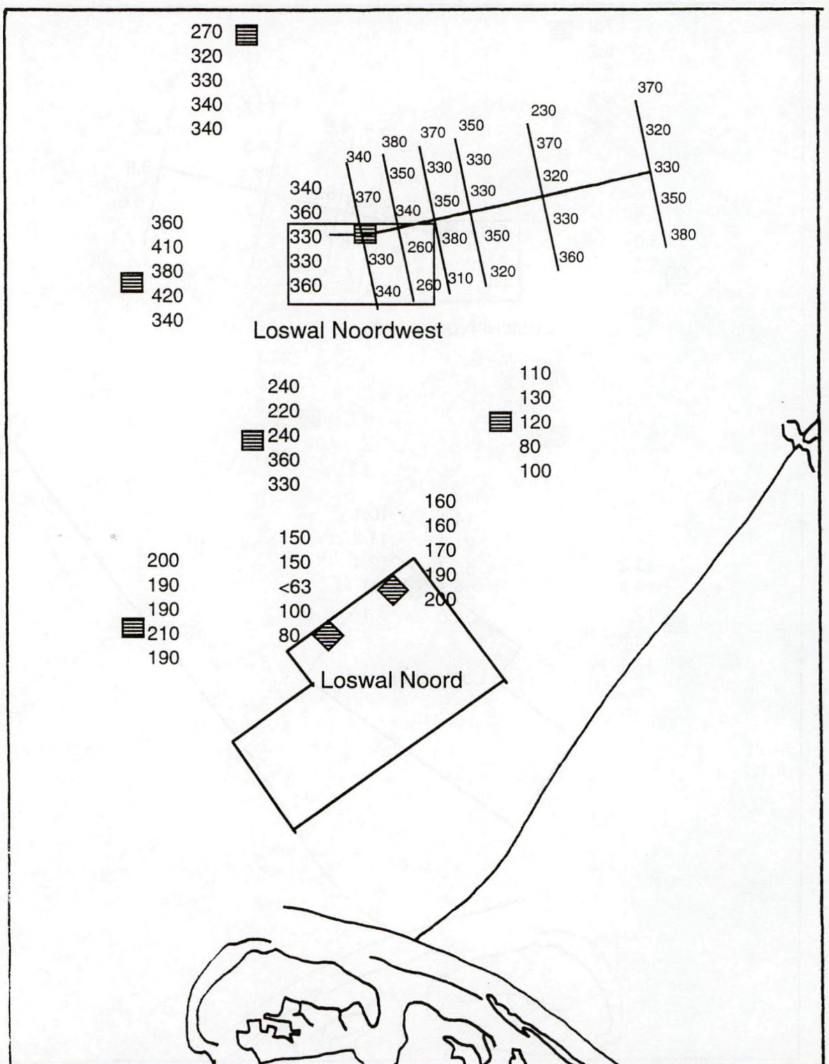
Fig. 4: Mediane korrelgrootte ( \mu\text{m} ) van het sediment (inclusief de slibfractie) op en rond Loswal Noord en Loswal Noordwest.
