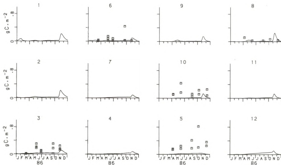
Fig. 3.20. Gesimuleerde (—) en gemeten (□) biomassa aan macroepibenthos in het sublittoraal (UMAC, \text{gC} \cdot \text{m}^{-2} ). Let op onderlinge verschillen in schaal.
