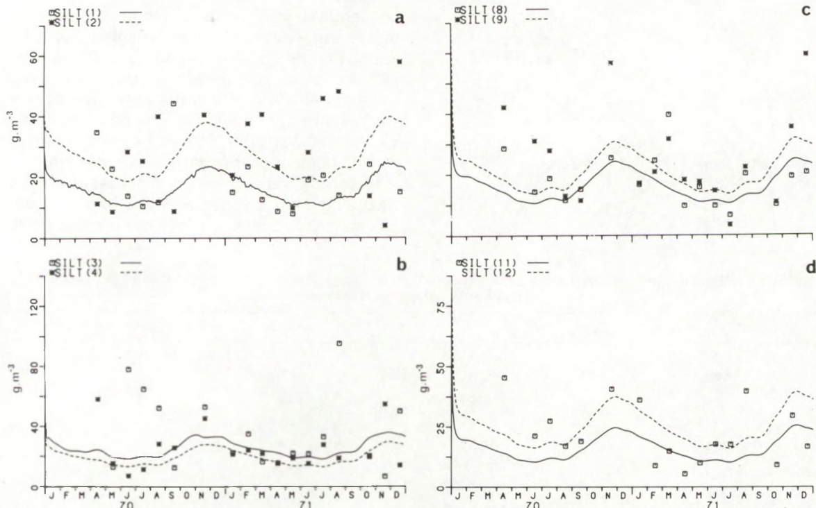
Fig. 2.17. Simulatie waarnemingen van de hoeveelheid gesuspendeerd materiaal, M, vergeleken met veldwaarnemingen in de periode 1970-1971. a. compartiment 1 en 2; b. compartiment 3 en 4; c. compartiment 8 en 9; d. compartiment 11 en 12.
