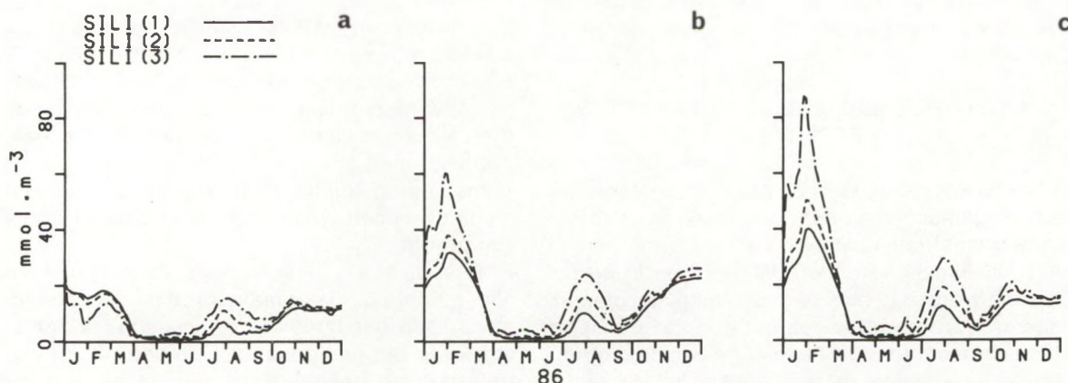
Fig. 4.4. Seizoensverloop van de concentratie opgelost reactief silicaat (SILI; mmol·m -3 ) in de compartimenten 1, 2 en 3 gesimuleerd met een P-, Si-belasting vanuit het IJsselmeer, die gelijk is aan: a) 0; b) de standaardwaarde; en c) 1.5 keer zo groot als de standaardwaarde.
