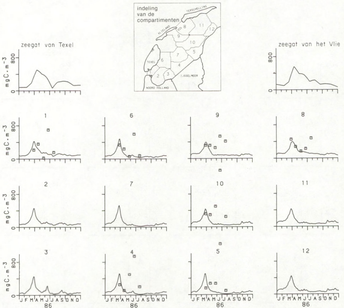
Fig. 3.11. Gesimuleerde (—) en gemeten (□) waarden voor de biomassa aan pelagische diatomeeën (PDIA, \text{mg C} \cdot \text{m}^{-3} ).
