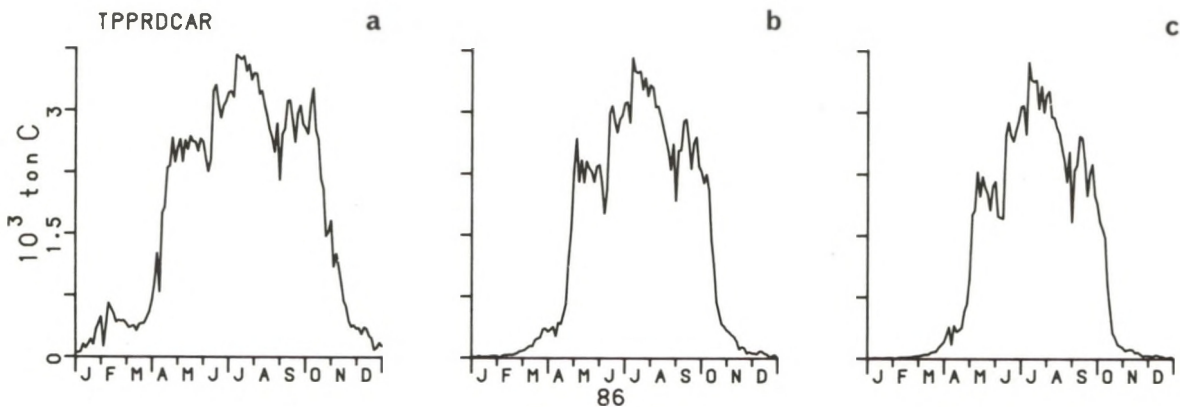
Fig. 4.1. De totale primaire produktie in de westelijke Waddenzee (TPPRDCAR; 10^3 ton C) gesimuleerd met a) ZZSIL = 0 ; b) ZZSIL = 40 \cdot 10^{-6} \text{ m}^2 \cdot \text{mg}^{-1} (de standaard situatie) en c) ZZSIL = 80 \cdot 10^{-6} \text{ m}^2 \cdot \text{mg}^{-1} .
