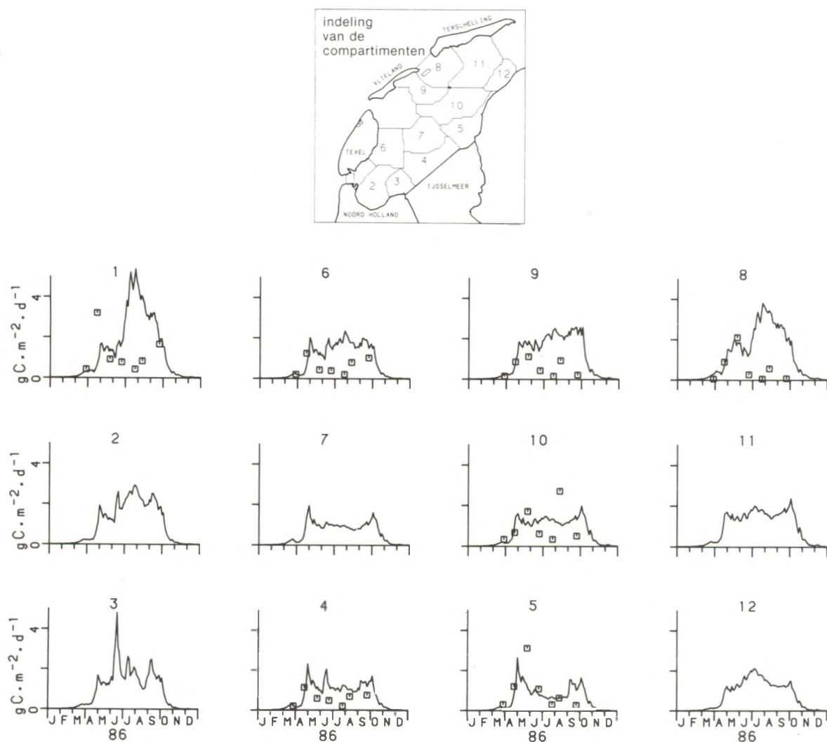
Fig. 3.12. Gesimuleerde (—) en gemeten (□) waarden voor de totale pelagische primaire produktie (MPPP, gC·m -2 ·dag -1 ).
