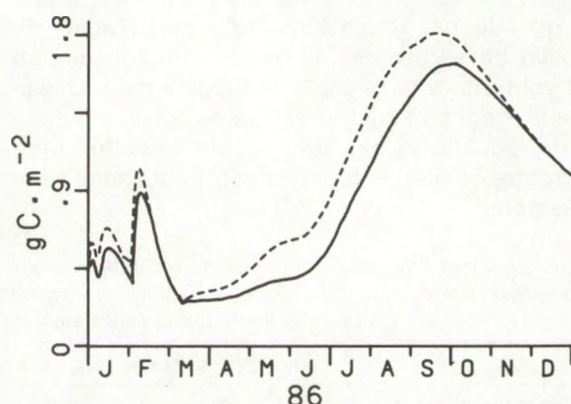
Fig. 4.12. Biomassaverloop van de epibenthische predatoren in het sublitoraal, UMAC, (—) in het gemodificeerde model (BARETTA & RUARDIJ, 1988a) met verhoogde startwaarden voor USF; ter vergelijking het biomassaverloop van USF (---) in het gemodificeerde model zonder verhoogde startwaarden voor USF. Eenheid \text{gC} \cdot \text{m}^{-2} .
