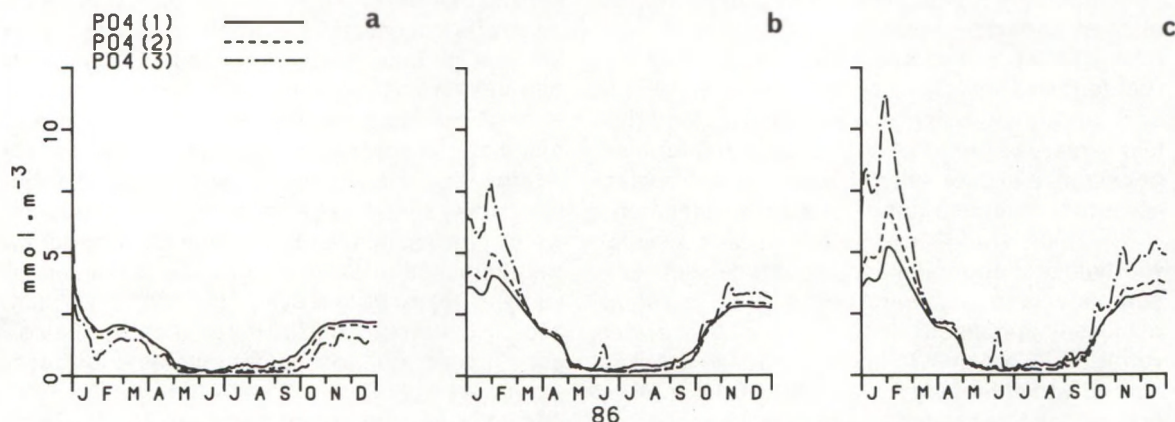
Fig. 4.3. Seizoensverloop van de concentratie opgelost reactief fosfaat (PO 4 ; mmol·m -3 ) in de compartimenten 1, 2 en 3 gesimuleerd met een P-, Si-belasting vanuit het IJsselmeer, die gelijk is aan: a) 0; b) de standaardwaarde; en c) 1.5 keer zo groot als de standaardwaarde.
