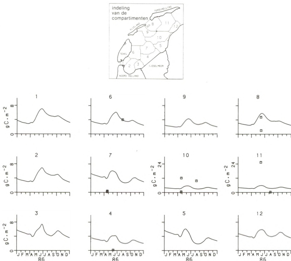
Fig. 3.18. Gesimuleerde (—) en gemeten (□) biomassa aan macrobenthische "suspension feeders" in het litoraal (BSF, mgC \cdot m^{-2} ). Let op onderlinge verschillen in schaal.
