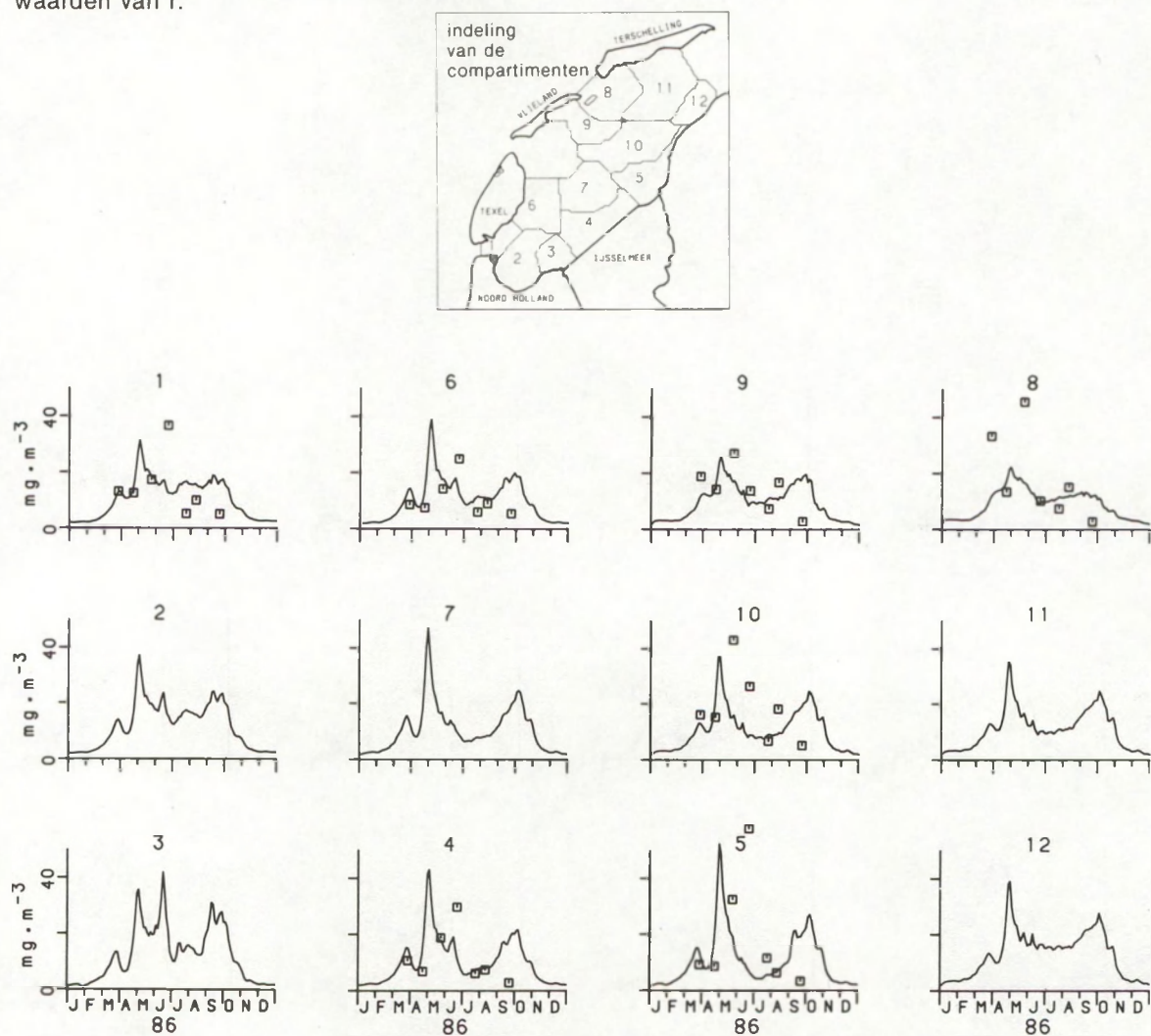
Fig. 3.9. Gesimuleerde (—) en gemeten (□) waarden voor de concentraties aan chlorofyl-a (CHLA, mg · m -3 ).
