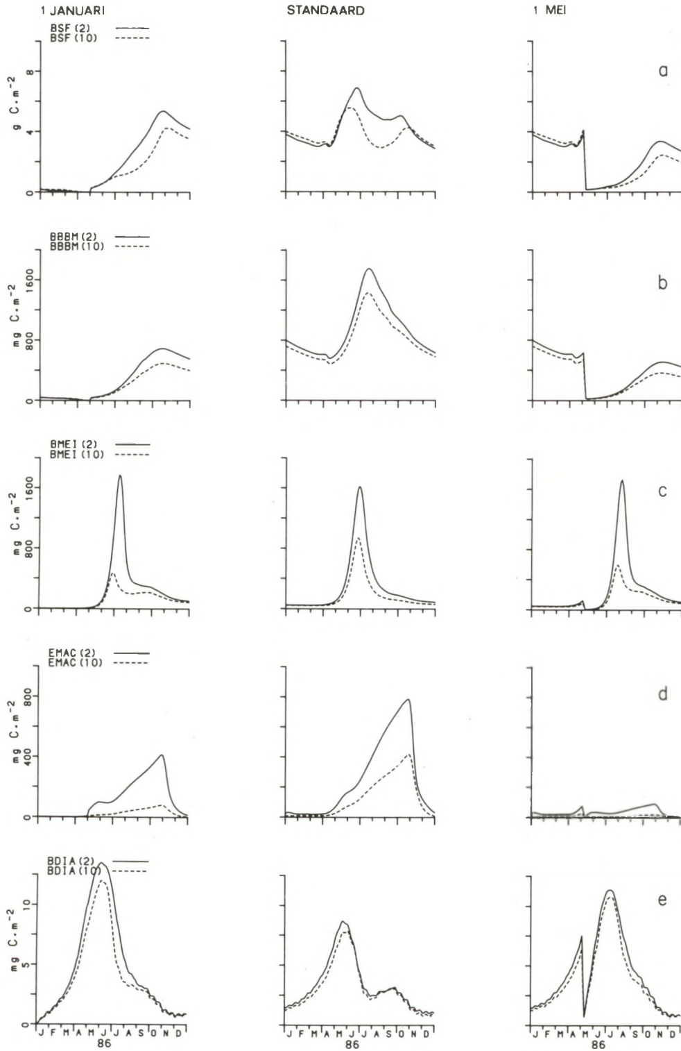
Fig. 4.13. Biomassverloop op de getijdenplaten in de compartimenten 2 en 10 van a) benthische suspension feeders; b) deposit feeders; c) meiobenthos; d) epibenthische predatoren; e) benthische diatomeeën gesimuleerd met een reductie van het (epi)benthisch systeem met 95% op 1 januari (links), in de standaard situatie (midden) en na reductie op 1 mei (rechts).
