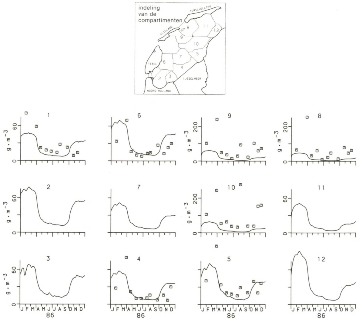
Fig. 3.3. Gesimuleerde (—) en gemeten ( \square ) gehalten aan gesuspendeerd materiaal (SUSM, \text{mg} \cdot \text{m}^{-3} ). Let op onderlinge verschillen in schaal.
