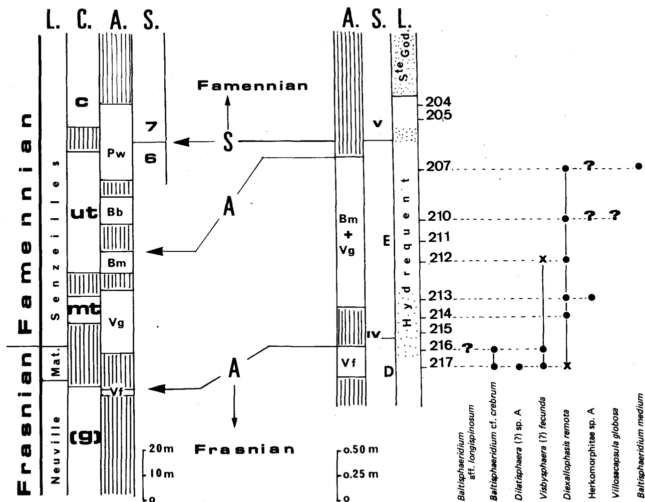
Figure 2.- Comparaison entre l'Ardenne et le Boulonnais à la transition Frasnien-Famennien.
