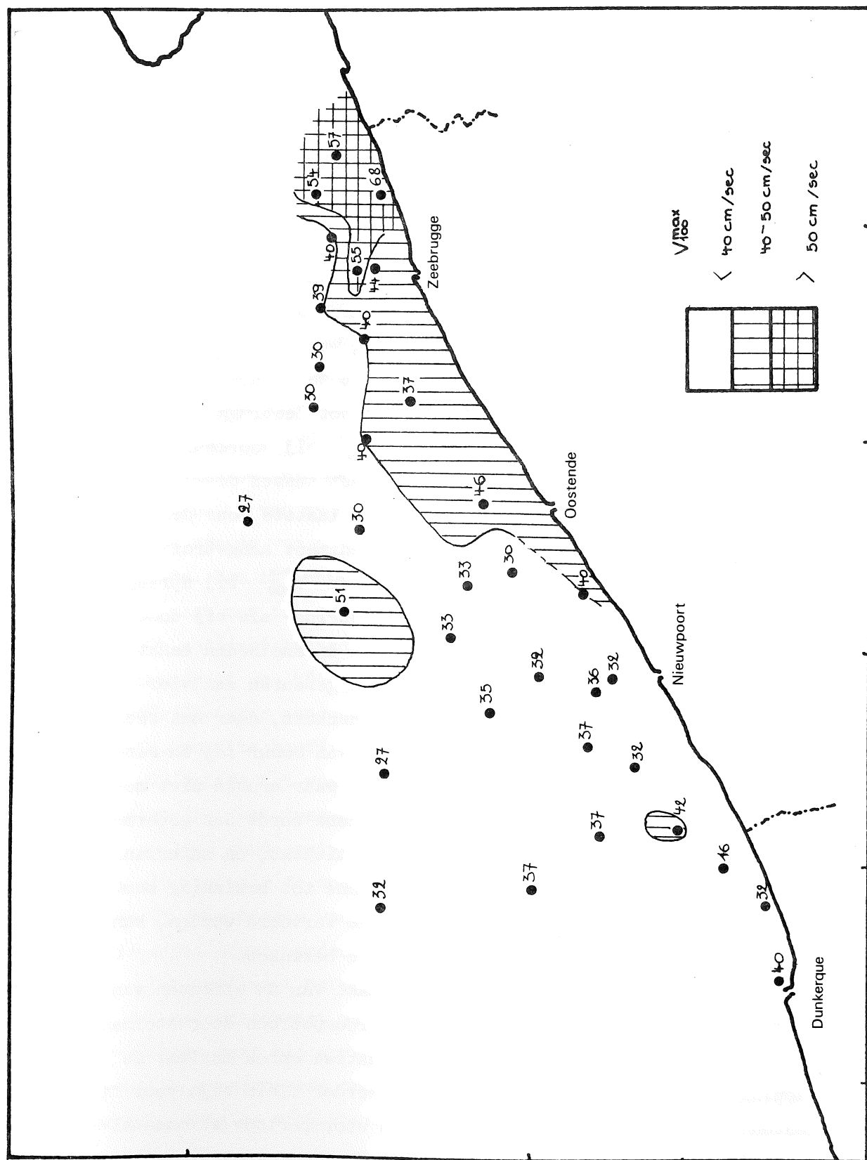
fig. 42. Verdeling van de V_{100}^{max} bij doortij (maximumsnelheid op 1 m van de bodem)
