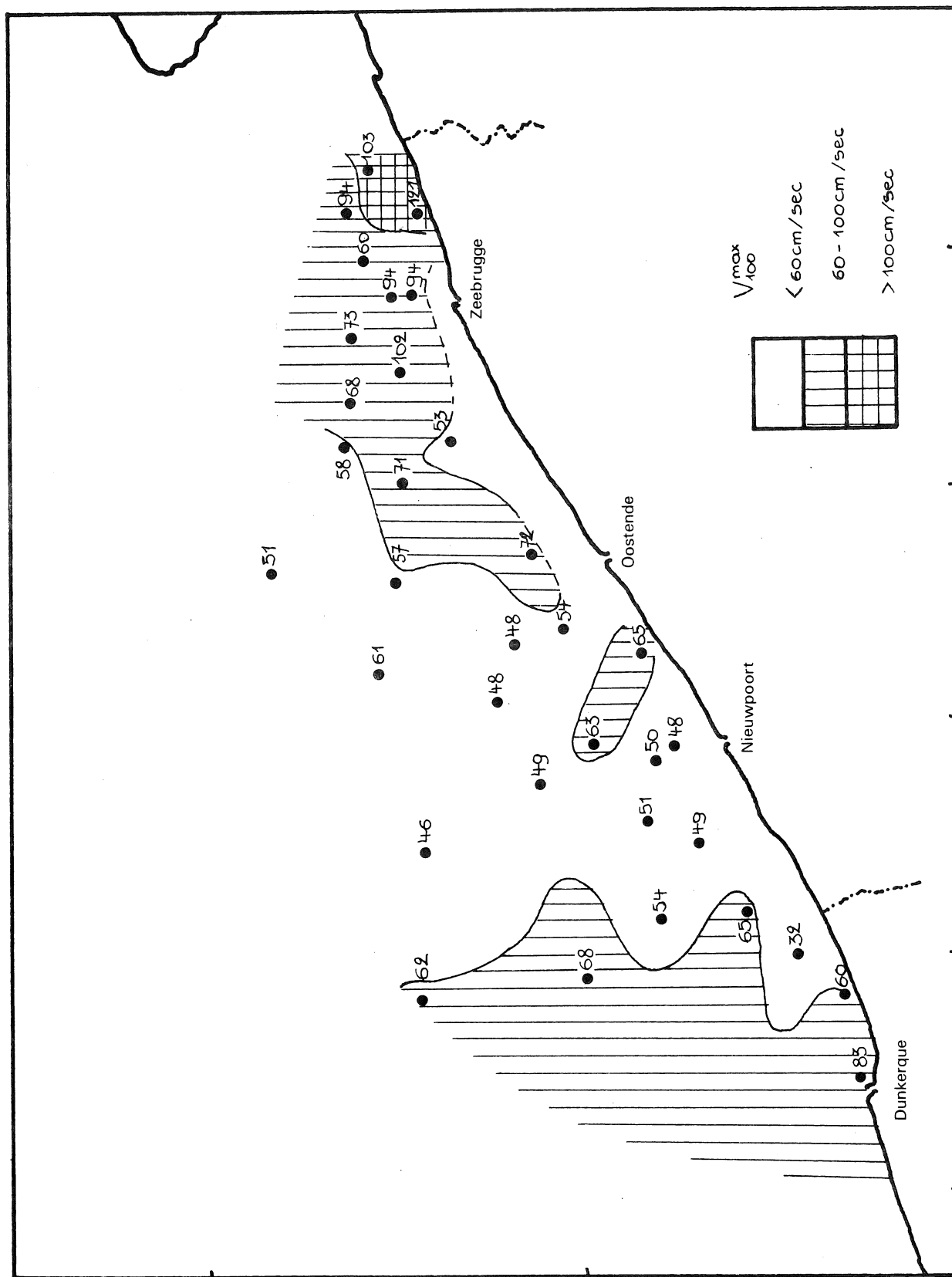
fig. 41. Verdeling van de V_{100}^{\max} bij springtij (maximumsnelheid op 1 m van de bodem)
