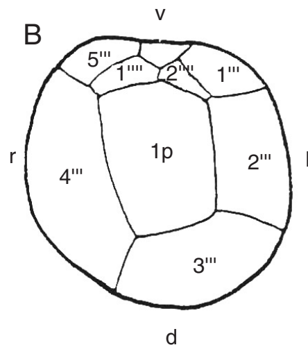
Fig. 13. Tabulation chez Gambierdiscus . A: épithèque, B: hypothèque, d: dorsal, v: ventral, l: gauche, r: droite. (tiré de Fukuyo 1981).
