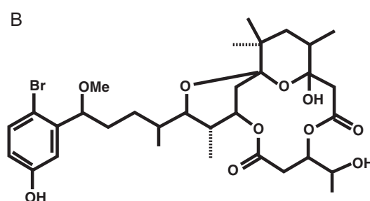
Fig. 27. Structure de la Lyngbyatoxine A (A) et de l'aplysiatoxine (B) (redessiné de Sivonen 1996).
