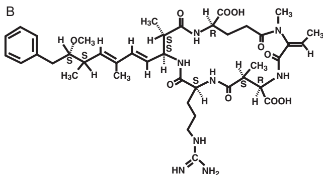
Fig. 24. Structure générale des microcystines (A) et nodularines (B) (redessiné de Sivonen 1996, Carmichael 1995).
