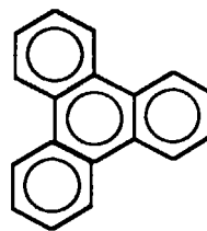
Triphenylene 217-59-4
