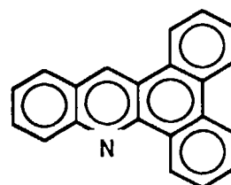
Dibenz[a,c]- acridine 215-62-3
