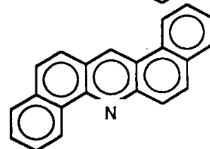
Dibenz[a,h]- acridine 226-92-6
