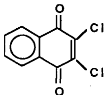
Dichlone 117-65-6
