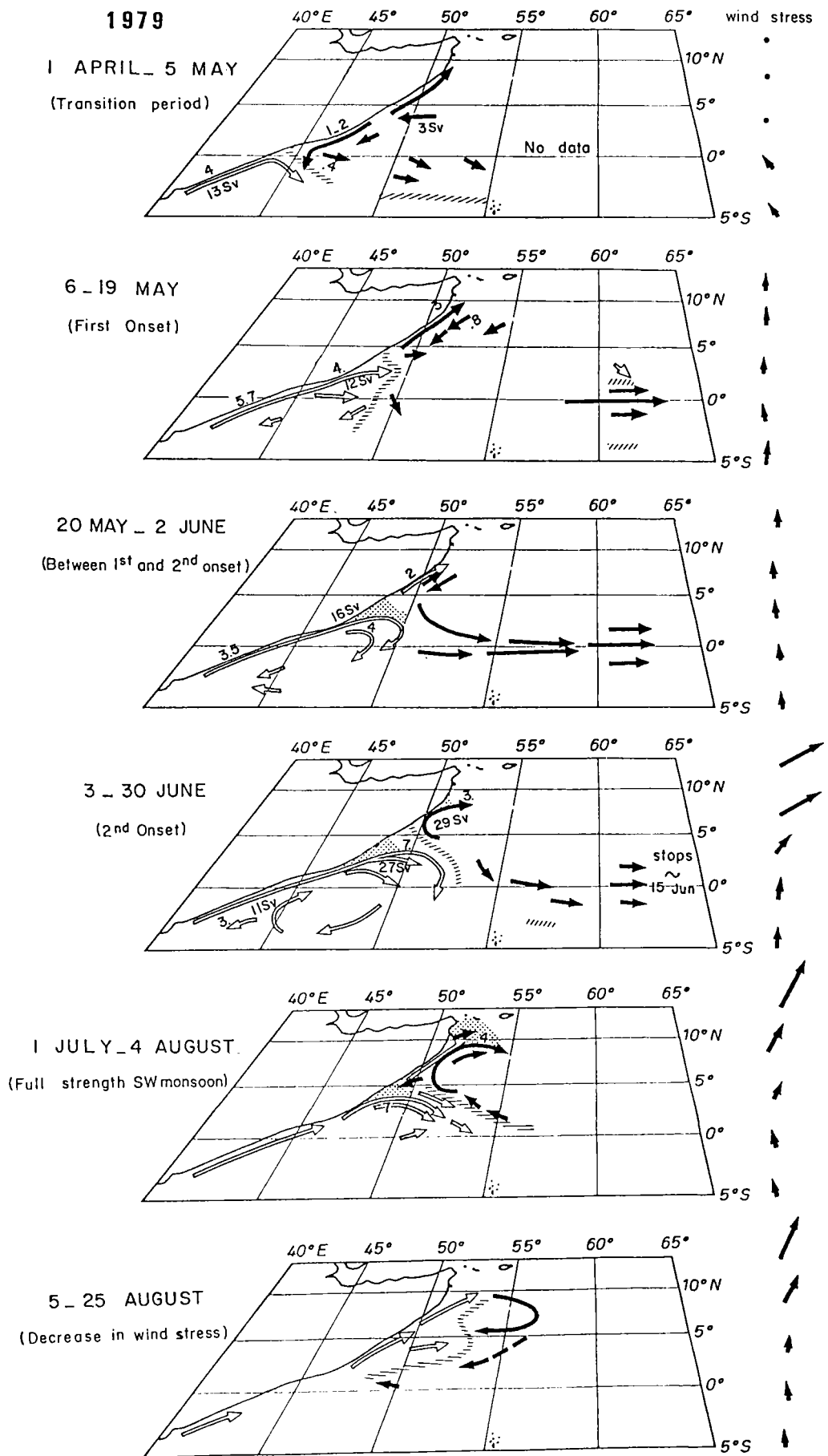
FIGURE 3 - Evolution de la circulation de surface d'après les observations de 1979 (vitesse en noeuds , flux en Sv=10^6 m^3 s^{-1} , \Rightarrow = salinités basses, \rightarrow = salinités élevées, --- = fronts, \square = upwellings).
