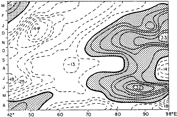
FIGURE 8 - Cycle saisonnier de la profondeur de l'isotherme 25°C à l'équateur dans l'océan Indien, en mètres ( +65m ). (G.REVERDIN)
