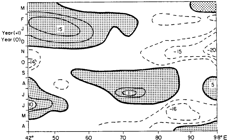
FIGURE 9 - Anomalies de l'isotherme 25°C, en mètres, à l'équateur pour une année El Nino composite ( 1957,1965,1969,1972 et 1976 ). (G.REVERDIN)
