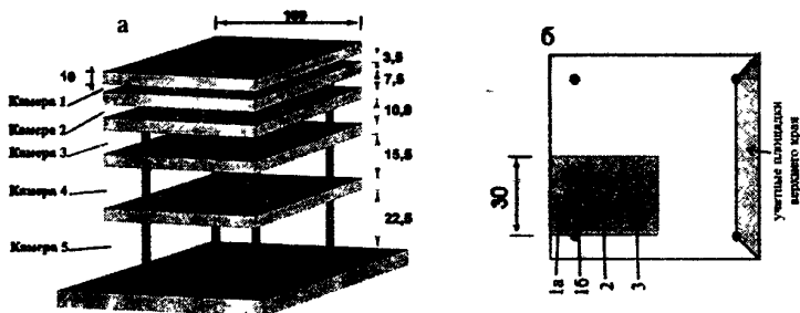
Рис. 3. Схема экспериментальной конструкции искусственный риф БИМЛЭМ (а); схема учетных площадок на плитах рифа (б). Все размеры даны в сантиметрах.
