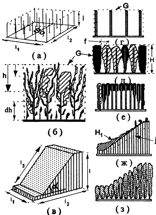
Рис.9. Схемы двух типов экспериментальных конструкций (модулей) для фитообращения со стержневыми структурными элементами с одинаковой (а) и разной длиной (в, модуль - "склон"). (б, ж, з) - стержневые структуры, обросшие многоклеточными и (г-е) - диатомовыми водорослями при разной плотности расположения структур в модуле ( N/S_0 : 0.054 (б, г); 0.188 (ж, з); 0.284 (д) и 1.068 (е) экз./см 2 ). l - длина стержневой структуры; l_1, l_2 и S_0 - линейные размеры и поверхность "дна" модуля; l_3 - длина поверхности склона модуля, проходящего по верхушкам опорных структур и угол ( \alpha = 35^\circ ) наклон этой
