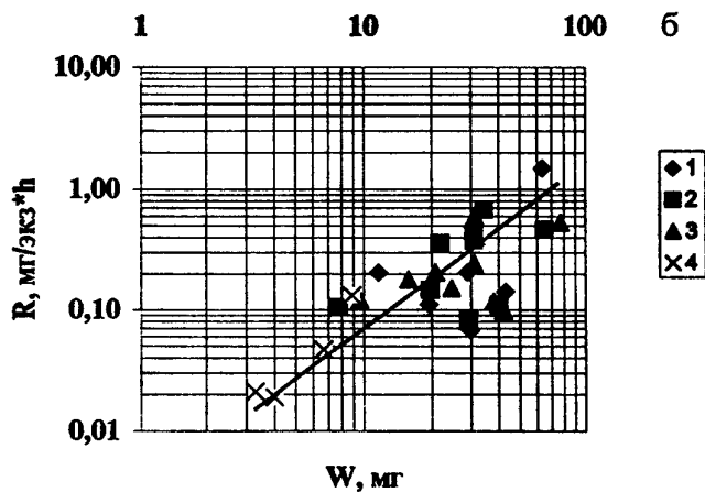
Рис. 60. Зависимость скорости дыхания молодежи кефали и атерины от сухой массы тела: а - переменная величина концентрации массы в опытах, б - концентрация массы есть величина постоянная ( C_0=100 \text{ мг}\cdot\text{л}^{-1} ). 1- 4 - тоже, что и на рис.59.
