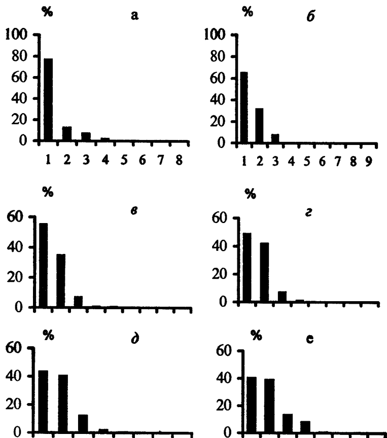
Рис. 55. Убывание разнообразия эпифитона в бухте Омега по таксонам (% обилия, а,б - Дача, в,г - Маяк, д,е - Пирс 1990, 1991 гг.).
