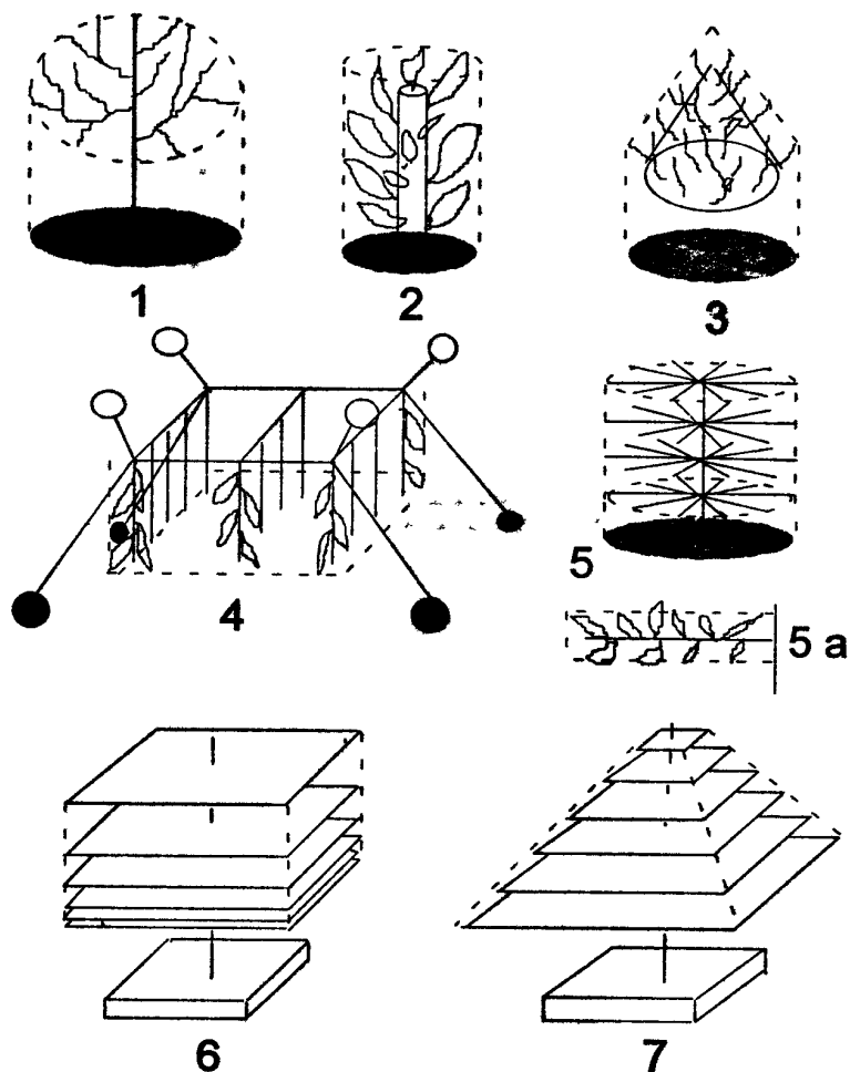
Рис. 1. Схема экспериментальных модулей для фитообрастания с пластинчатыми (NN 6,7), стержневыми (NN 5-7) и конусообразными (NN 8-12) структурными элементами, а также модулей камерного типа для зоообрастания (NN 13-16) Подробно в тексте.
