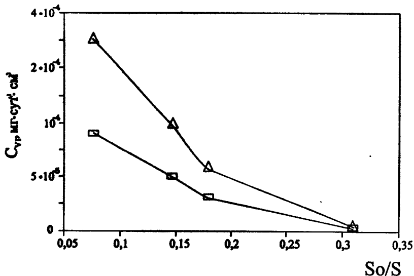
Рис. 8. Зависимость потребления спирорбисами растворенного органического вещества в расчете на единицу объема ( C_v ) от параметра So/S камер рифа: ( \Delta ) – гидролизат цистозины, ( \square ) – бикарбонат.
