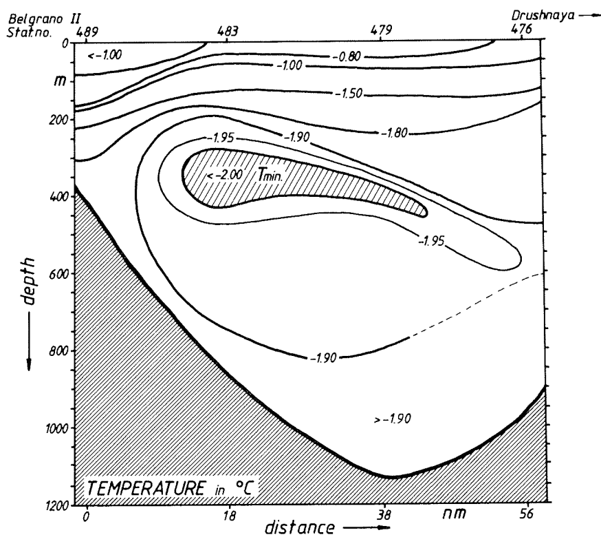
Abb. 3: Temperaturschnitte aus den unvollständig korrigierten (d.h. keine Skalengkorrektur !) Umkippthermometermessungen.
