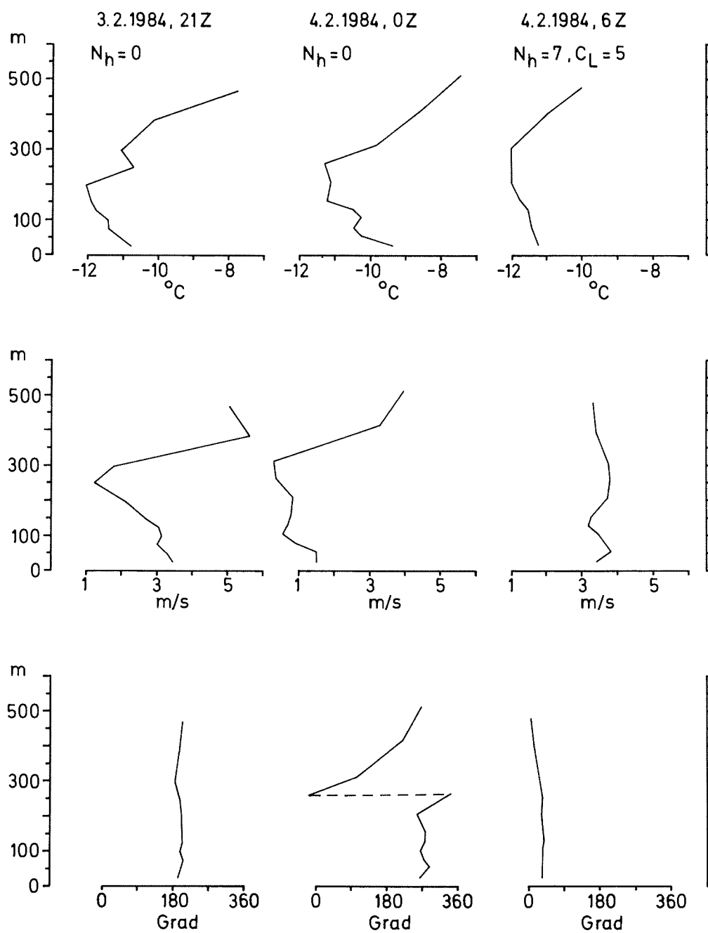
Abbildung 4: Vertikalprofile der Lufttemperatur, der Windgeschwindigkeit und der Windrichtung aus Fesselsondenaufstiegen von Bord der "Polarstern" aus während der 3. MEFIS-Intensivmeßphase. ( N_h Bedeckungsgrad, C_L Wolkentyp der niedrigen Wolken.)
