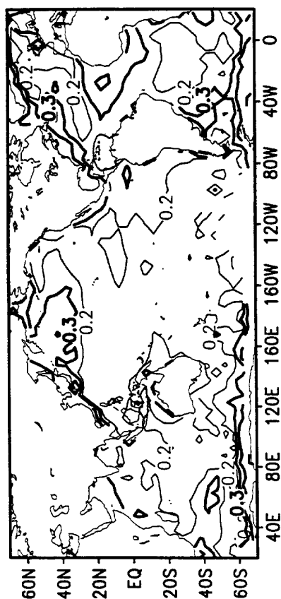
NRL SST Anomaly (°C)
