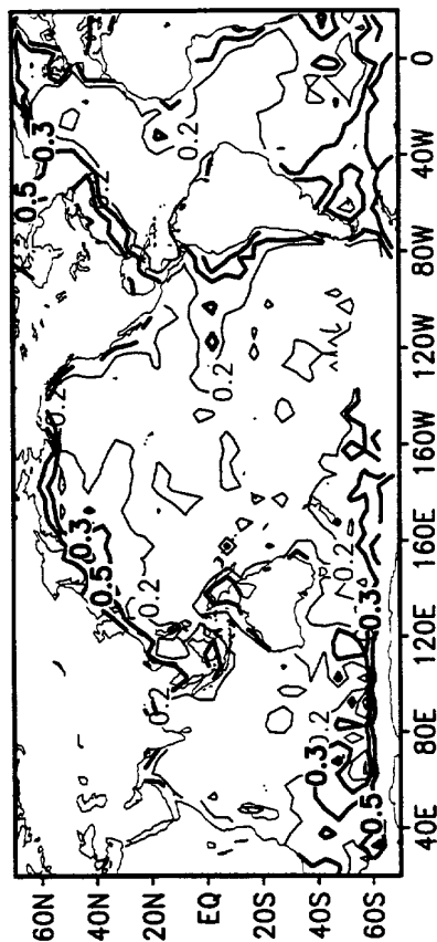
BMRC SST Anomaly (°C)
