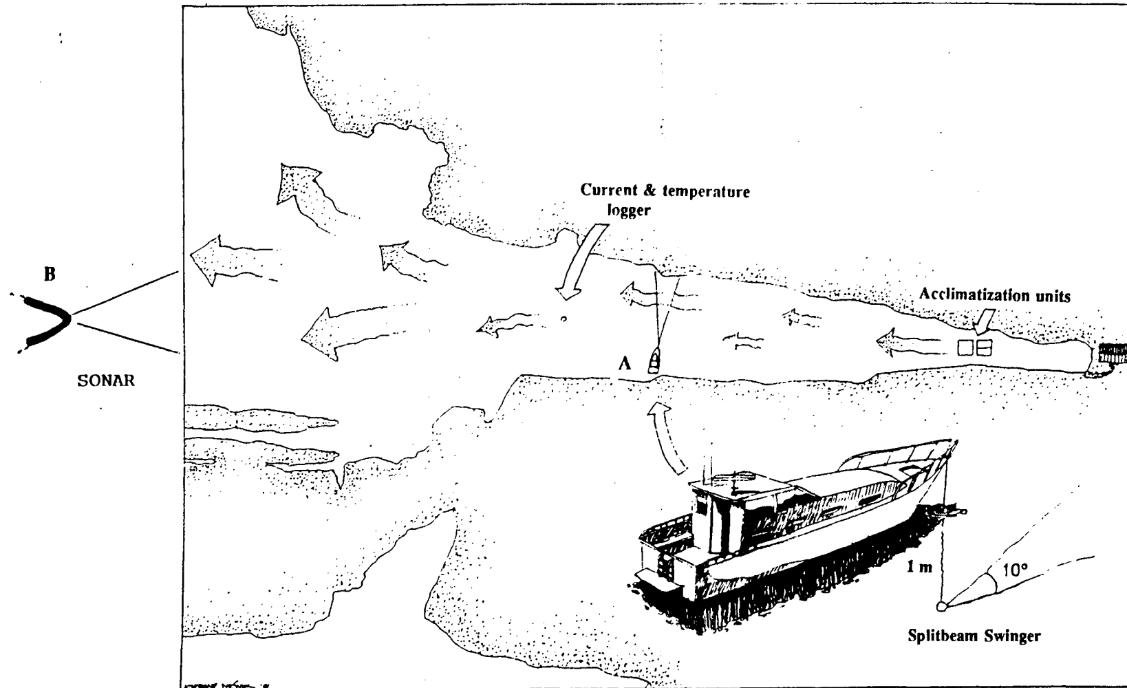
Fig.2. Setup of tracking in Selstøvågen.
