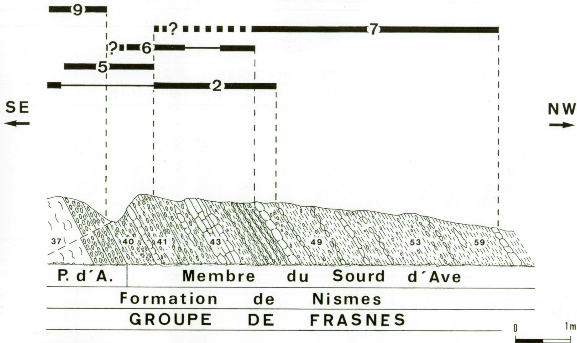
Fig. 5. – Dessin de l'affleurement LJ-1978-1B indiquant les différentes unités litho-stratigraphiques et l'extension des espèces d'Atrypidae. Seule la partie de la coupe ayant livré des Atrypidae a été dessinée. La signification des chiffres est donnée dans l'explication de la figure 4 dans le texte.
