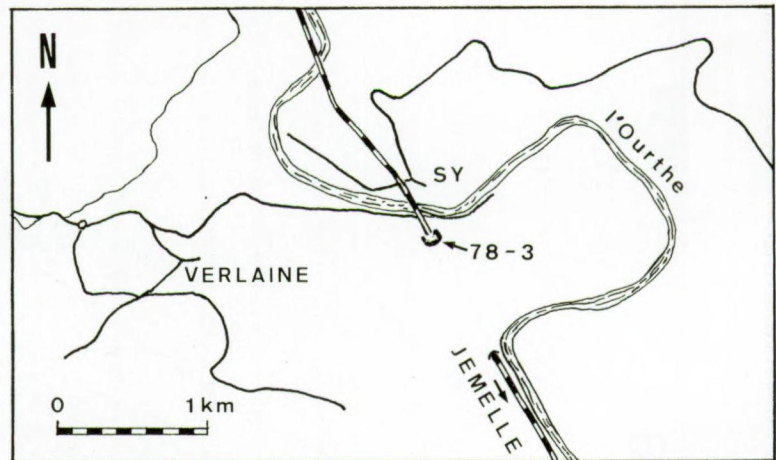
Fig. 13. – Localisation de l'affleurement LJ-1978-3 (78-3).
