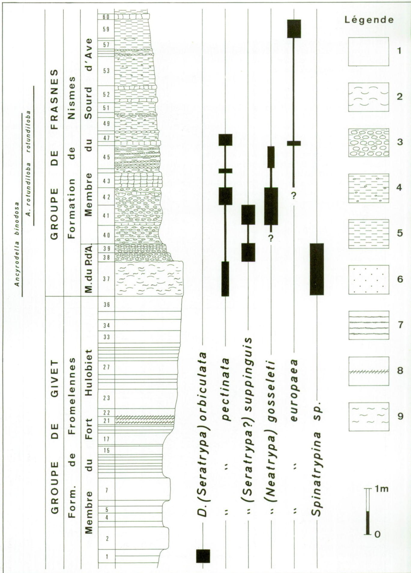
Fig. 3. — Extension verticale des Atrypidae dans les affleurements LJ-1978-1A et LJ-1978-1B. Les deux affleurements ont été groupés. Seule la partie de l'affleurement LJ-1978-1B ayant livré des Atrypidae a été figurée.
