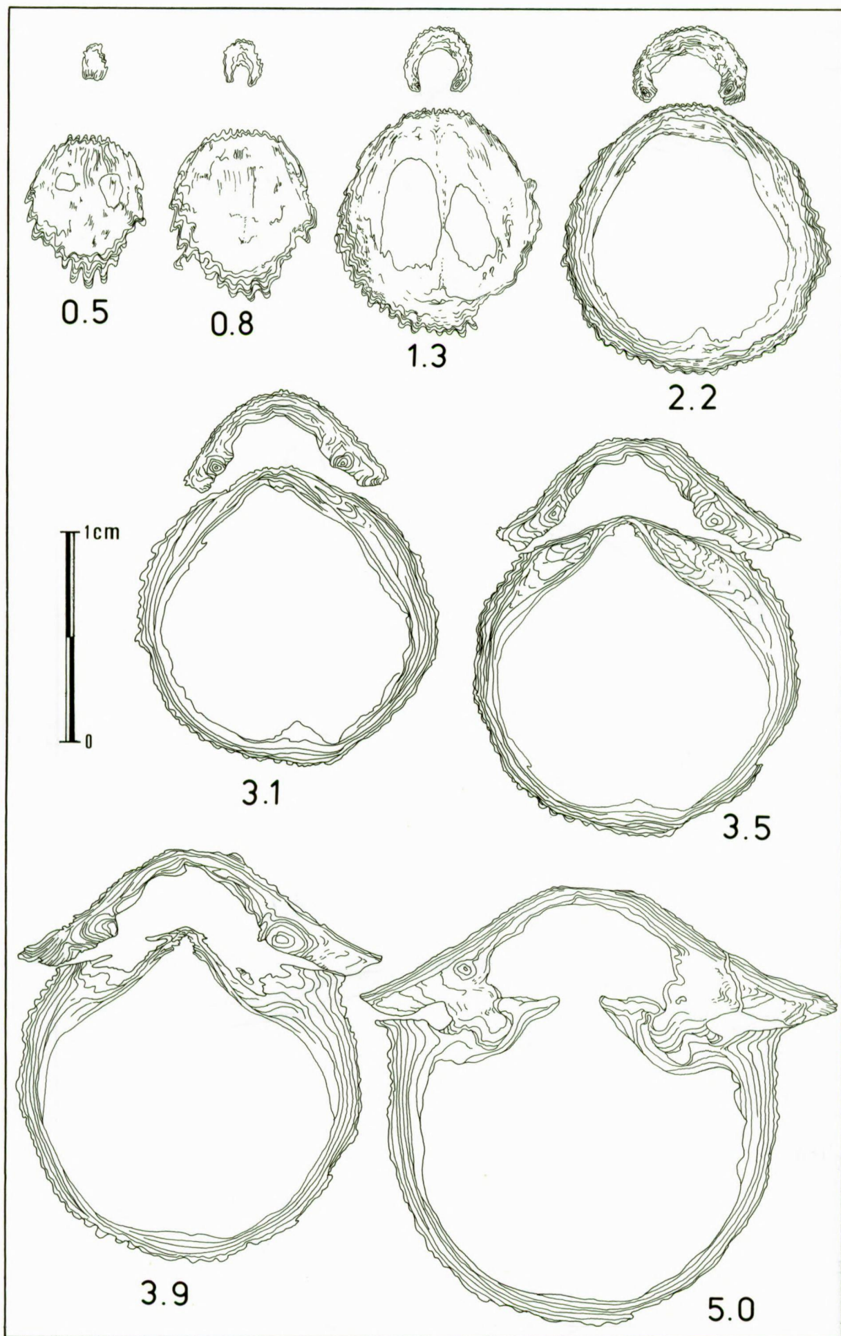
Fig. 21. – Desquamatia (Seratrypa?) suppinguis n. sp. Paratype G. Sections s eriees transverses; les distances, en millim etres, sont mesur ees depuis le sommet de l'umbo dorsal.
