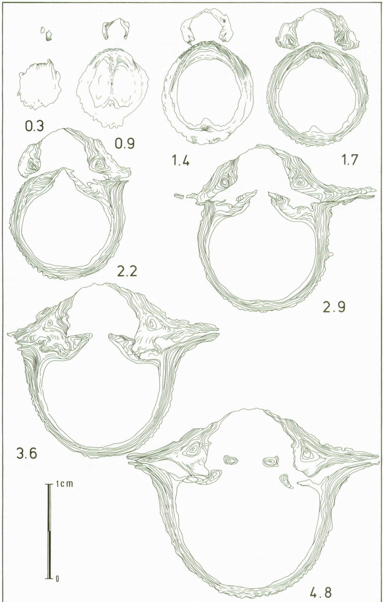
Fig. 22. - Desquamatia (Neatrypa) gosseleti n. sp. Paratype E. Sections s eries transverses; les distances, en millim tres, sont mesur es depuis le sommet de l'umbo dorsal.
