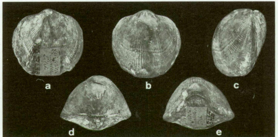
Fig. 18. Terebratulites priscus von SCHLOTHEIM, E., 1820. Museum für Naturkunde der Humbolt-Universität zu Berlin, MB.B.426.
