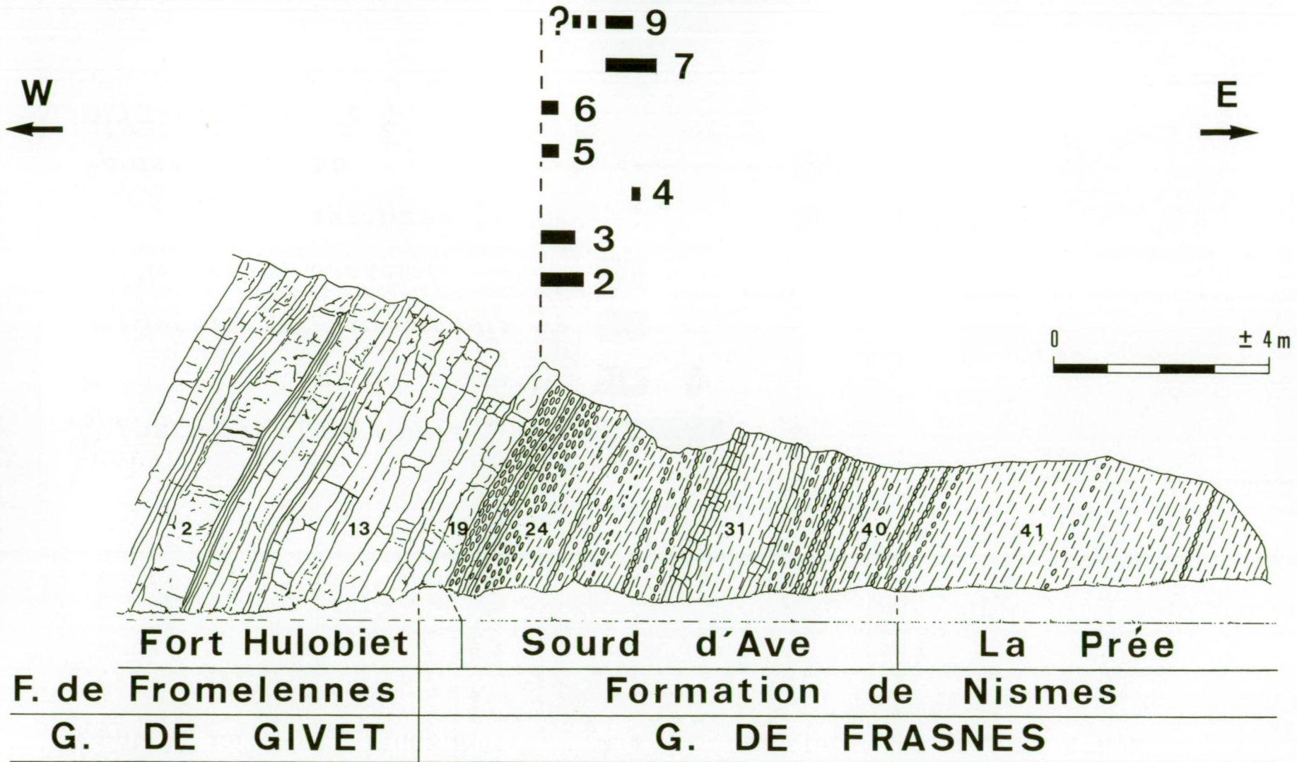
Fig. 12. – Dessin de l'affleurement LJ-1978-2 indiquant les différentes unités litho-stratigraphiques et l'extension des espèces d' Atrypidae . La signification des chiffres est donnée dans l'explication de la figure 4 dans le texte.
