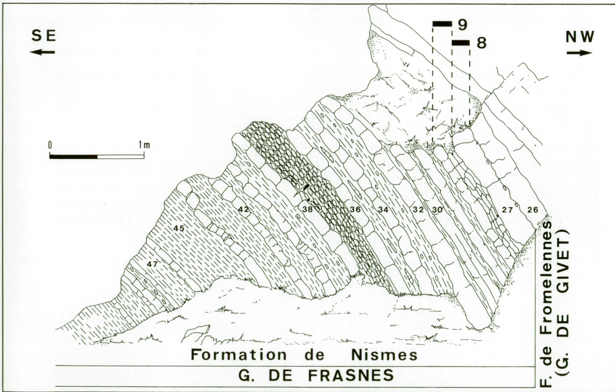
Fig. 15. – Dessin de l'affleurement LJ-1978-3 indiquant les différentes unités litho-stratigraphiques et l'extension des espèces d'Atrypidae. La signification des chiffres est donnée dans l'explication de la figure 4 dans le texte.
