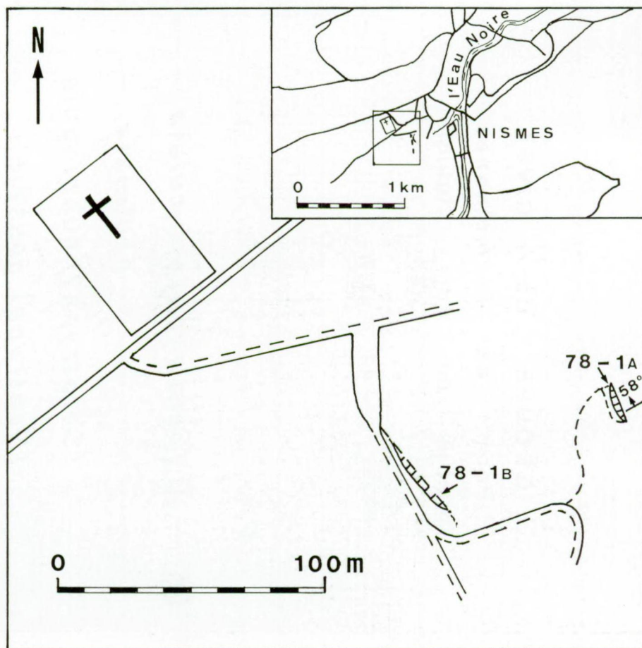
Fig. 2. Localisation des affleurements LJ-1978-1A (78-1A) et LJ-1978-1B (78-1B). Le plan schématique à grande échelle correspond à la partie encadrée dans la carte occupant la partie supérieure droite de la figure.
