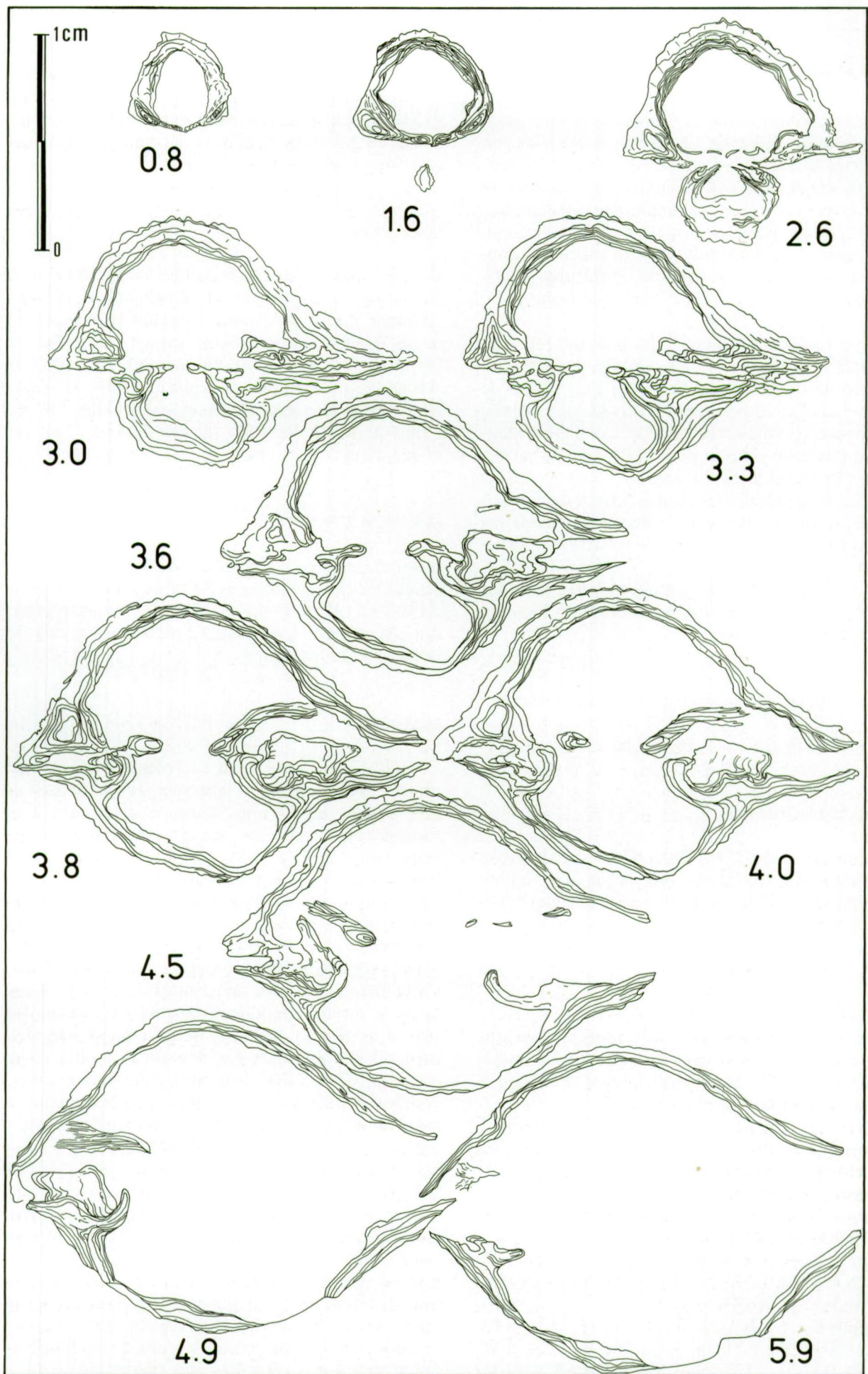
Fig. 16. – Desquamatia (Independatrypa) coenaubertorum n. sp. Paratype F. Sections séries transverses; les distances, en millimètres, sont mesurées depuis le crochet ventral.
