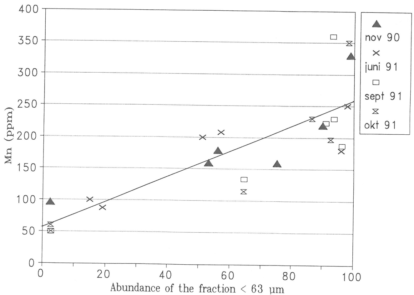
Figuur 2. Totale Mn concentratie in functie van de abundantie van de fractie < 63 \mu\text{m} .
