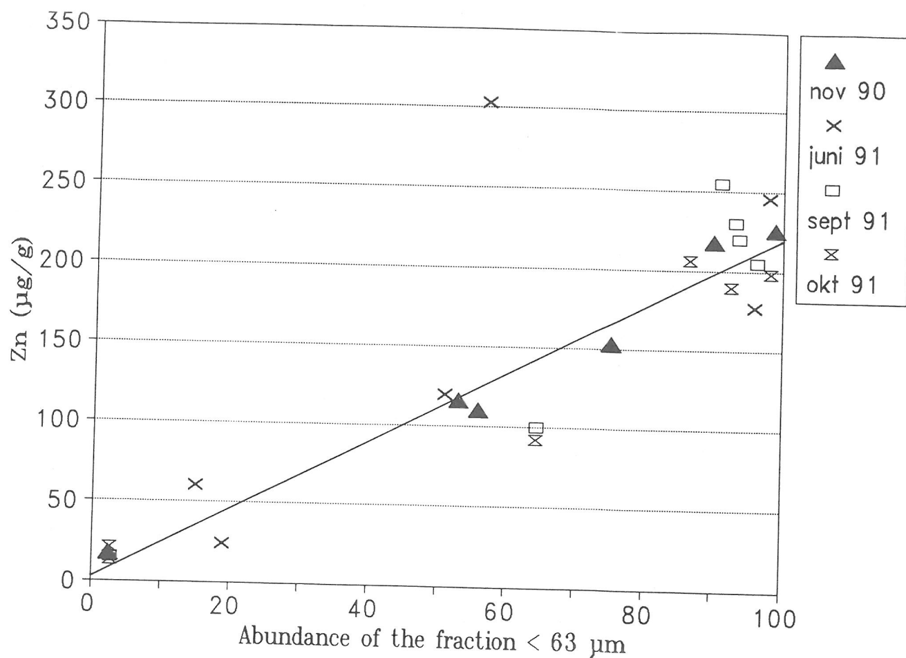
Figuur 5. Totale Zn concentratie in functie van de abundantie van de fractie < 63 \mu\text{m} .
