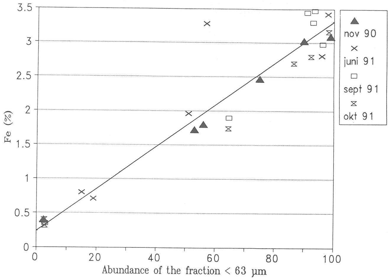
Figuur 3. Totale Fe concentratie in functie van de abundantie van de fractie < 63 \mu\text{m} .
