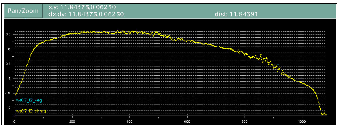
Figuur 3.7b: Profiel over de plaat ten noorden van Terneuzen uit levering 2, de filtering is goed aangepast.
