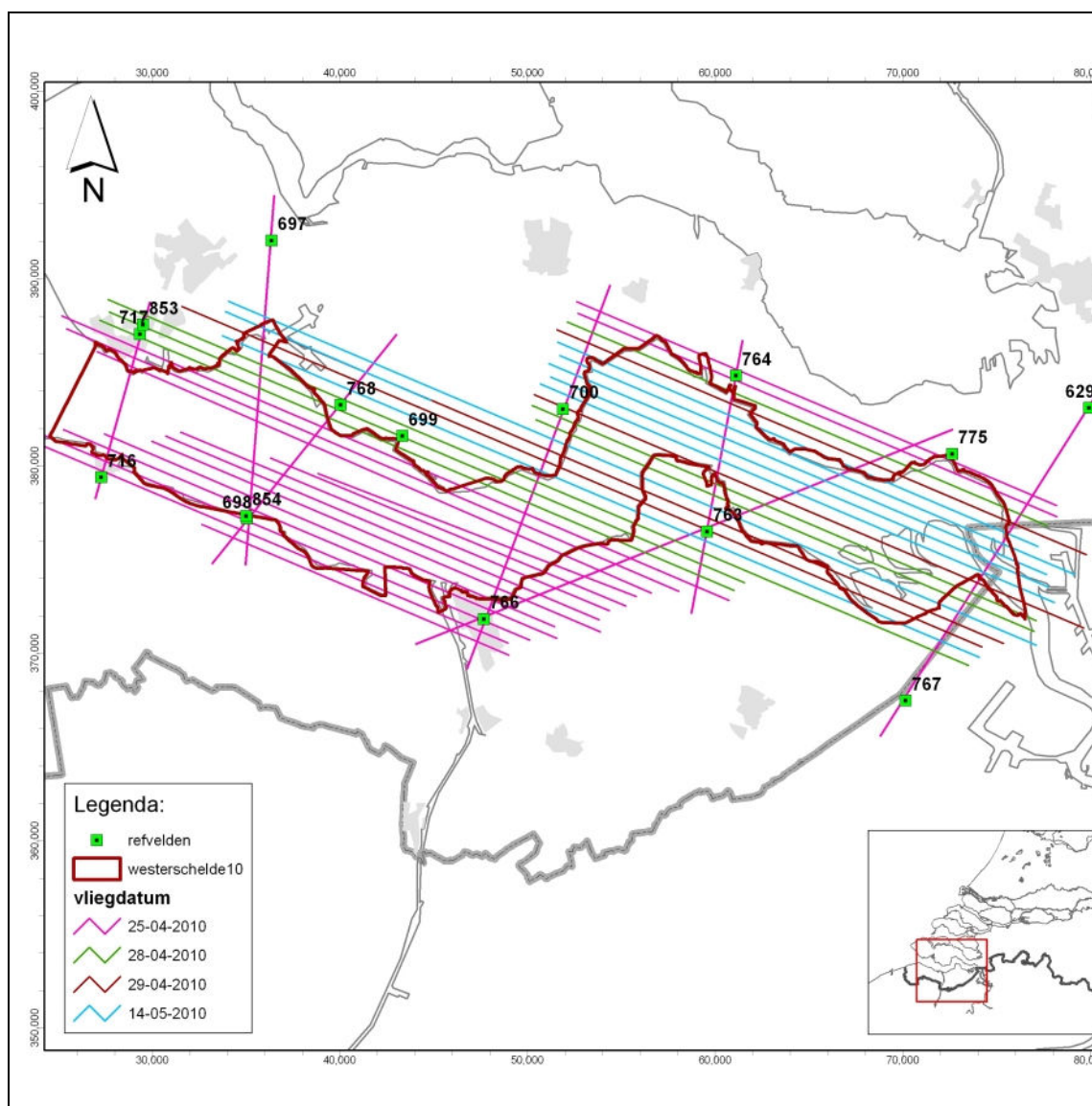
Figuur 3.2: Overzicht vluchtlijnen projectgebied Westerschelde 2010
