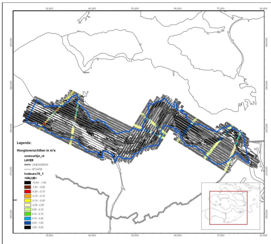
Figuur 3.5b: Verschilgrid van de dwarsstroken en de maaiveld-laserdata.
