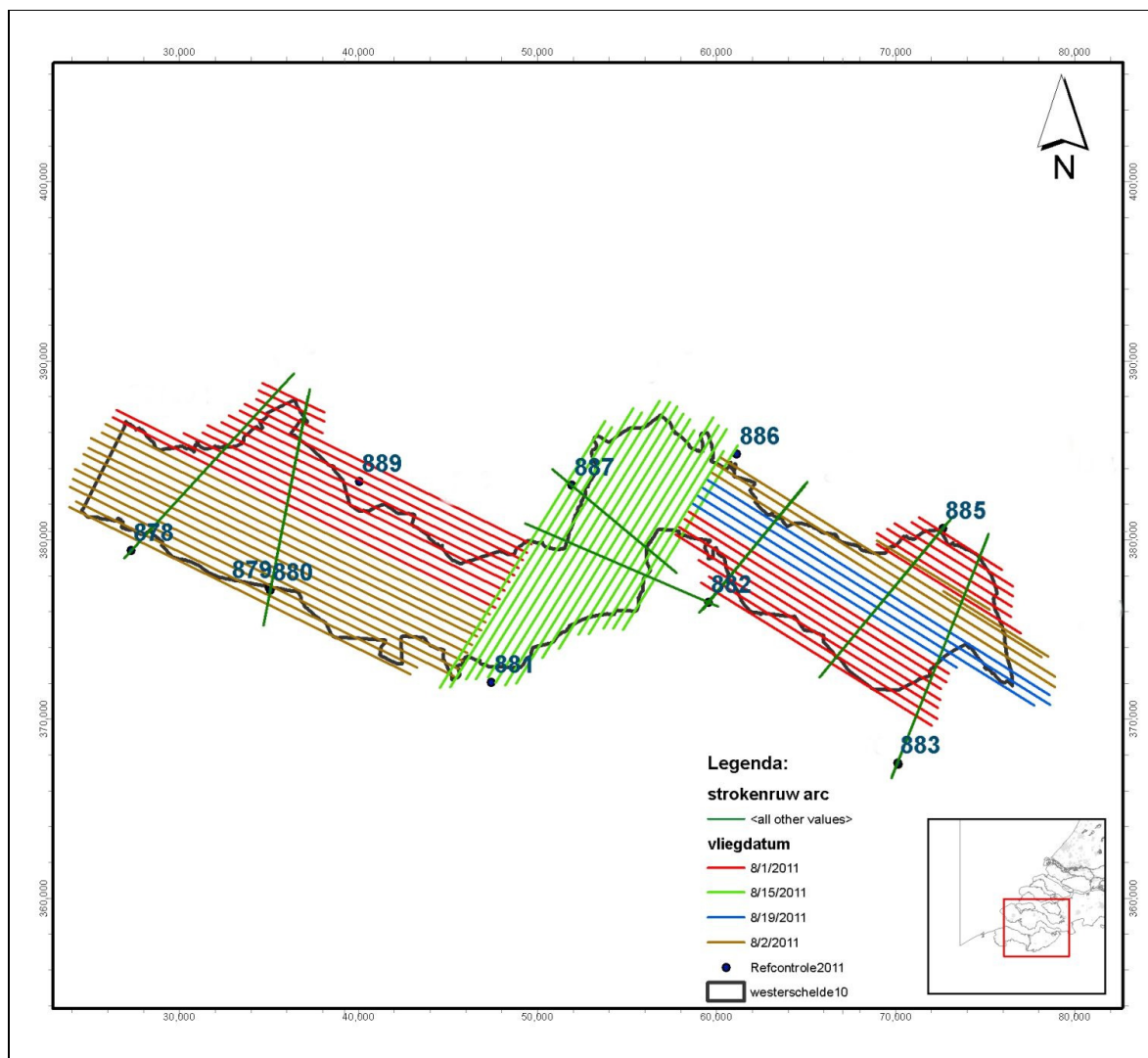
Figuur 3.2: Overzicht vluchtlijnen projectgebied Westerschelde 2011
