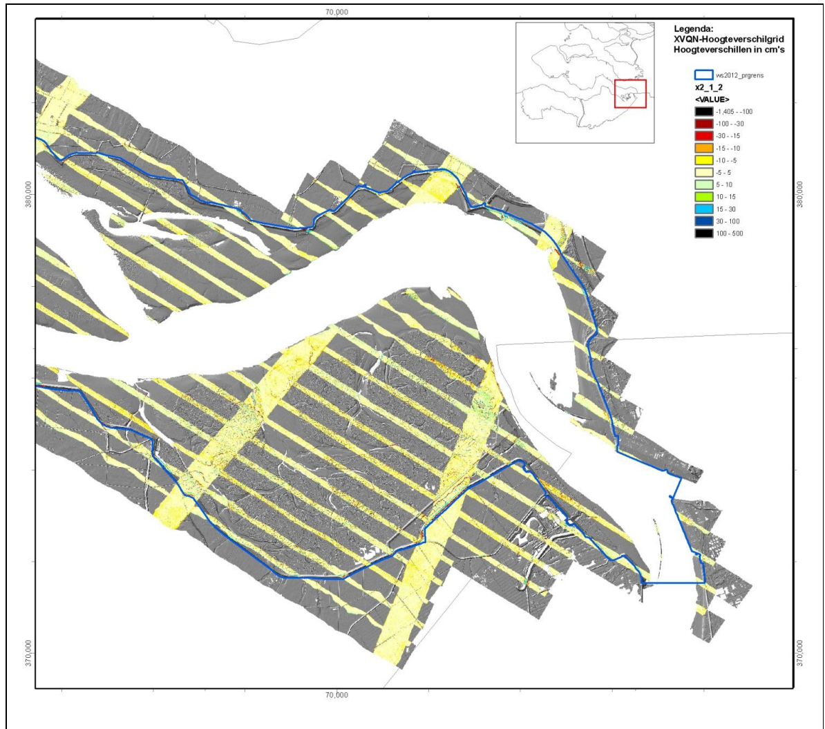
Figuur 3.5b: Detail van het hoogteverschilgrid van de overlappen van de laserdata.
