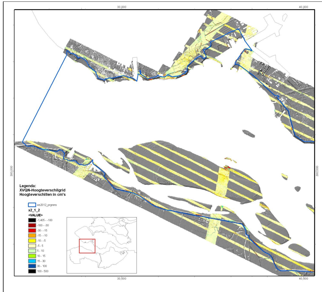
Figuur 3.5a: Detail van het hoogteverschilgrid van de overlappen van de laserdata.
