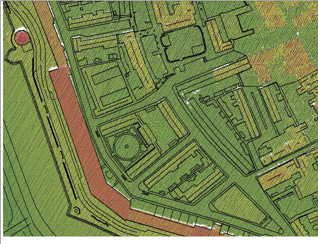
Figuur 3.6: De planimetrie controle is uitgevoerd d.m.v. vergelijking met dtb-lijnen.
