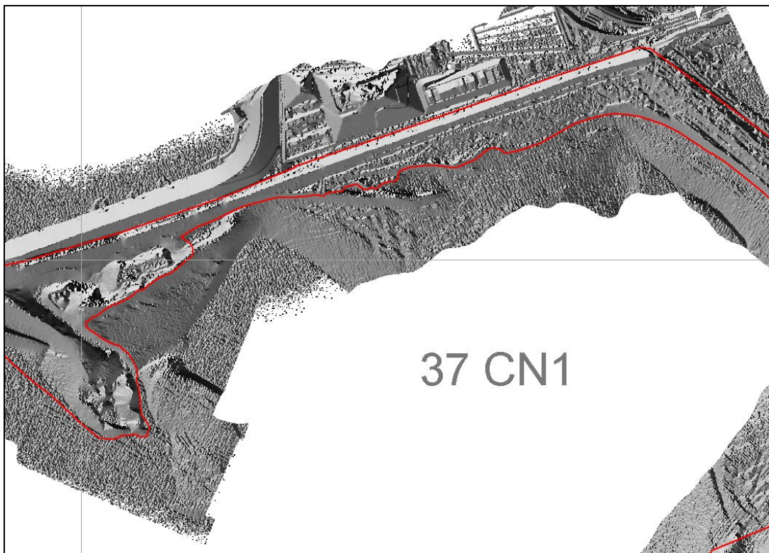
Figuur 8.9a: Aspectgrid (ruw), het betreft een gedeelte van het deelgebied Holland. De rode lijn is de indicatieve water/land grens.
