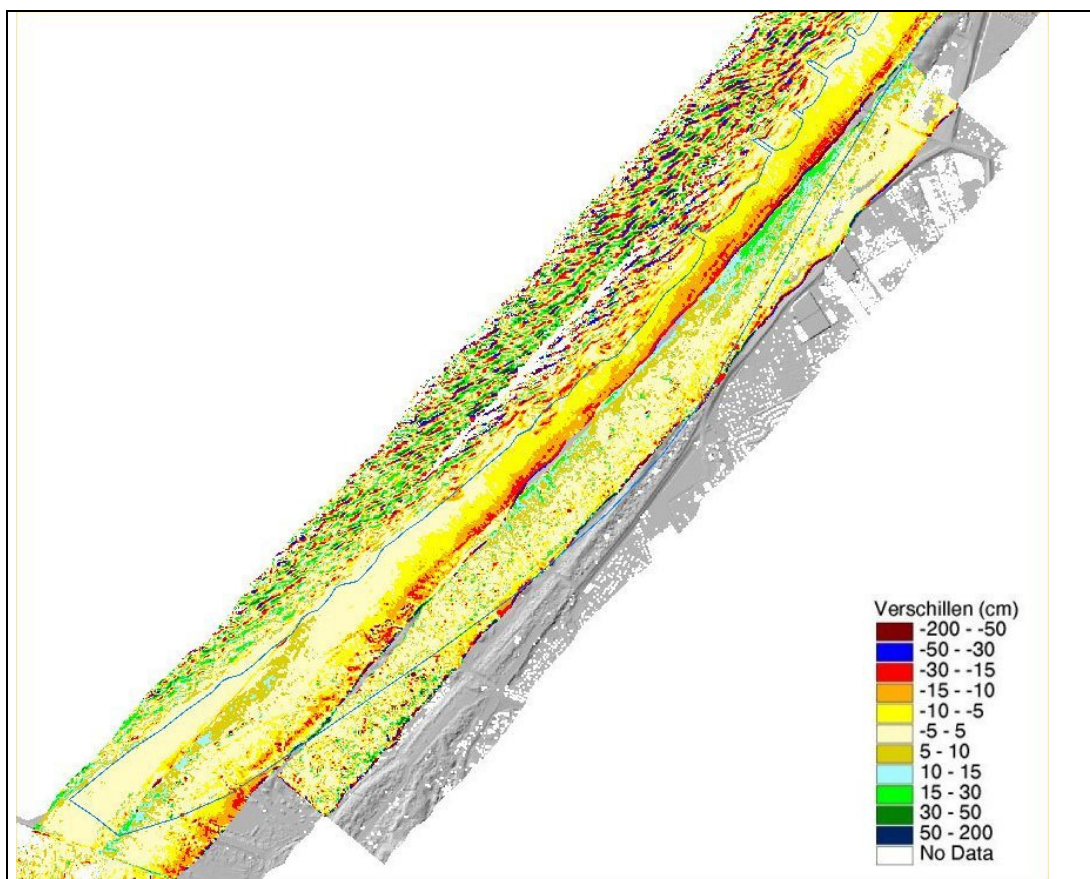
Figuur 8.6b: Detail van het verschilgrid van de overlappen van de laserhoogtedata deelgebied Holland met als ondergrond een hillshade. Hierin is duidelijk te zien dat er verschillen tussen de stroken optraden tot 30 centimeter. De veelgekleurde streepjes (boven en links) zijn de verschillen boven zee.
