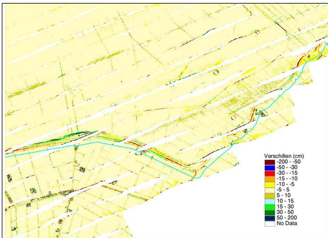
Figuur 8.6e: Detail van het verschilgrid van de overlappen van de laserhoogtedata deelgebied Friese Kwelders.
