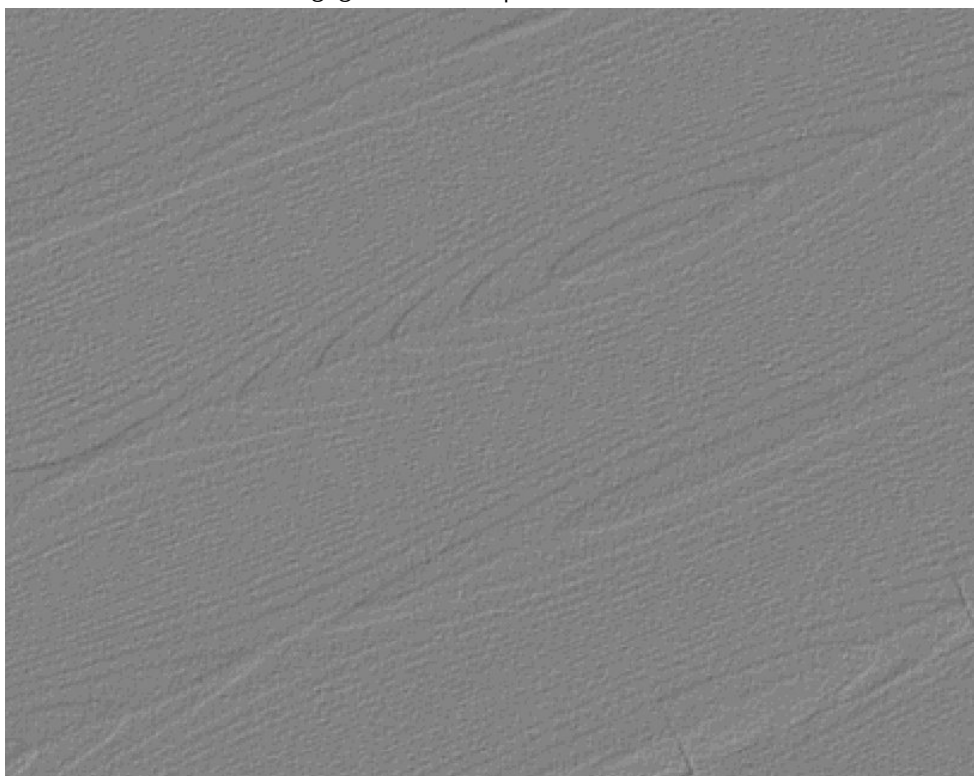
Figuur 8.8a: Voorbeeld van het houtnerfpatroon. De afbeelding is van de hillshade van het deelgebied Friese Kwelders.
