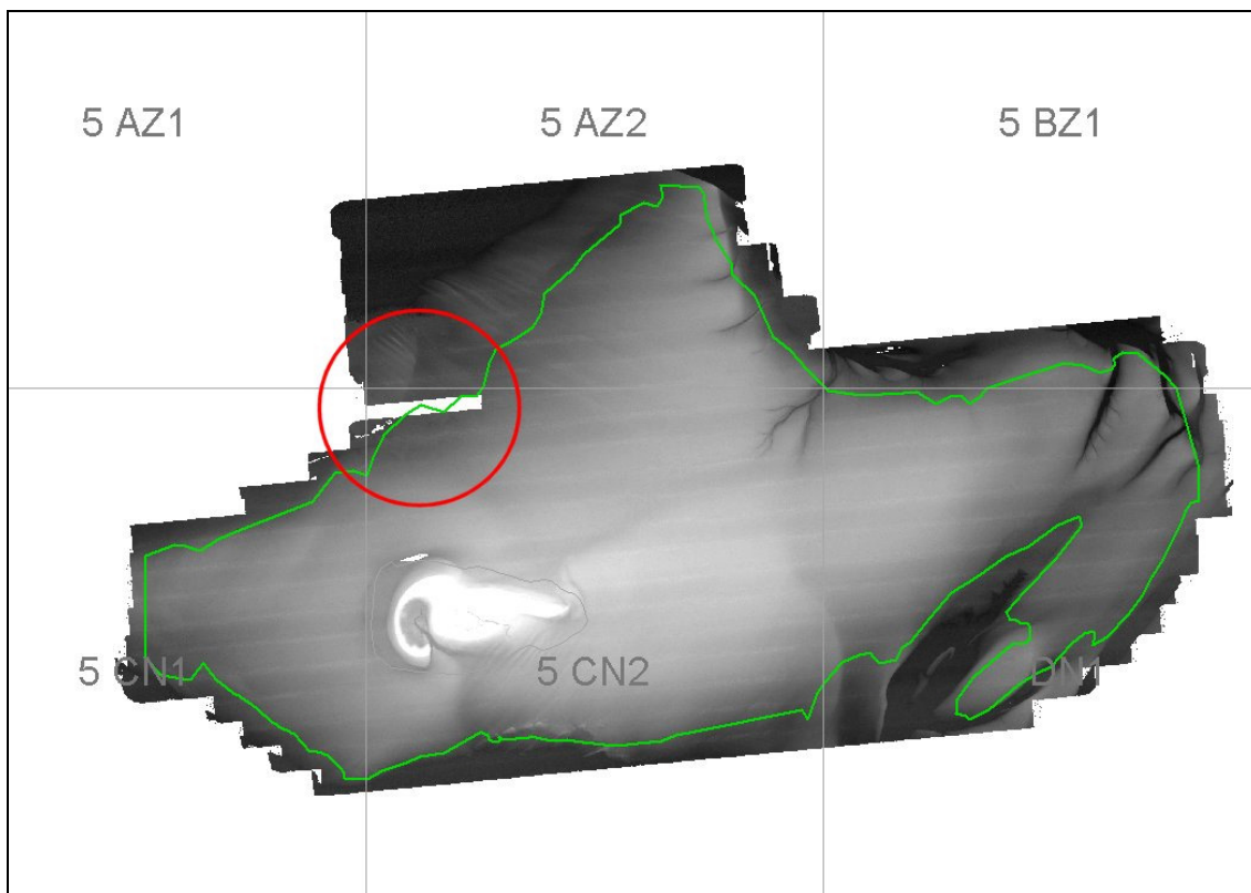
Figuur 8.5a: Ontbrekende data in het projectgebied Kust 2004, deelgebied Wadplaten.
