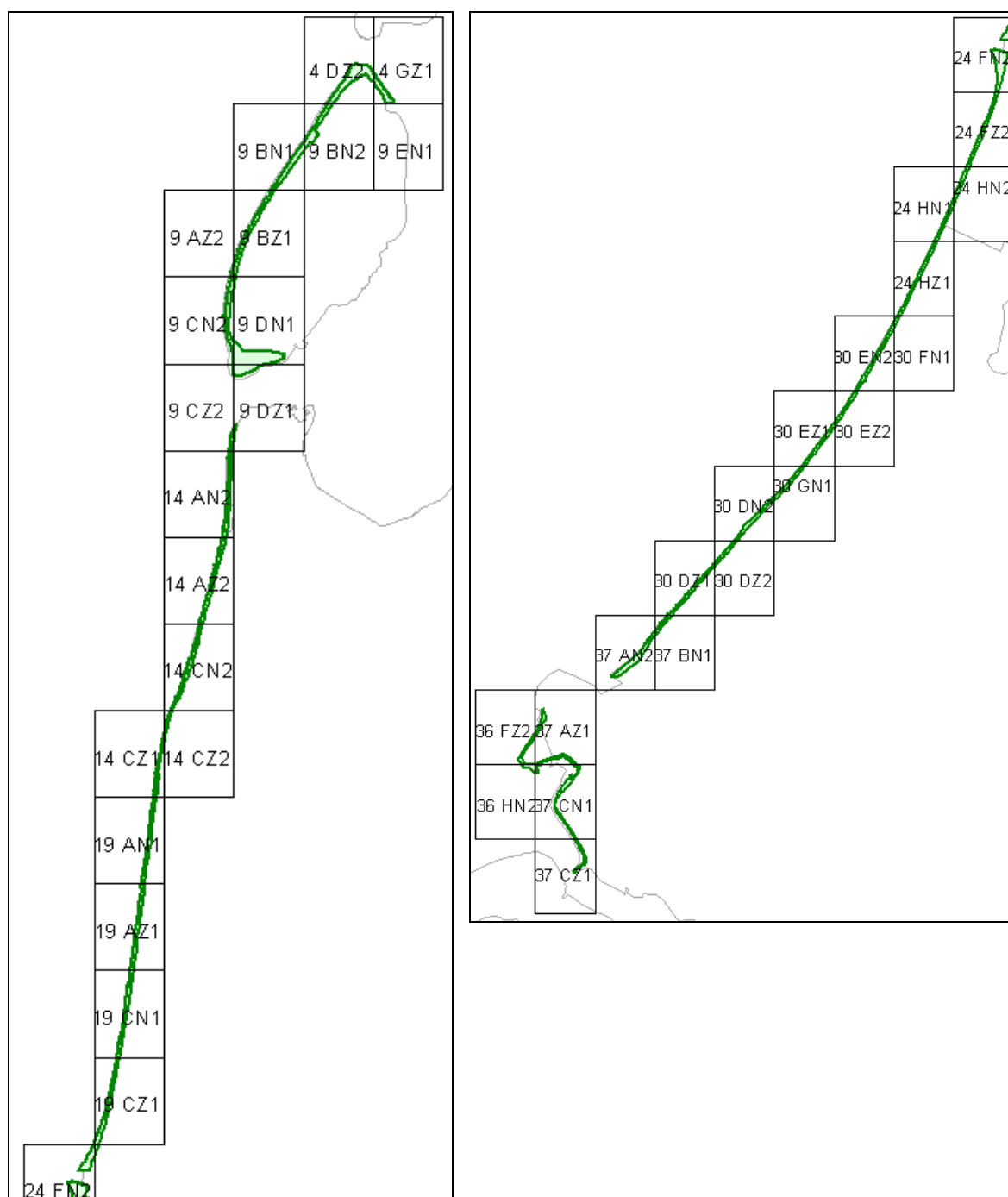
Figuur 8.1b: De kaartbladen van het projectgebied Kust 2004, deelgebied Holland.
