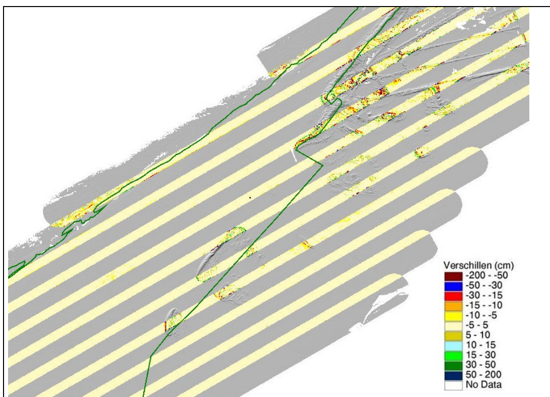
Figuur 8.6c: Detail van het verschilgrid van de overlappen van de laserhoogtedata deelgebied Wadden met als ondergrond een hillshade. Ook hier zijn de stroken geknipt.
