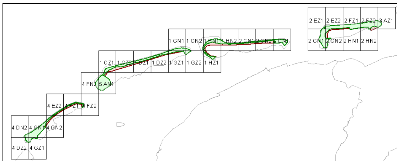
Figuur 8.1c: De kaartbladen van het projectgebied Kust 2004, deelgebied Wadden en aanvulling Wadden..
