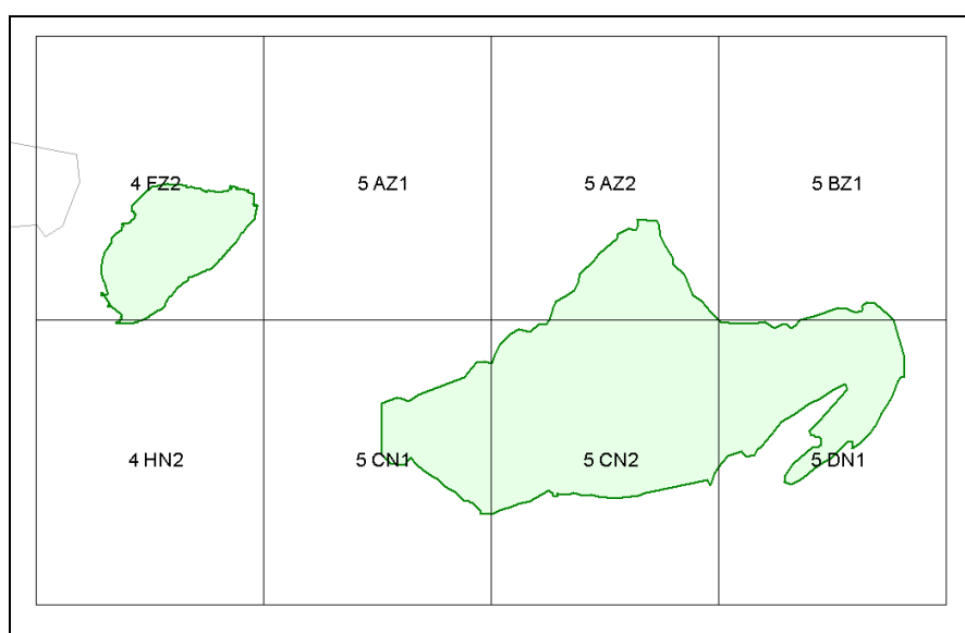
Figuur 8.1d: De kaartbladen van het projectgebied Kust 2004, deelgebied Wadplaten.
