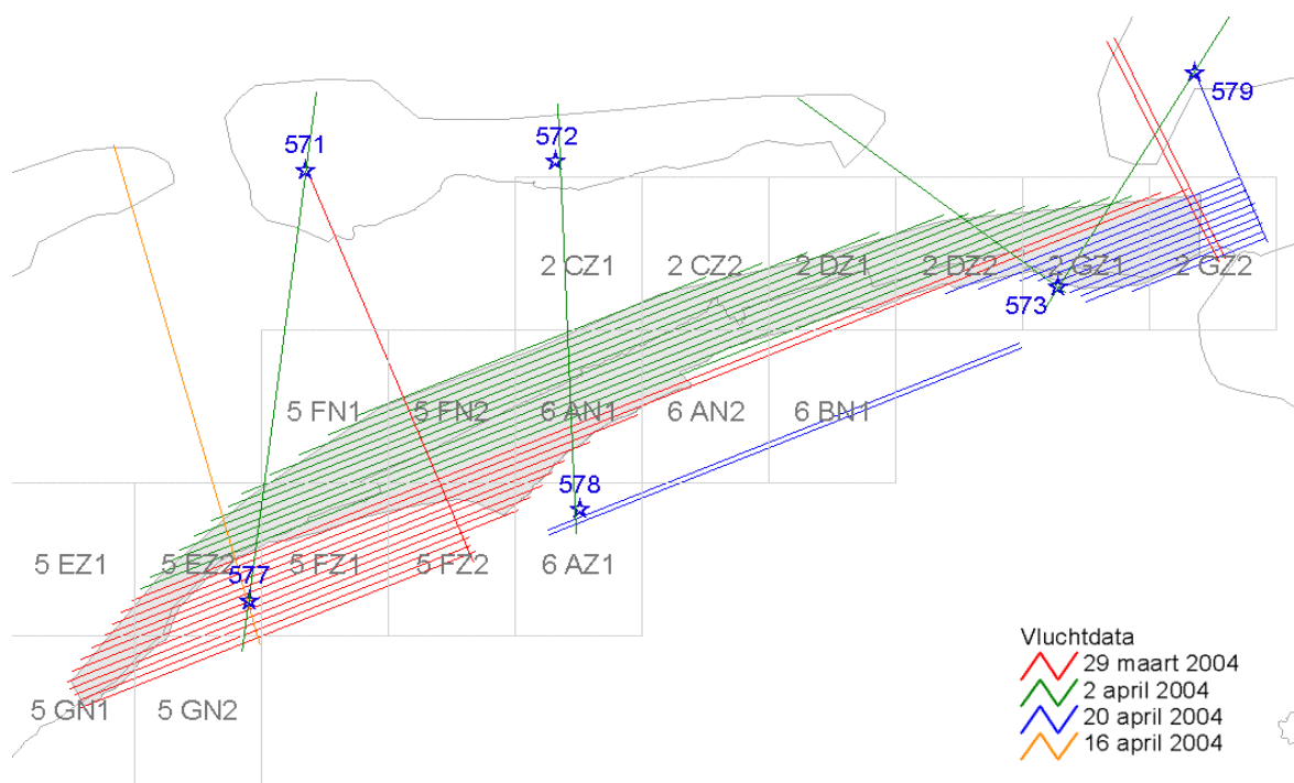
Figuur 8.2e: Overzicht vluchten met vliegdata en locatie referentiegebieden AGI, deelgebied Friese Kwelders.
