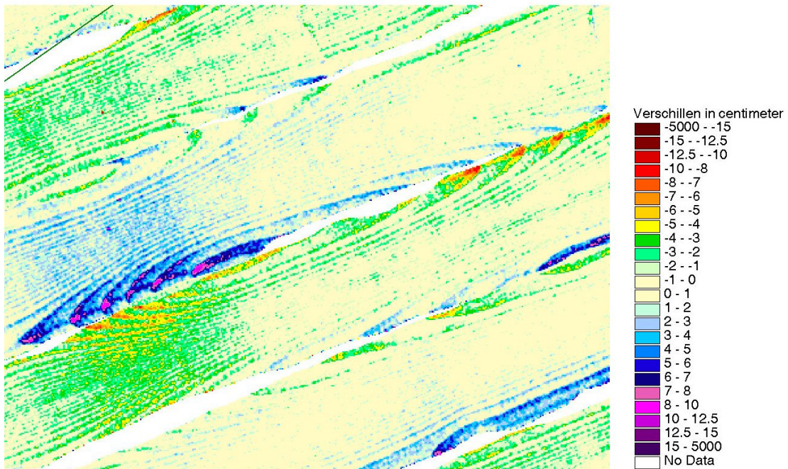
Figuur 8.8b: Hoogteverschilgrid met verschillen in centimeters. Het betreft een gedeelte van het deelgebied Friese Kwelders.
