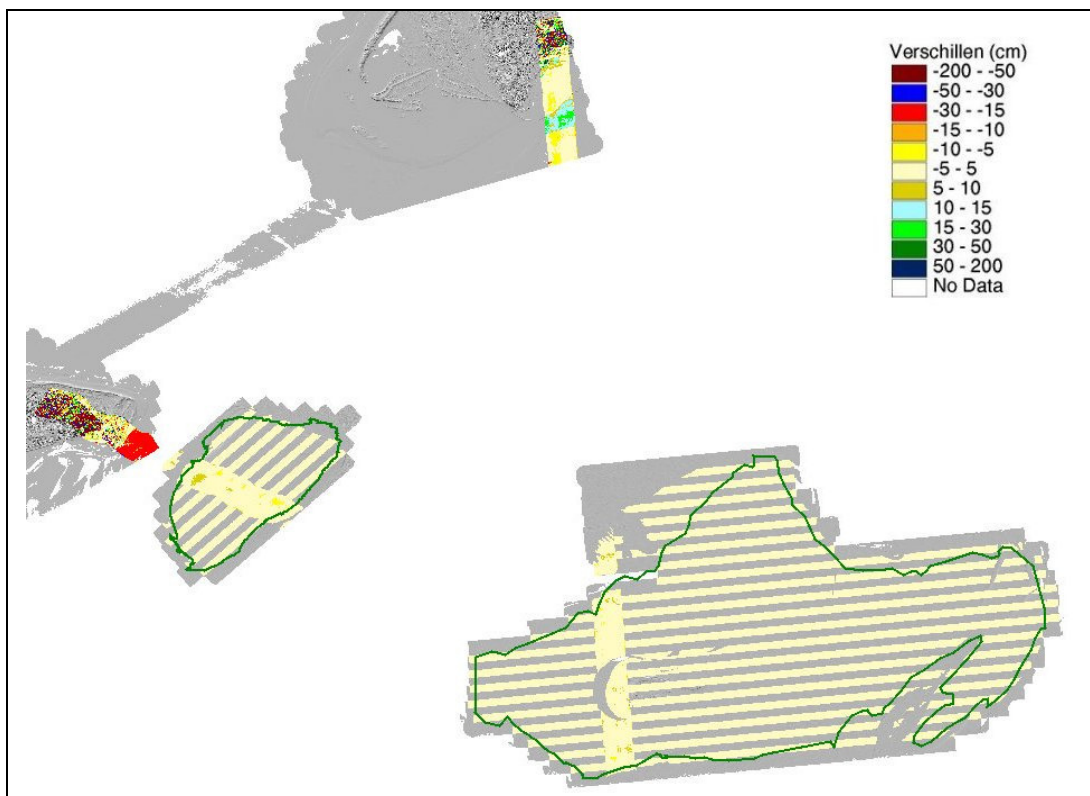
Figuur 8.6d: Detail van het verschilgrid van de overlappen van de laserhoogtedata deelgebied Wadplaten met als ondergrond een ruwe hillshade. De grote verschillen in de dwarsstroken over het gebied Wadden (links rood en rechts groen) komen doordat daar water aanwezig is. Ook hier zijn de stroken weer geknipt.
