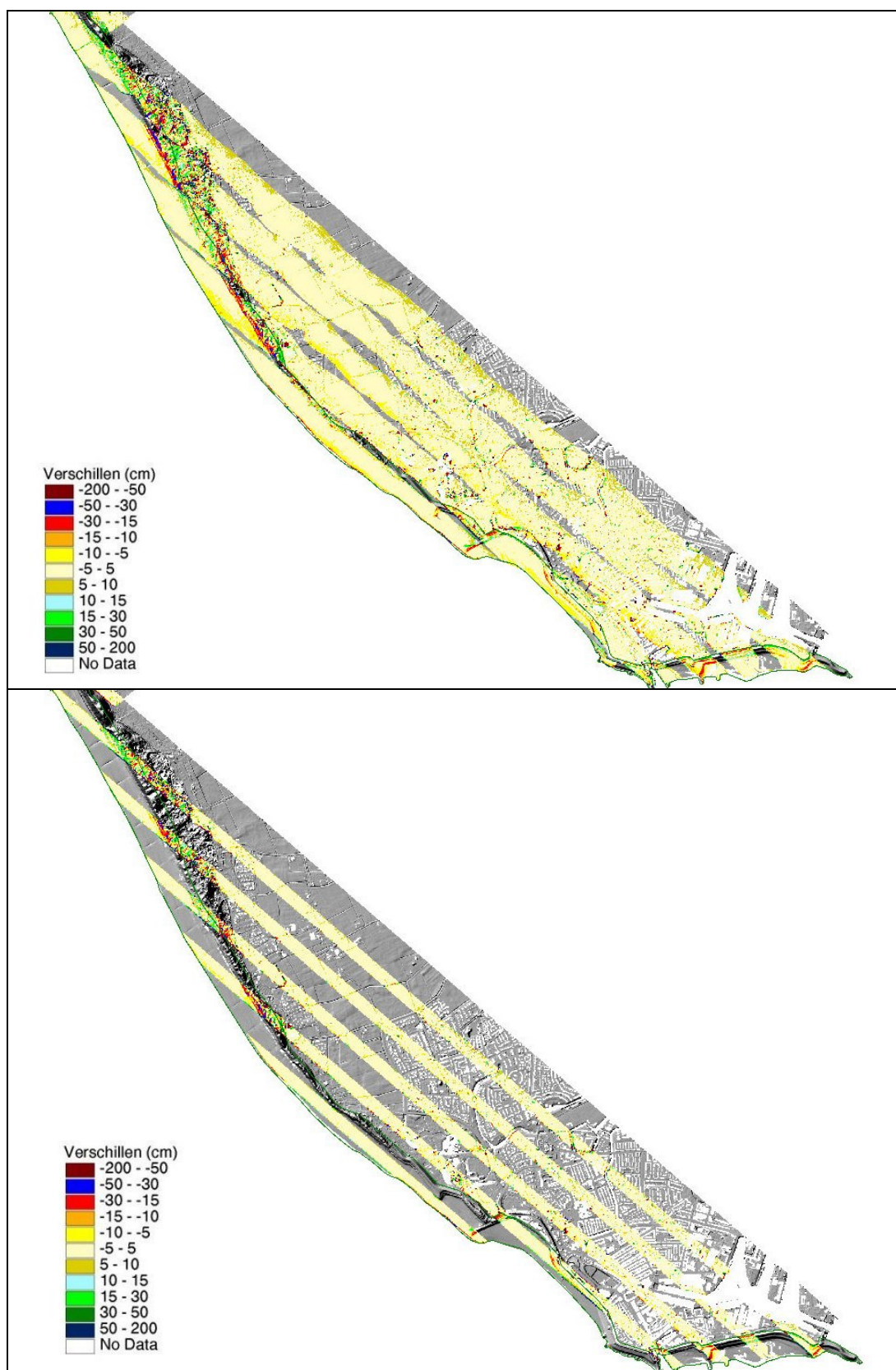
Figuur 8.6a: Detail van het verschilgrid van de overlappen van de laserhoogtedata deelgebied Zeeland met als ondergrond een hillshade. Boven is een voorbeeld gegeven van de eerste levering, onder een voorbeeld van de tweede levering. De verschillen die in het bovenste plaatje aan de randen te zien zijn, zijn door het knippen van de stroken in het onderste plaatje verdwenen.
