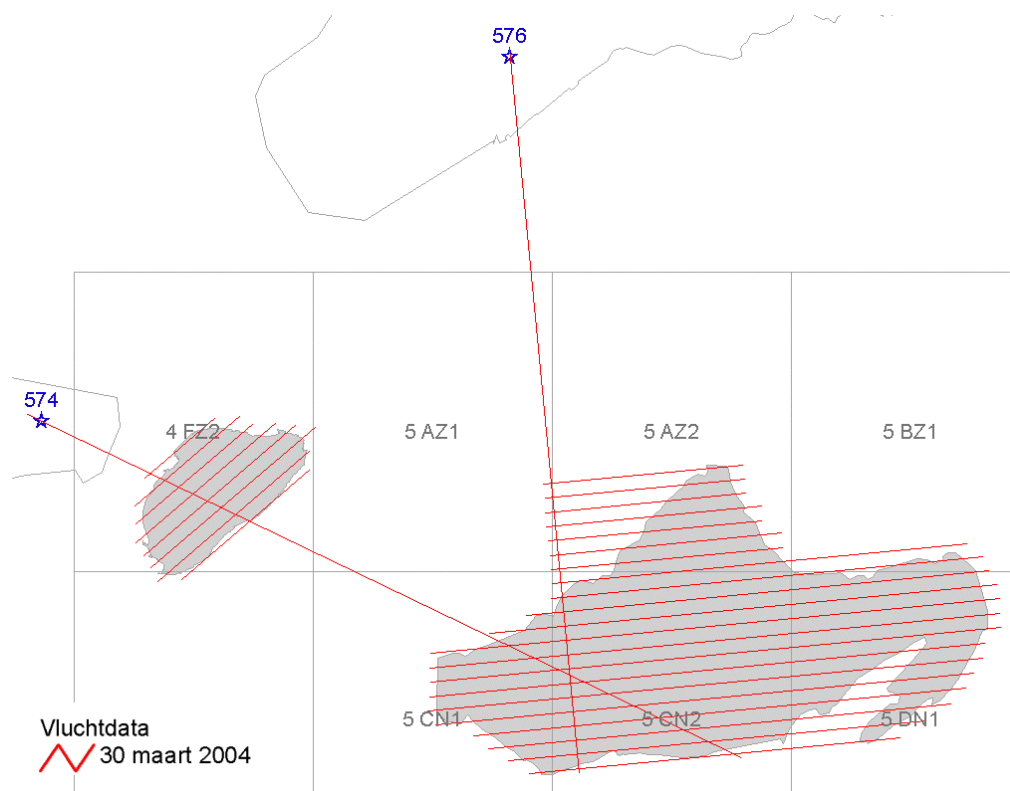
Figuur 8.2d: Overzicht vluchten met vliegdata en locatie referentiegebieden AGI, deelgebied Wadplaten.
