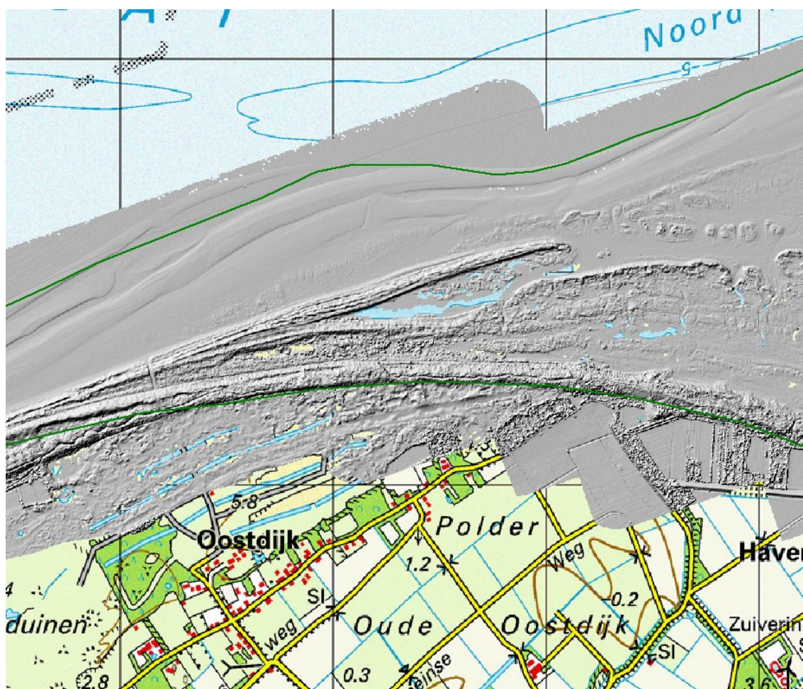
Figuur 8.5b: Detail van een schaduwbestand van de laserhoogtedata van deelgebied Zeeland, Goeree, ten noordoosten van Ouddorp met als ondergrond een TOP50rasterbestand.
