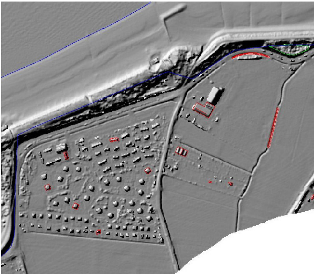
Figuur 8.7: Voorbeeld van de planimetrische controle met behulp van fotogrammetrisch ingewonnen bebouwing.
