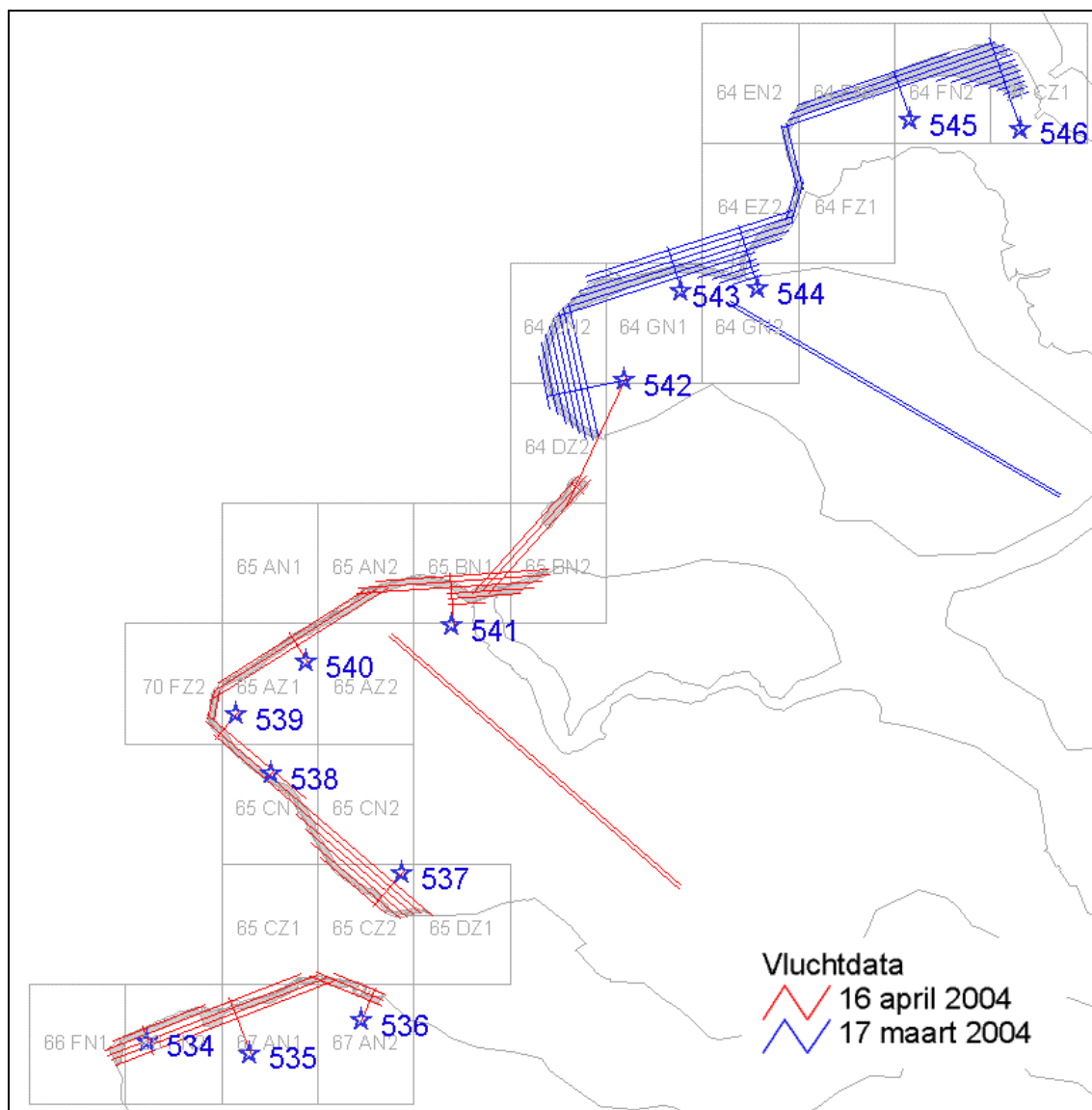
Figuur 8.2a: Overzicht vluchten met vliegdata en locatie referentiegebieden AGI, deelgebied Zeeland.
