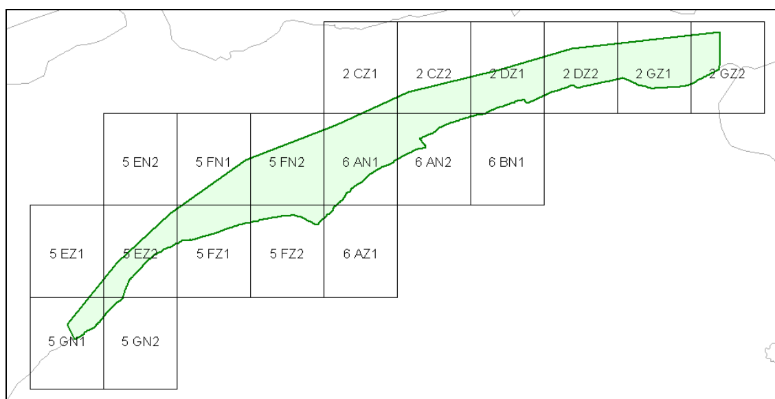
Figuur 8.1e: De kaartbladen van het projectgebied Kust 2004, deelgebied Friese Kwelders.
