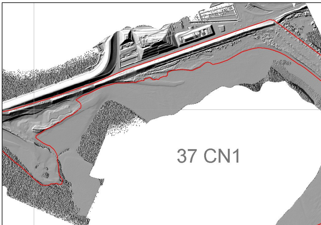
Figuur 8.9b: Aspectgrid (ruw) met daaroverheen de gefilterde hillshade (lichtgrijs). Het betreft een gedeelte van het deelgebied Holland. De rode lijn is de indicatieve water/land grens.
