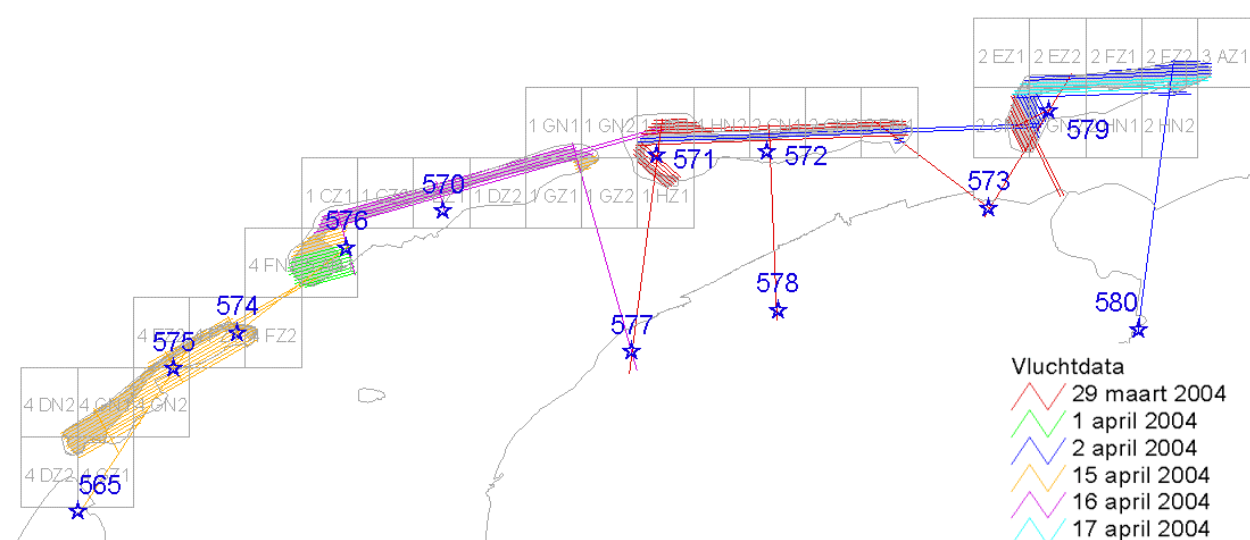
Figuur 8.2c: Overzicht vluchten met vliegdata en locatie referentiegebieden AGI, deelgebied Wadden.
