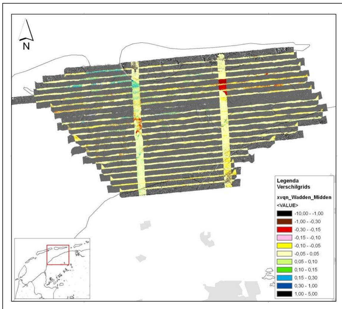
Figuur 3.6a: Hoogteverschillen tussen de overlappende stroken van Wadden Midden, de hoogteverschillen zijn in de kleurentabel in m's weergegeven.
