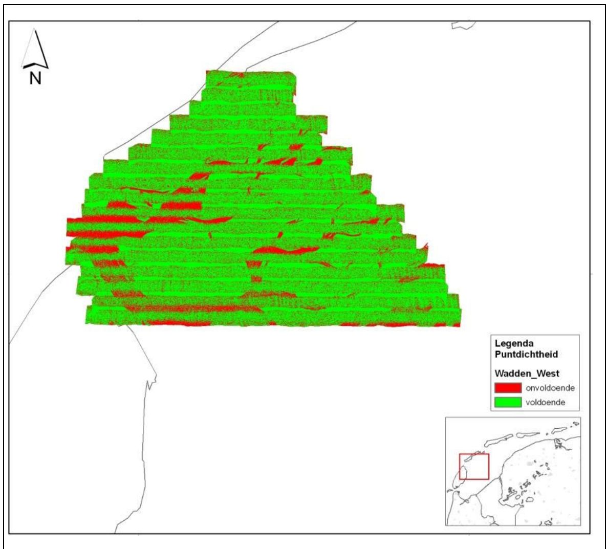
Figuur 3.4b: Overzicht van de punt dichtheid van de laserhoogtedata van het projectgebied Wadden West.
