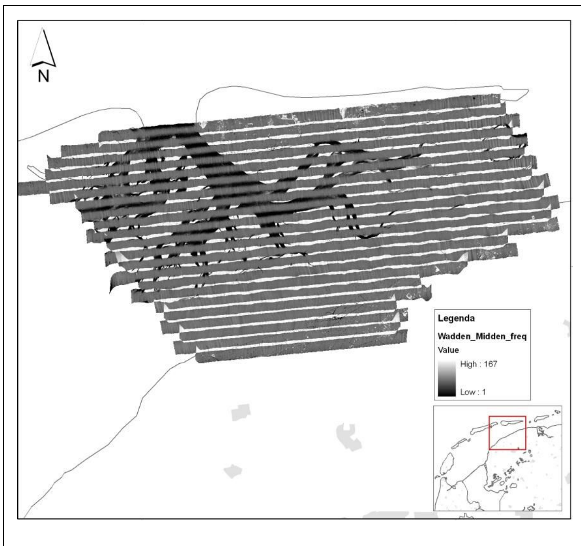
Figuur 3.3a: Frequentiegrid van de ongefilterde laserdata van Wadden Midden.
