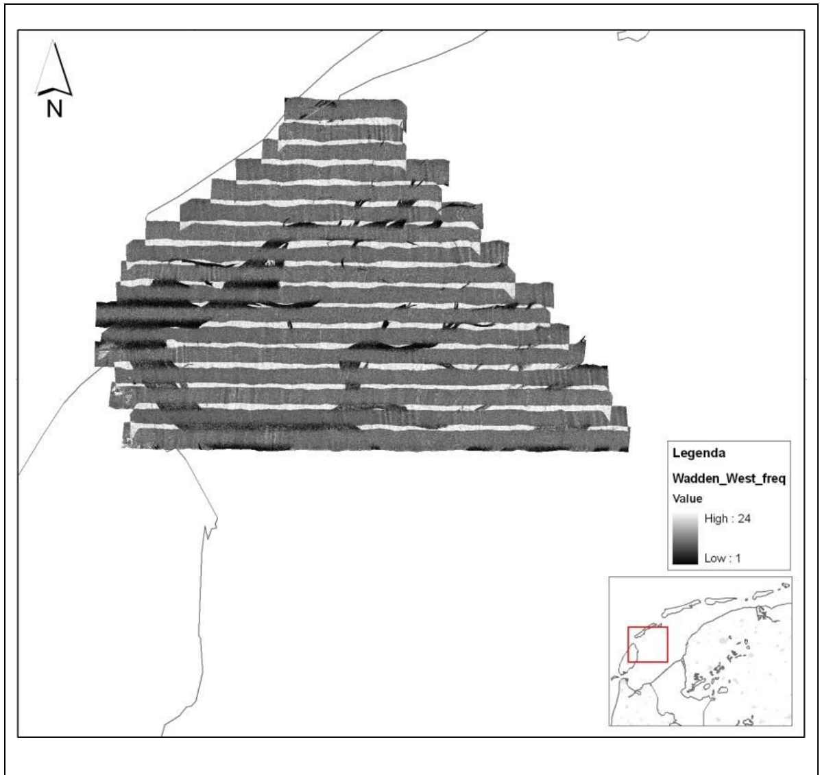
Figuur 3.3b: Frequentiegrid van de ongefilterde laserdata van Wadden West.
