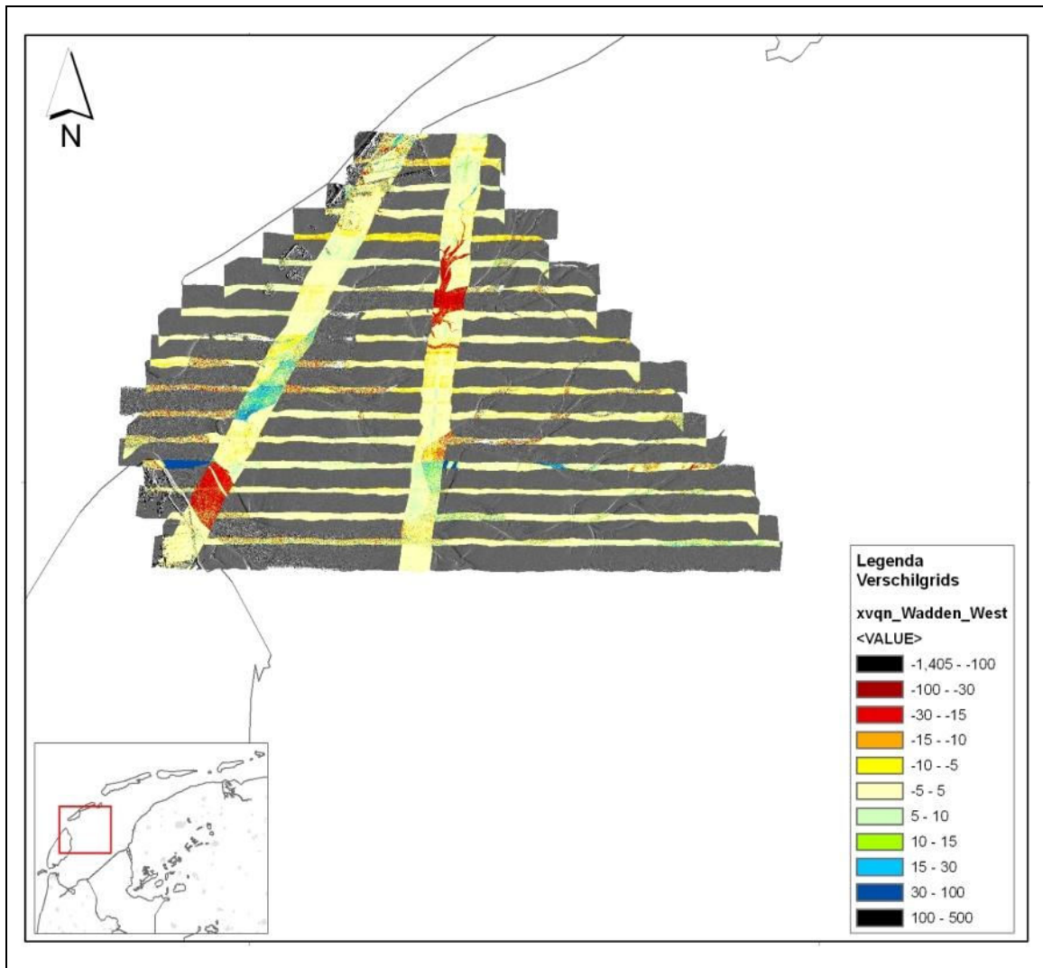
Figuur 3.6b: Hoogteverschillen tussen de overlappende stroken van Wadden West, de hoogteverschillen zijn in de kleurentabel in m's weergegeven.
