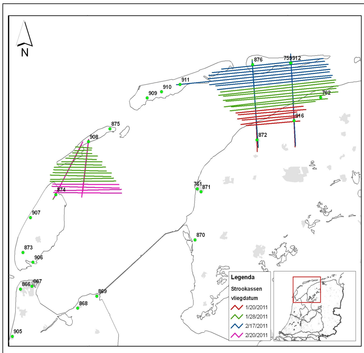
Figuur 3.2a: Overzicht van de vluchtlijnen en referentiegebiedjes van projectgebied Schiermonnikoog.
