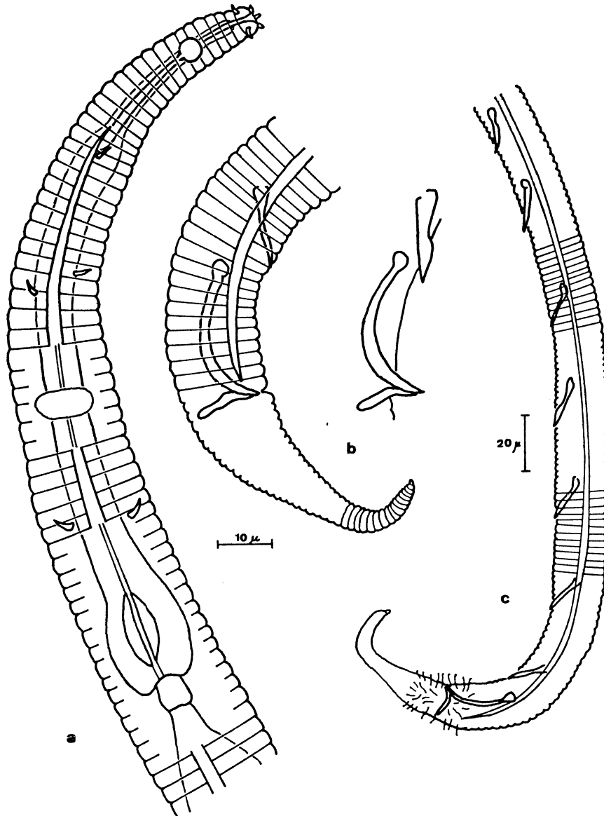
FIG. 3 Leptolaimus alatus .
