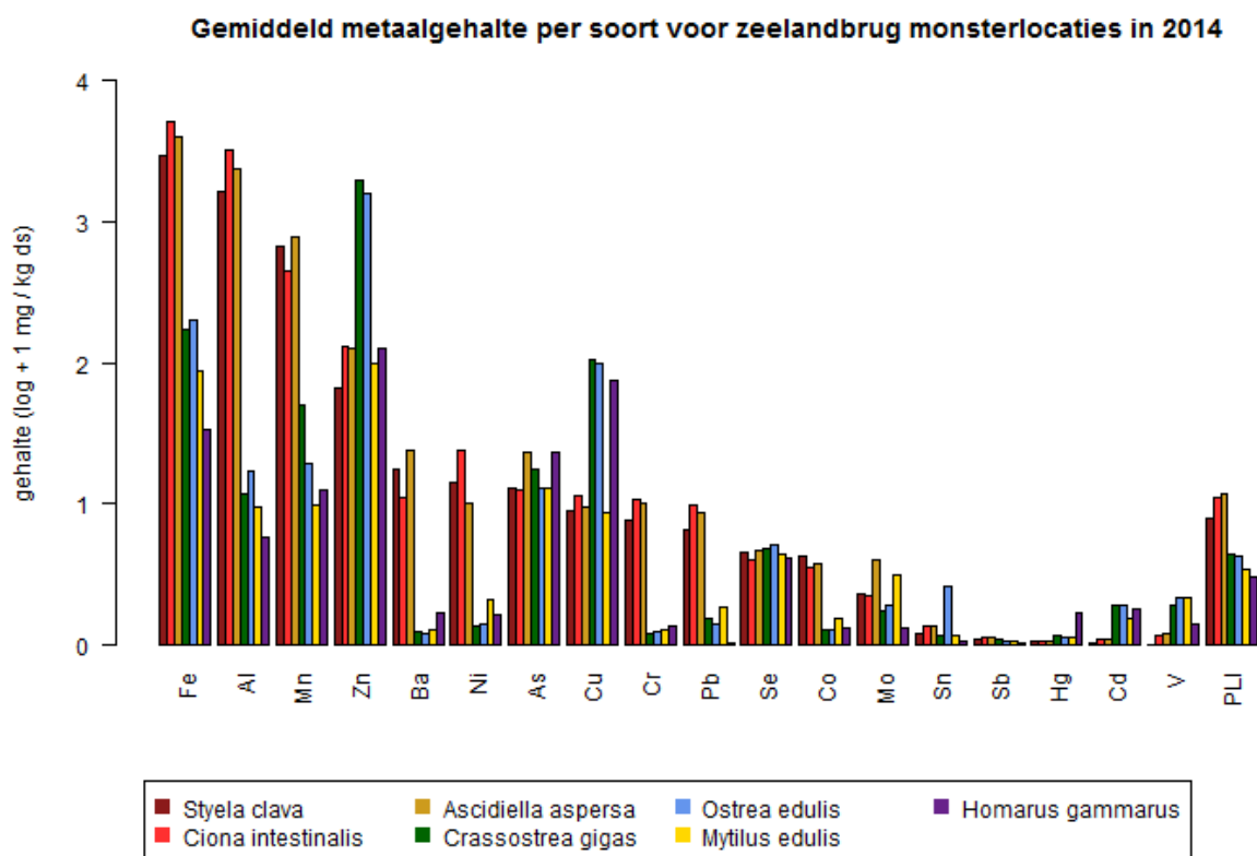
Figuur 4: Gemiddelde metaalgehalte per soort zoals gemeten op de bemonsteringslocaties rond de Zeelandbrug (stort locaties) en bij de Zuidbout (referentielocatie) in 2014.
