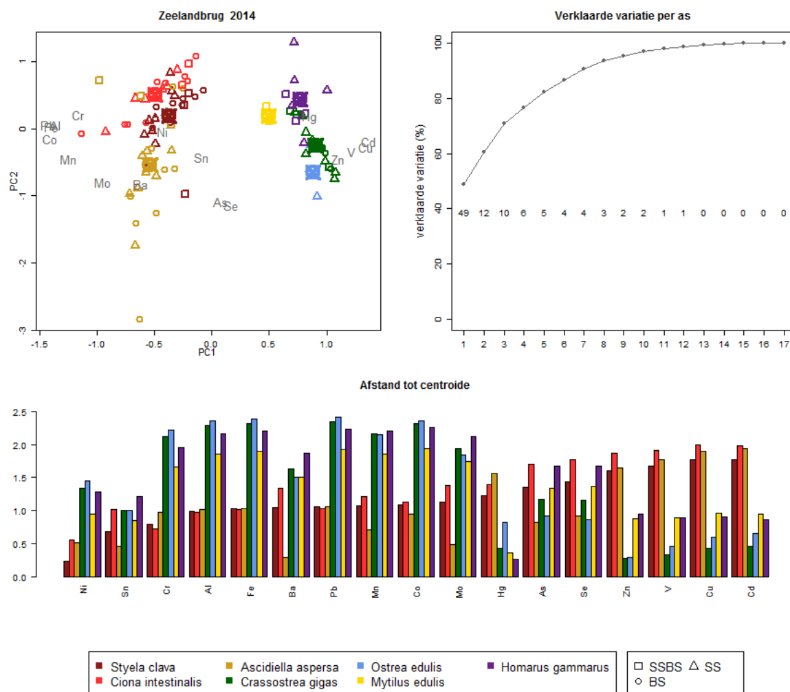
Figuur 12: Linksboven principal component (PCA) oriëntatie op z-gestransformeerde metaalgehalte in de zakpijpsoorten Styela clava , Ciona intestinalis en Asciidiella aspersa , de oesters Crassostrea gigas en Ostrea edulis , de mossel Mytilus edulis en de kreeft Homarus gammarus bemonsterd op de Zeelandbrug in 2014. Scaling factor 2 (nadruk op metaalverschillen). Metalen met meer dan 75% meetwaarden onder de detectielimiet zijn buitenbeschouwing gelaten. Rechtsboven de verklaarde variatie per PCA-as. Onder de afstand van de metalen tot de centroide van de verschillende ondergronden, geordend op Ciona intestinalis .
