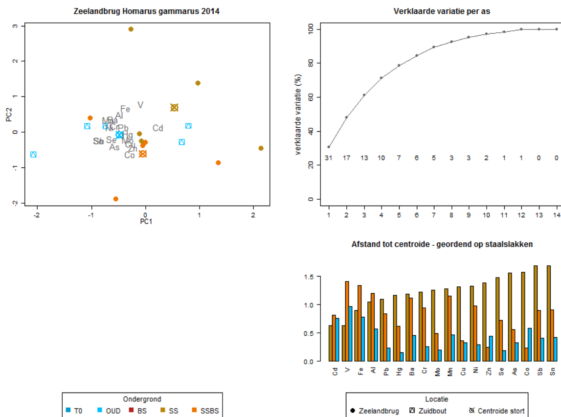
Figuur 34: Linksboven principal component (PCA) oriëntatie op z-gestransformeerde metaalgehalten in Homarus gammarus weefsel bemonsterd in 2014 bij de Zeelandbrug met scaling factor 2 (nadruk op metaalverschillen). De ondergrondtypen worden als volgt aangeduid: T0 = meting voor bestorting, OUD= oude ondergrond op referentielocatie, BS = breukstenen, SS = staalslakken, SSBS = staan onder invloed van staalslakken en breukstenen. Metalen met meer dan 75% meetwaarden onder de detectielimiet zijn buitenbeschouwing gelaten. Rechtsboven de verklaarde variatie per PCA-as. Linksonder de afstand van de metalen tot de centroïde van de verschillende ondergronden, geordend op toenemende afstand centroïde breukstenen, rechtsonder geordend op toenemende afstand centroïde staalslakken; hoe korter de afstand hoe relatief hoger het metaalgehalte.
