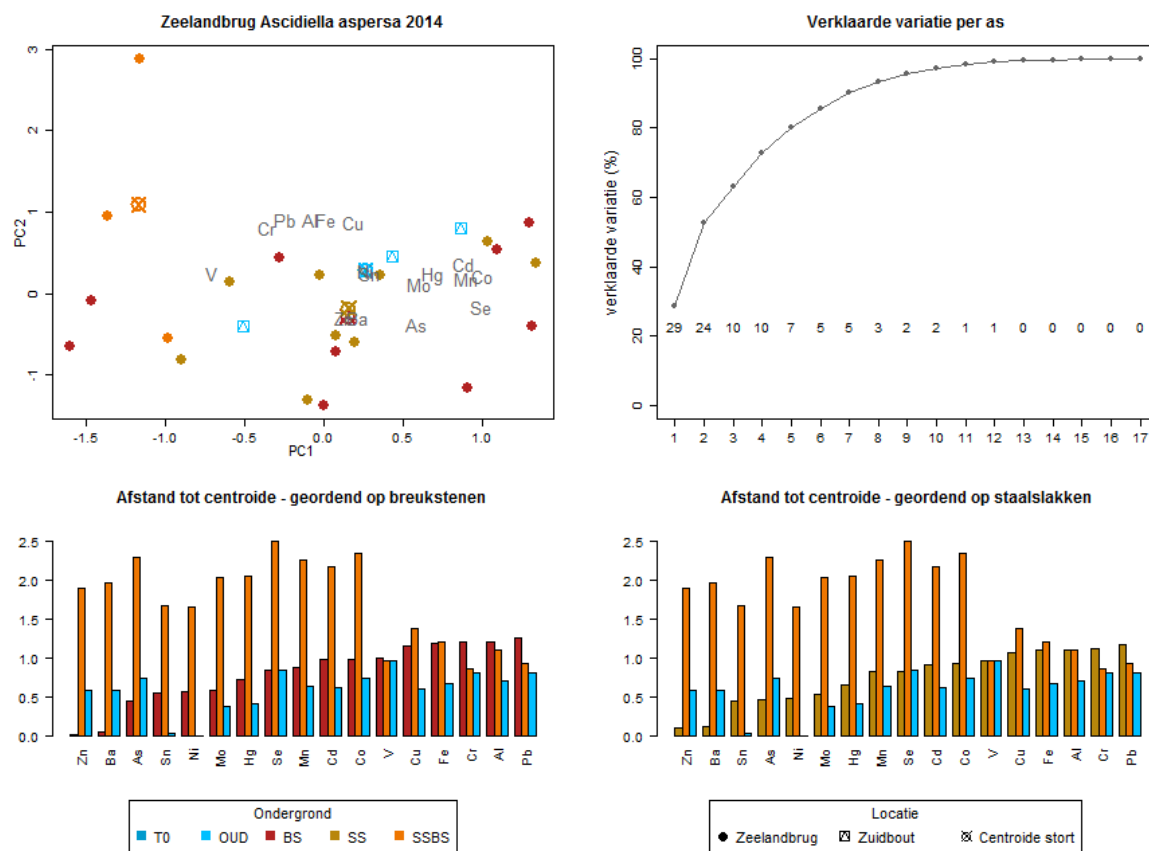
Figuur 26: Linksonder principal component (PCA) oriëntatie op z-gestransformeerde metaalgehalten in Ascidella aspersa weefsel bemonsterd in 2014 bij de Zeelandbrug met scaling factor 2 (nadruk op metaalverschillen). De ondergrondtypen worden als volgt aangeduid: T0 = meting voor bestorting, OUD= oude ondergrond op referentielocatie, BS = breukstenen, SS = staalslakken, SSBS = staan onder invloed van staalslakken en breukstenen. Metalen met meer dan 75% meetwaarden onder de detectielimiet zijn buitenbeschouwing gelaten. Rechtsboven de verklaarde variatie per PCA-as. Linksonder de afstand van de metalen tot de centroide van de verschillende ondergronden, geordend op toenemende afstand centroide breukstenen, rechtsonder geordend op toenemende afstand centroide staalslakken; hoe korter de afstand hoe relatief hoger het metaalgehalte.
