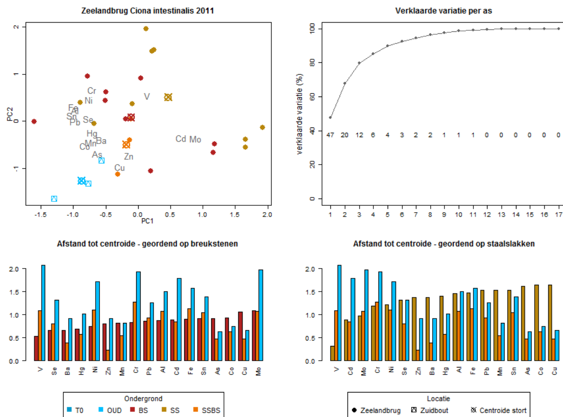
Figuur 22: Linksonder principal component (PCA) oriëntatie op z-gestransformeerde metaalgehalten in Ciona intestinalis weefsel bemonsterd in 2011 bij de Zeelandbrug met scaling factor 2 (nadruk op metaalverschillen). De ondergrondtypen worden als volgt aangeduid: T0 = meting voor bestorting, OUD= oude ondergrond op referentielocatie, BS = breukstenen, SS = staalslakken, SSBS = staan onder invloed van staalslakken en breukstenen. Metalen met meer dan 75% meetwaarden onder de detectielimiet zijn buitenbeschouwing gelaten. Rechtsboven de verklaarde variatie per PCA-as. Linksonder de afstand van de metalen tot de centroide van de verschillende ondergronden, geordend op toenemende afstand centroide breukstenen, rechtsonder geordend op toenemende afstand centroide staalslakken; hoe korter de afstand hoe relatief hoger het metaalgehalte.
