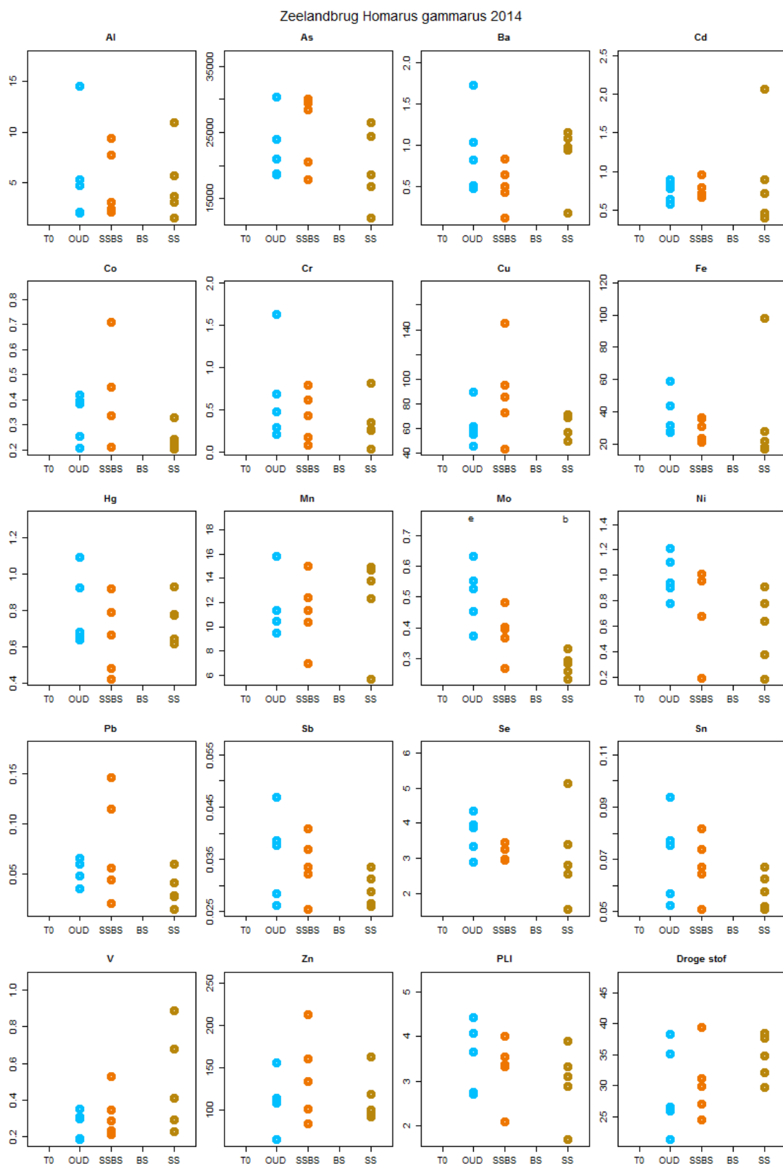
Figuur 35: Metaalgehalten, PLI en drogestof in Homarus gammarus bemonsterd op verschillende ondergronden bij de Zeelandbrug in 2014. De ondergrondtypen worden als volgt aangeduid: T0 = meting voor bestorting, OUD= oude ondergrond op referentielocatie, BS = breukstenen, SS = staalslakken, SSBS = staan onder invloed van staalslakken en breukstenen. Metaalgehalten die onder de detectielimiet liggen worden weergegeven met zwarte stippen. De lettercode geeft significante verschillen weer (ANOVA, Tukey Posthoc).
