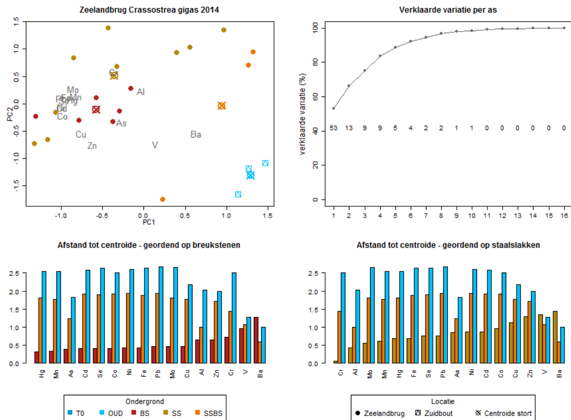
Figuur 28: Linksonder principal component (PCA) oriëntatie op z-gestransformeerde metaalgehalte in Crassostrea gigas weefsel bemonsterd in 2014 bij de Zeelandbrug met scaling factor 2 (nadruk op metaalverschillen). De ondergrondtypen worden als volgt aangeduid: T0 = meting voor bestorting, OUD= oude ondergrond op referentielocatie, BS = breukstenen, SS = staalslakken, SSBS = staan onder invloed van staalslakken en breukstenen. Metalen met meer dan 75% meetwaarden onder de detectielimiet zijn buitenbeschouwing gelaten. Rechtsboven de verklaarde variatie per PCA-as. Linksonder de afstand van de metalen tot de centroide van de verschillende ondergronden, geordend op toenemende afstand centroide breukstenen, rechtsonder geordend op toenemende afstand centroide staalslakken; hoe korter de afstand hoe relatief hoger het metaalgehalte.
