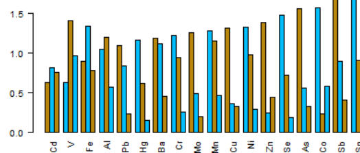
Afstand tot centroe - geordend op staalslakken
