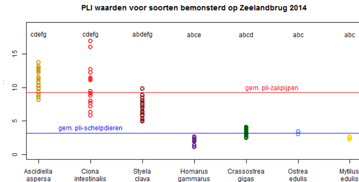
Figuur 3: PLI-waarden voor 3 zakpijpsorten, kreeft, 2 oestersorten en mossel bemonsterd op de Zeelandbrug in 2014. Significante verschillen worden aangegeven met lettercode.
