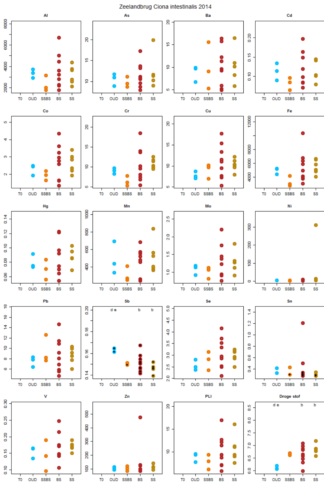
Figuur 25: Metaalgehalten, PLI en drogestof in Ciona intestinalis bemonsterd op verschillende ondergronden bij Zeelandbrug in 2014. De ondergrondtypen worden als volgt aangeduid: T0 = meting voor bestorting, OUD = oude ondergrond op referentielocatie, BS = breukstenen, SS = staalslakken, SSBS = staan onder invloed van staalslakken en breukstenen. Metaalgehalten die onder de detectielimiet liggen worden weergegeven met zwarte stippen. De lettercode geeft significante verschillen weer (ANOVA, Tukey Posthoc).
