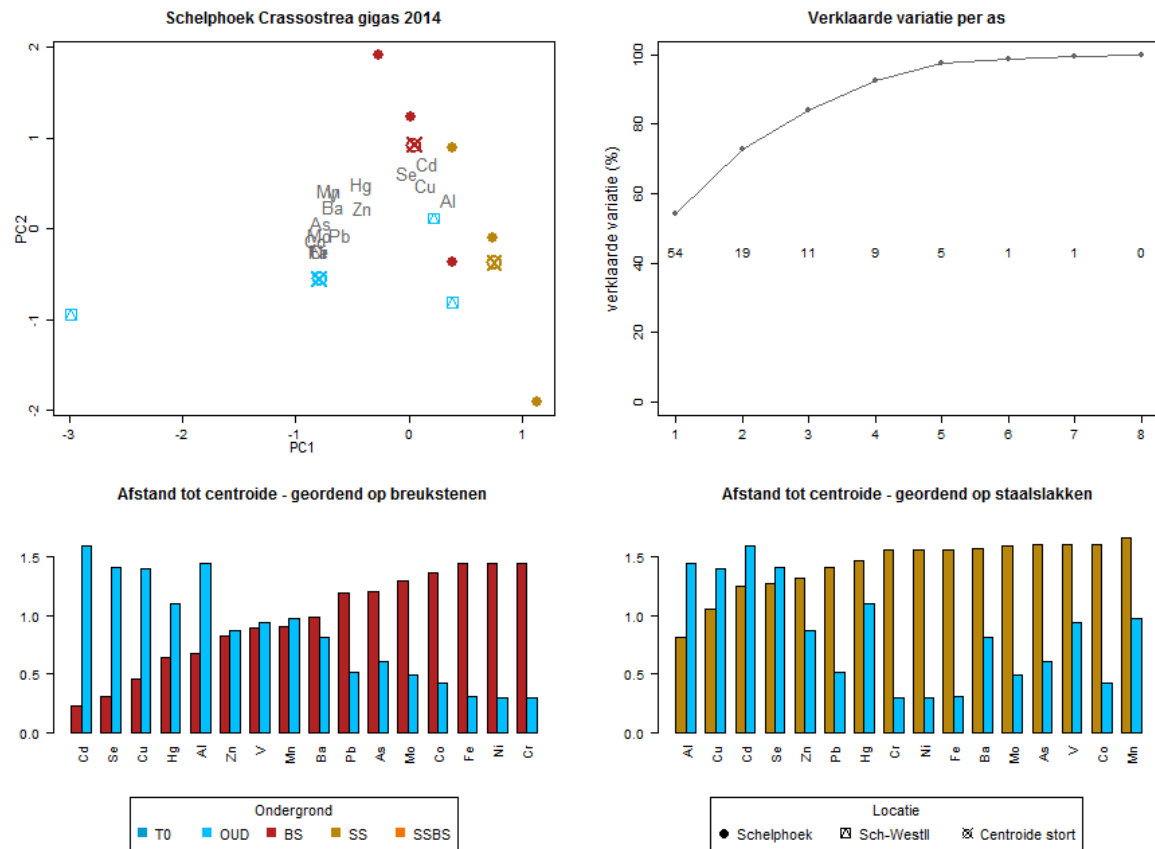
Figuur 30: Linksonder principal component (PCA) oriëntatie op z-gestransformeerde metaalgehalten in Crassostrea gigas weefsel bemonsterd in 2014 bij Schelphoek met scaling factor 2 (nadruk op metaalverschillen). De ondergrondtypen worden als volgt aangeduid: T0 = meting voor bestorting, OUD= oude ondergrond op referentielocatie, BS = breukstenen, SS = staalslakken, SSBS = staan onder invloed van staalslakken en breukstenen. Metalen met meer dan 75% meetwaarden onder de detectielimiet zijn buitenbeschouwing gelaten. Rechtsboven de verklaarde variatie per PCA-as. Linksonder de afstand van de metalen tot de centroide van de verschillende ondergronden, geordend op toenemende afstand centroide breukstenen, rechtsonder geordend op toenemende afstand centroide staalslakken; hoe korter de afstand hoe relatief hoger het metaalgehalte.
