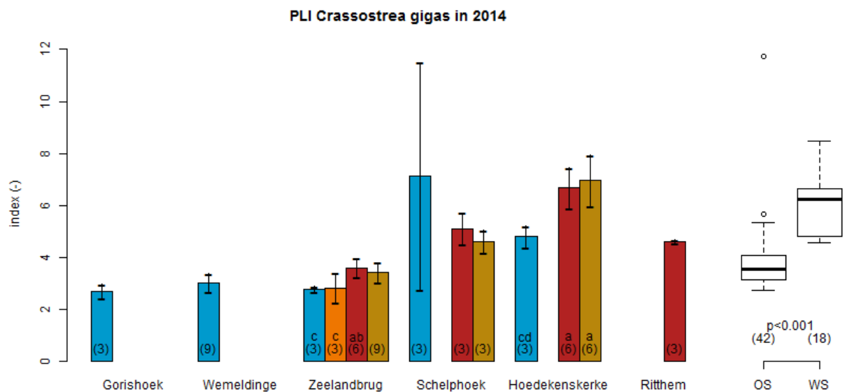
Figuur 5: Links gemiddelde ( \pm SD) Pollution Load Index (PLI) voor Japanse oesters verzameld op verschillende ondergronden en locaties in 2014. Blauwe bars zijn referentie/T0 metingen, oranje staalslakken + breukstenen, rood breukstenen en geel staalslakken. Bemonsteringslocaties in de Oosterschelde: Gorishoek, Wemeldinge, Zeelandbrug, Schelphoek, en in de Westerschelde: Hoedekenskerke en Ritthem. Rechts gehalten uitgedrukt per bekken. Significant verschillende PLI waarden tussen ondergrondtype worden aangegeven met letters binnen locaties (ANOVA, p < 0.05 ; Tukey Post hoc). Hierbij zijn de volgende referentie en stortlocaties gekoppeld: Zuidbout aan Zeelandbrug, Schelphoek-west II aan Schelphoek, Kappellebank aan Hoedekenskerke, en voor Ritthem was geen referentielocatie beschikbaar in 2014. De PLI uitschieter bij Schelphoek wordt veroorzaakt door hoge kobalt (Co), chroom (Cr), molybdeen (Mo) en nikkel (Ni) gehalten, zie Bijlage D.
