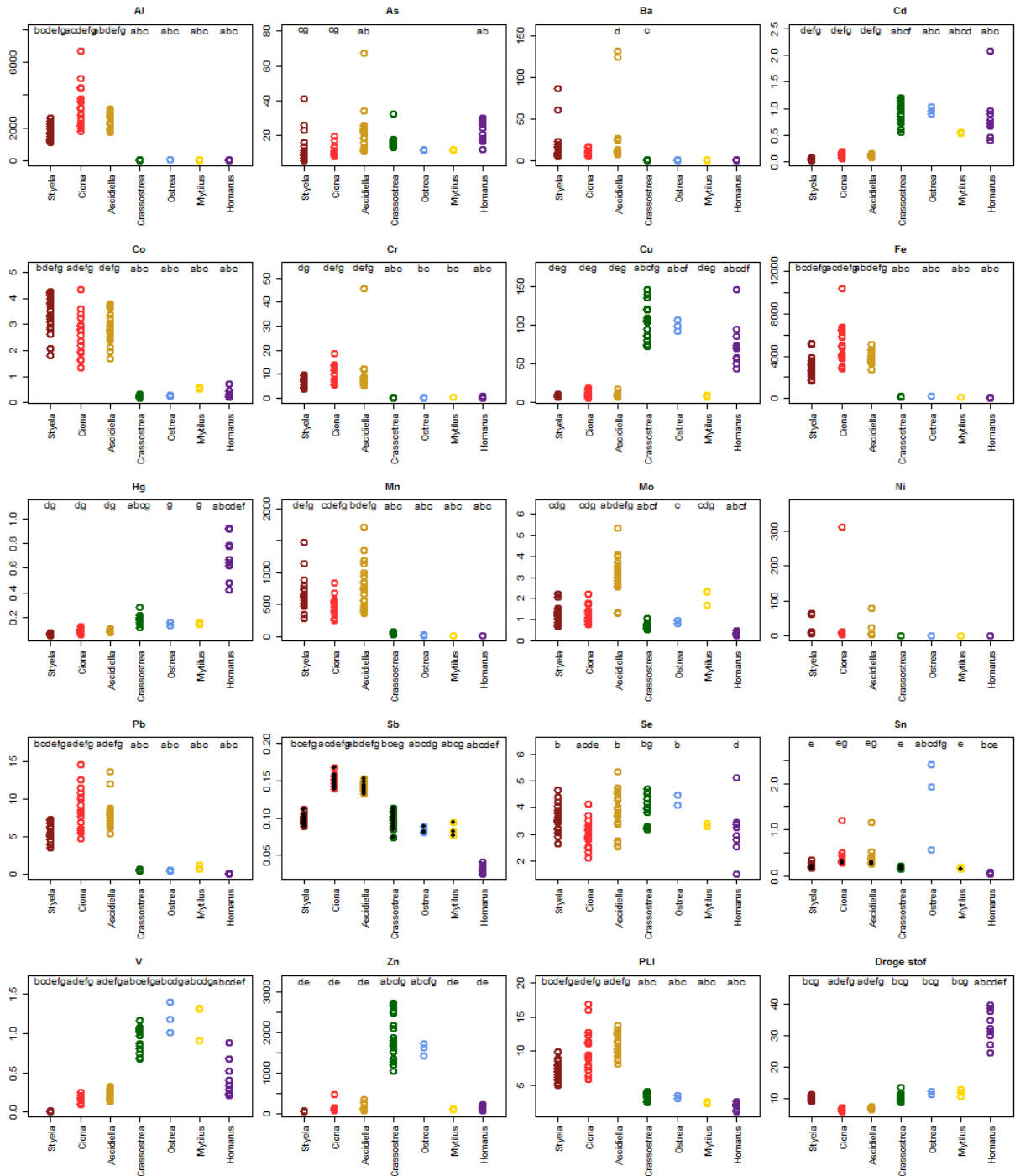
Figuur 13: Metaalgehalten, PLI en droge stof voor de zakpijpsorten Styela clava (a), Ciona intestinalis (b) en Ascidiella aspersa (c), de oesters Crassostrea gigas (d) en Ostrea edulis (e), de mossel Mytilus edulis (f) en de kreeft Homanus gammarus (g) bemonsterd op de Zeelandbrug in 2014. Metaalgehalten die onder de detectielimiet liggen worden weergegeven met zwarte stippen. De lettercode geeft significante verschillen weer (ANOVA, Tukey Post hoc).
