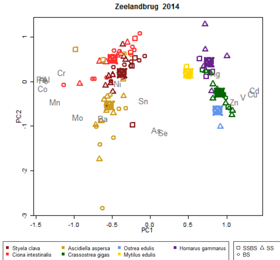
Figuur 2: Principal component (PCA) oriëntatie op z-gestransformeerde metaalgehalten in de zakpijpsorten Styela clava, Ciona intestinalis en Ascidiella aspersa, de oesters Crassostrea gigas en Ostrea edulis, de mossel Mytilus edulis en de kreeft Homarus gammarus bemonsterd op de Zeelandbrug in 2014. Scaling factor 2 (nadruk op metaalverschillen). Metalen met meer dan 75% meetwaarden onder de detectielimiet zijn buitenbeschouwing gelaten.
