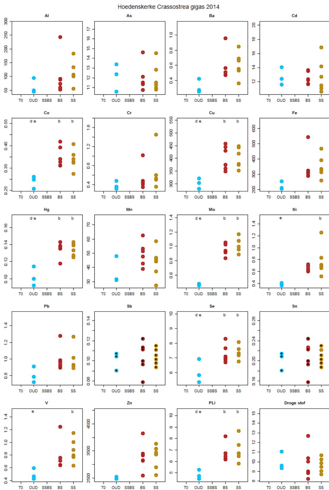
Figuur 33: Metaalgehalten, PLI en drogestof in Crassostrea gigas bemonsterd op verschillende ondergronden bij de Hoedekenskerke in 2014. De ondergrondtypen worden als volgt aangeduid: T0 = meting voor bestorting, OUD= oude ondergrond op referentielocatie, BS = breukstenen, SS = staalslakken, SSBS = staan onder invloed van staalslakken en breukstenen. Metaalgehalten die onder de detectielimiet liggen worden weergegeven met zwarte stippen. De lettercode geeft significante verschillen weer (ANOVA, Tukey Posthoc).
