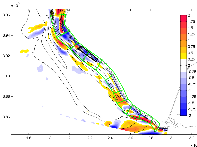
Figuur 3-10 Sedimentatie/erosie patronen (in meters) na 4 jaar voor suppletie 1 ( 2,5 \text{ Mm}^3 ). Rode tinten geven sedimentatie aan, blauwe tonen erosie.
