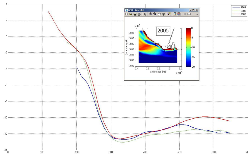
Figuur 2-13 Dwarsdoorsnedes van de drempel tussen Sardijngeul en Honte voor de jaren 1964, 2000 en 2005
