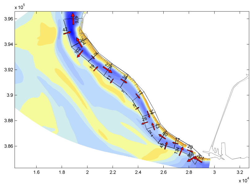
Figuur 3-26 Resttransporten ( \text{Mm}^3/\text{jaar} ) voor suppletie 3 ( 30 \text{ Mm}^3 ).
