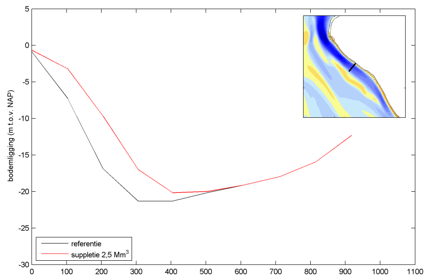
Figure 3-7 Dwarsdoorsnede van de suppletie 1 ( 2,5 \text{ Mm}^3 )
