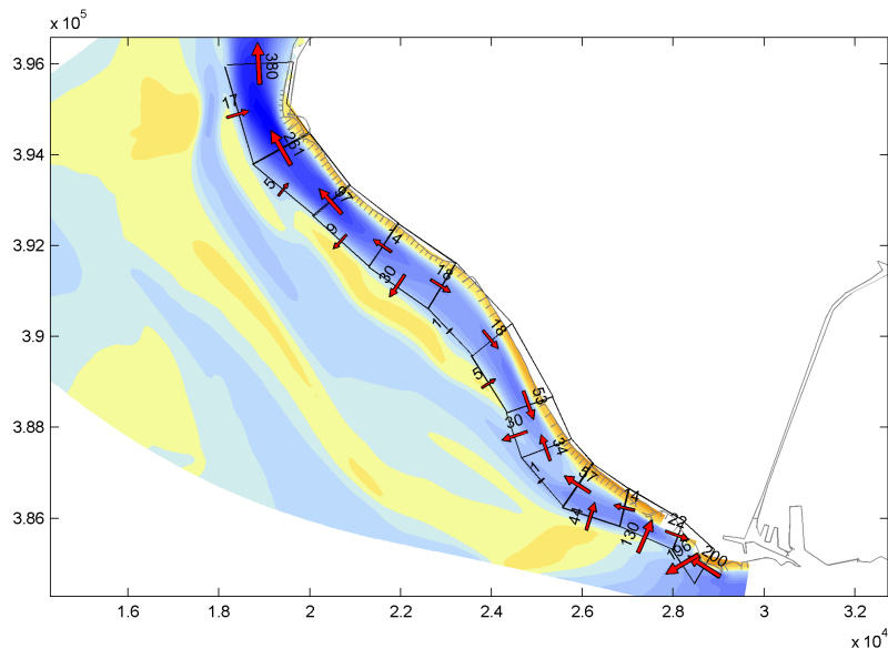
Figuur 3-12 Resttransporten ( \text{Mm}^3/\text{jaar} ) voor suppletie 1 ( 2,5 \text{ Mm}^3 ).
