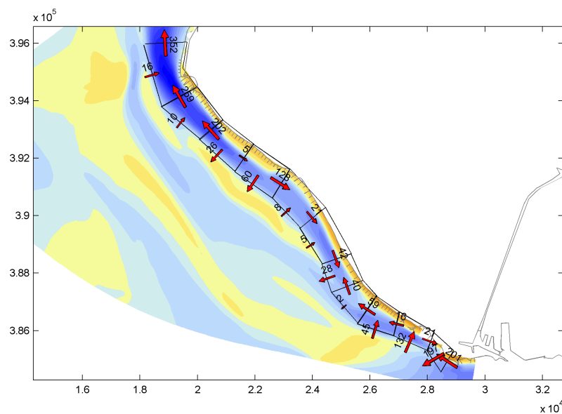
Figuur 3-18 Resttransporten ( \text{Mm}^3/\text{jaar} ) voor suppletie 2 ( 12 \text{ Mm}^3 ).
