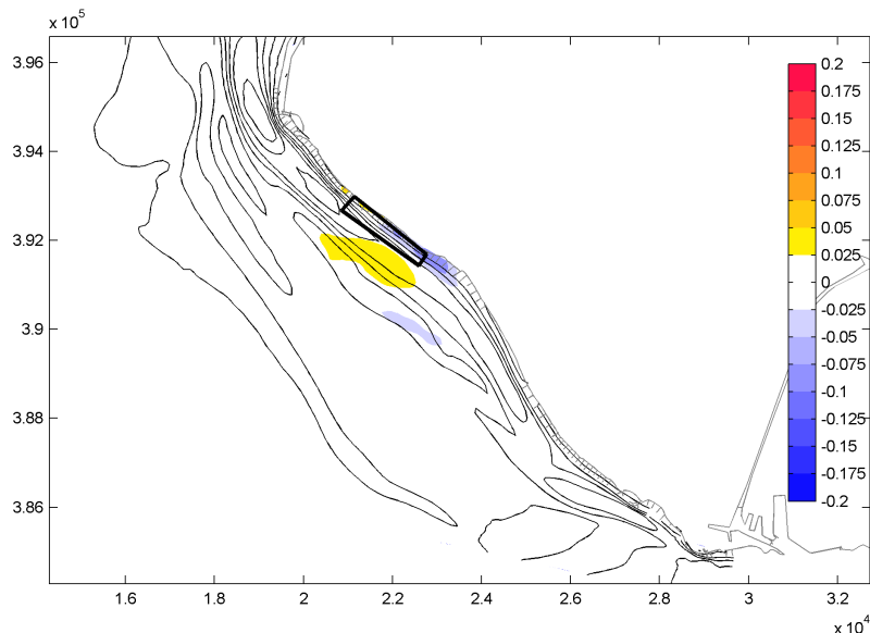
Figuur 3-9 Relatieve effecten van suppletie 1 (2,5 Mm³) op de stroomsnelheid bij maximum vloed. Rode tinten geven een toename aan, blauwe een afname.
