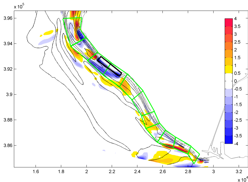
Figuur 3-16 Sedimentatie/erosie patronen (in meters) na 4 jaar voor suppletie 2 (12 Mm³). Rode tinten geven sedimentatie aan, blauwe tonen erosie.
