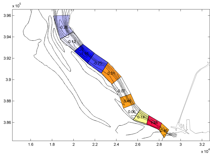
Figuur 3-17 Gemiddelde bodemveranderingen (in meters) na 4 jaar voor suppletie 2 (12 Mm 3 ). Rode tinten geven sedimentatie aan, blauwe tonen erosie.
