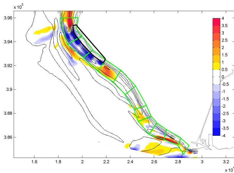
Figuur 3-24 Sedimentatie/erosie patronen (in meters) na 4 jaar voor suppletie 3 (30 Mm³). Rode tinten geven sedimentatie aan, blauwe tonen erosie.
