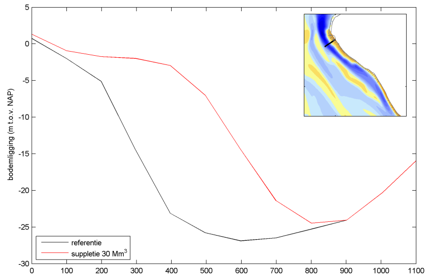
Figure 3-21 Dwarsdoorsnede van de suppletie 3 (30 Mm³)
