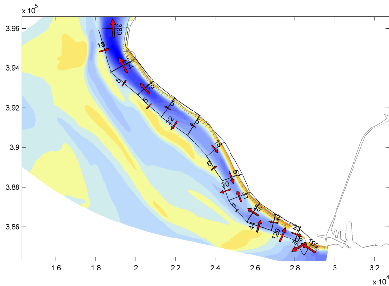
Figuur 3-6 Resttransporten ( \text{Mm}^3/\text{jaar} ) voor de referentiesituatie (geen suppletie).
