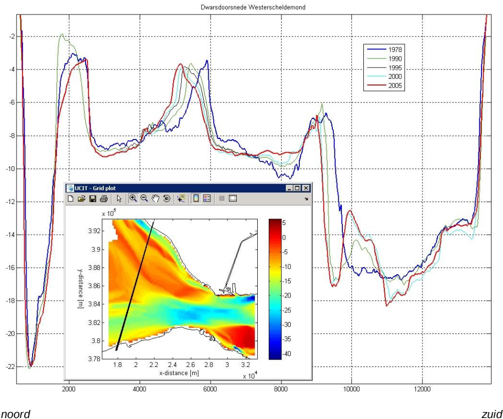
Figuur 2-7 Ontwikkelingen in een dwarsdoorsnede over de gehele monding over de periode 1978-2005. Links is Walcheren, rechts Zeeuws Vlaanderen, diepte in meters.
