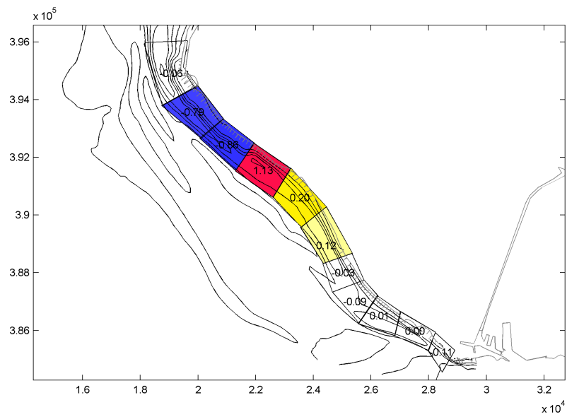
Figure 3-28 Relatieve gemiddelde bodemveranderingen (in meters) na 4 jaar t.g.v. suppletie 3 (30 Mm³). Rode tinten geven sedimentatie aan, blauwe tonen erosie.
