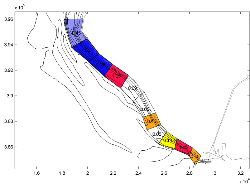
Figuur 3-25 Gemiddelde bodemveranderingen (in meters) na 4 jaar voor suppletie 3 (30 Mm³). Rode tinten geven sedimentatie aan, blauwe tonen erosie.
