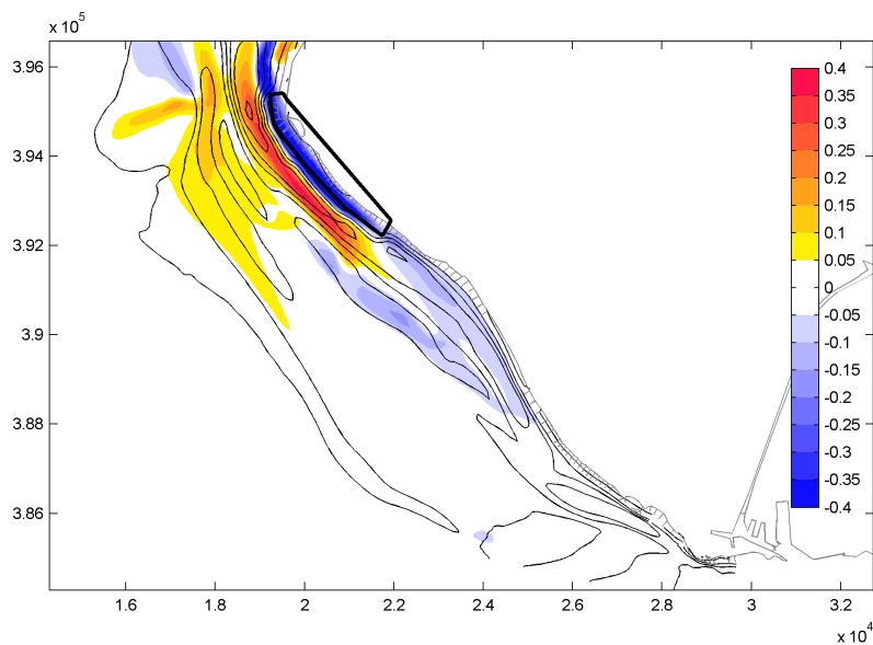
Figuur 3-22 Relatieve effecten van suppletie 3 (30 Mm³) op de stroomsnelheid bij maximum eb. Rode tinten geven een toename aan, blauwe een afname.
