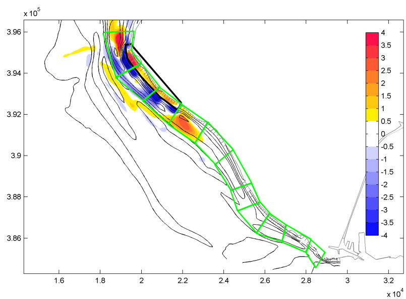
Figuur 3-27 Relatieve bodemveranderingen na 4 jaar ten gevolge van suppletie 3 ( 30 \text{ Mm}^3 ).
