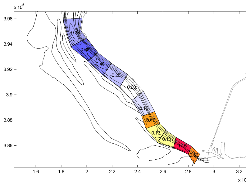
Figuur 3-11 Gemiddelde bodemveranderingen (in meters) na 4 jaar voor suppletie 1 ( 2,5 \text{ Mm}^3 ). Rode tinten geven sedimentatie aan, blauwe tonen erosie.
