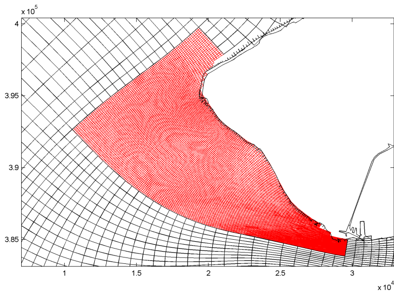
Figuur 3-2 Modelrooster (fijne domein)
