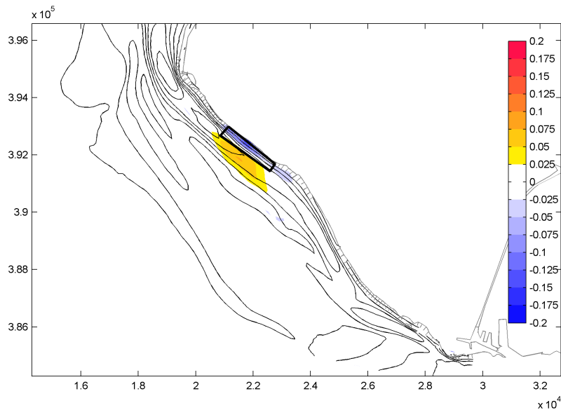
Figuur 3-8 Relatieve effecten van suppletie 1 (2,5 Mm³) op de stroomsnelheid bij maximum eb. Rode tinten geven een toename aan, blauwe een afname (+0,2 wil zeggen een toename met 20 %).
