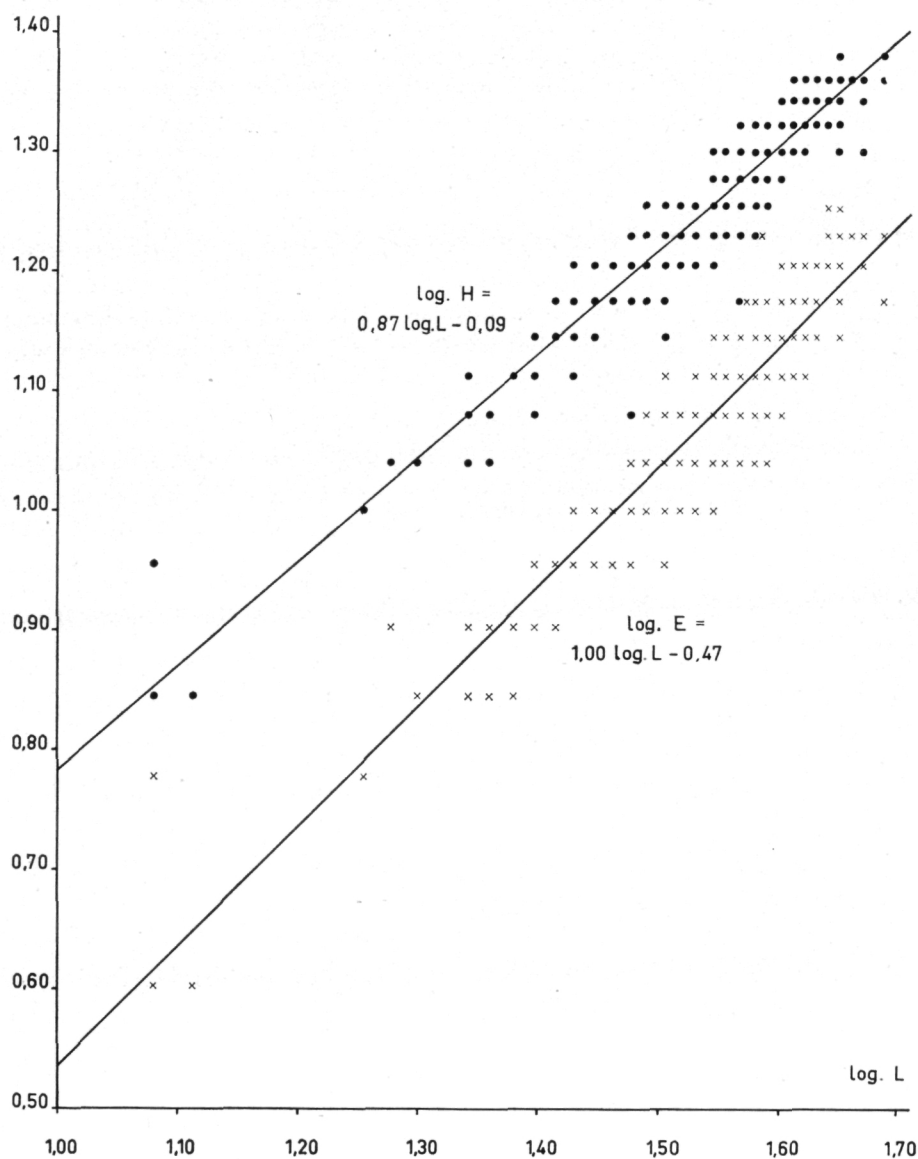
Fig. 6. — Moules recueillies sur la plaque en tufnol. Croissance relative de la hauteur (H) et de l'épaisseur (E) par rapport à la longueur (L). Coordonnées logarithmiques (4).
