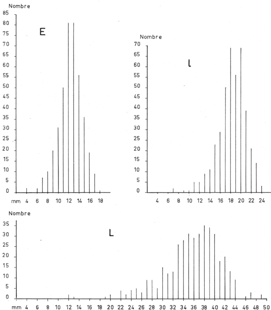
Fig. 4. — Mytilus edulis (L.) — Diagrammes des fréquences de la longueur (L), de la hauteur (l) et de l'épaisseur (E).
