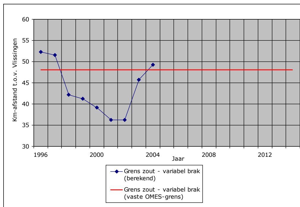
Figuur 5 De ligging van de berekende zoutgrens versus de vaste OMES-grens als afstand t.o.v. Vlissingen
